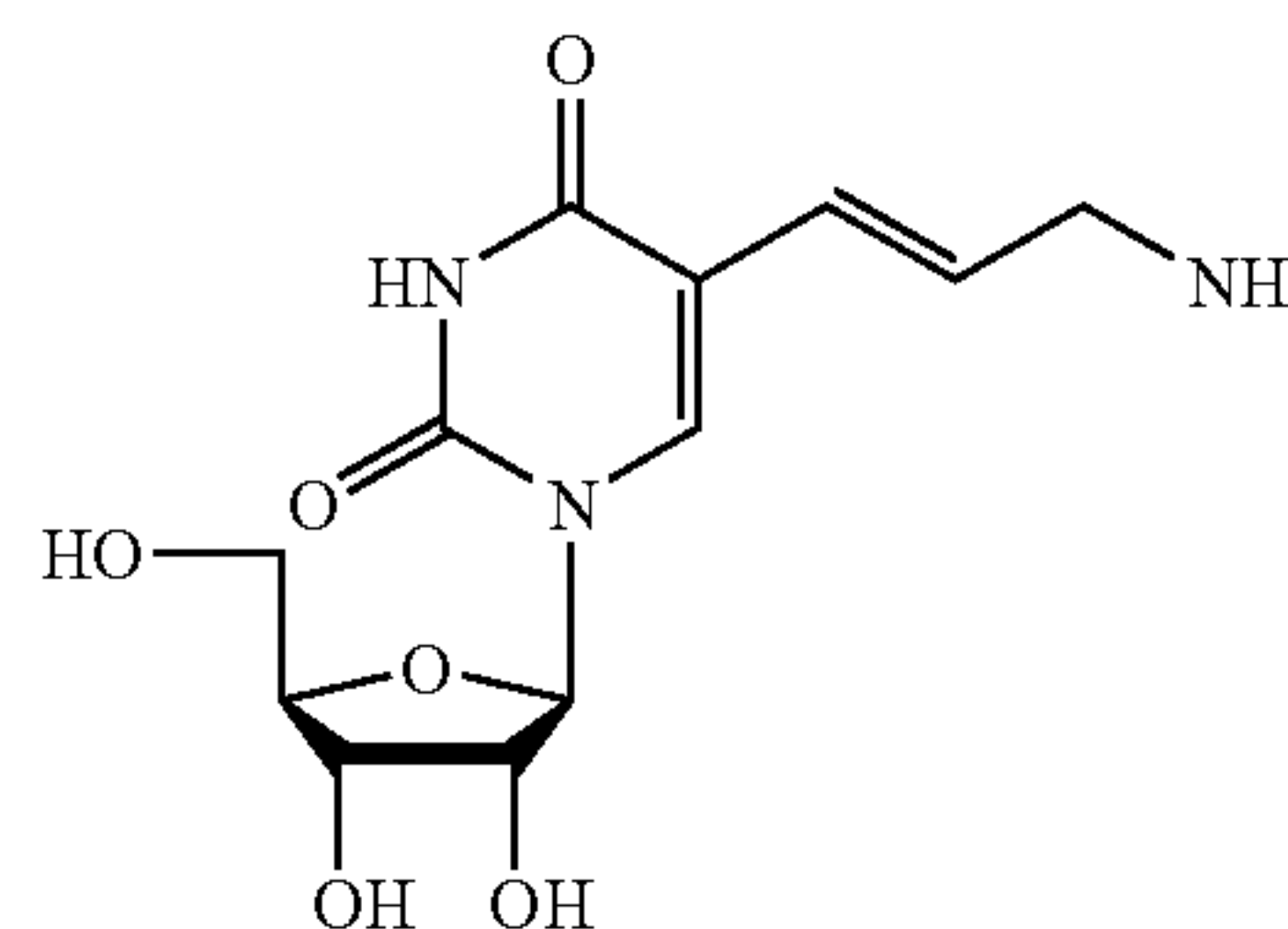
Allylamino-uridine
