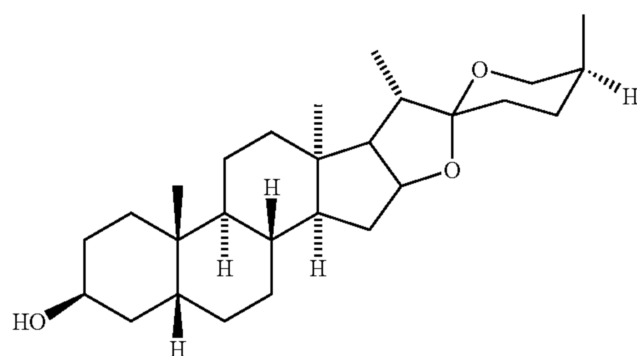
Sarsasapogenin
