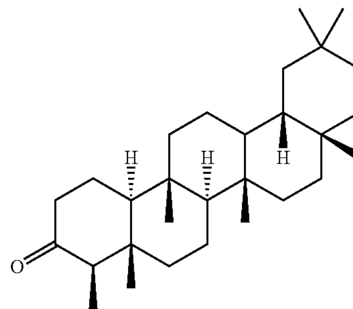
Friedelin
