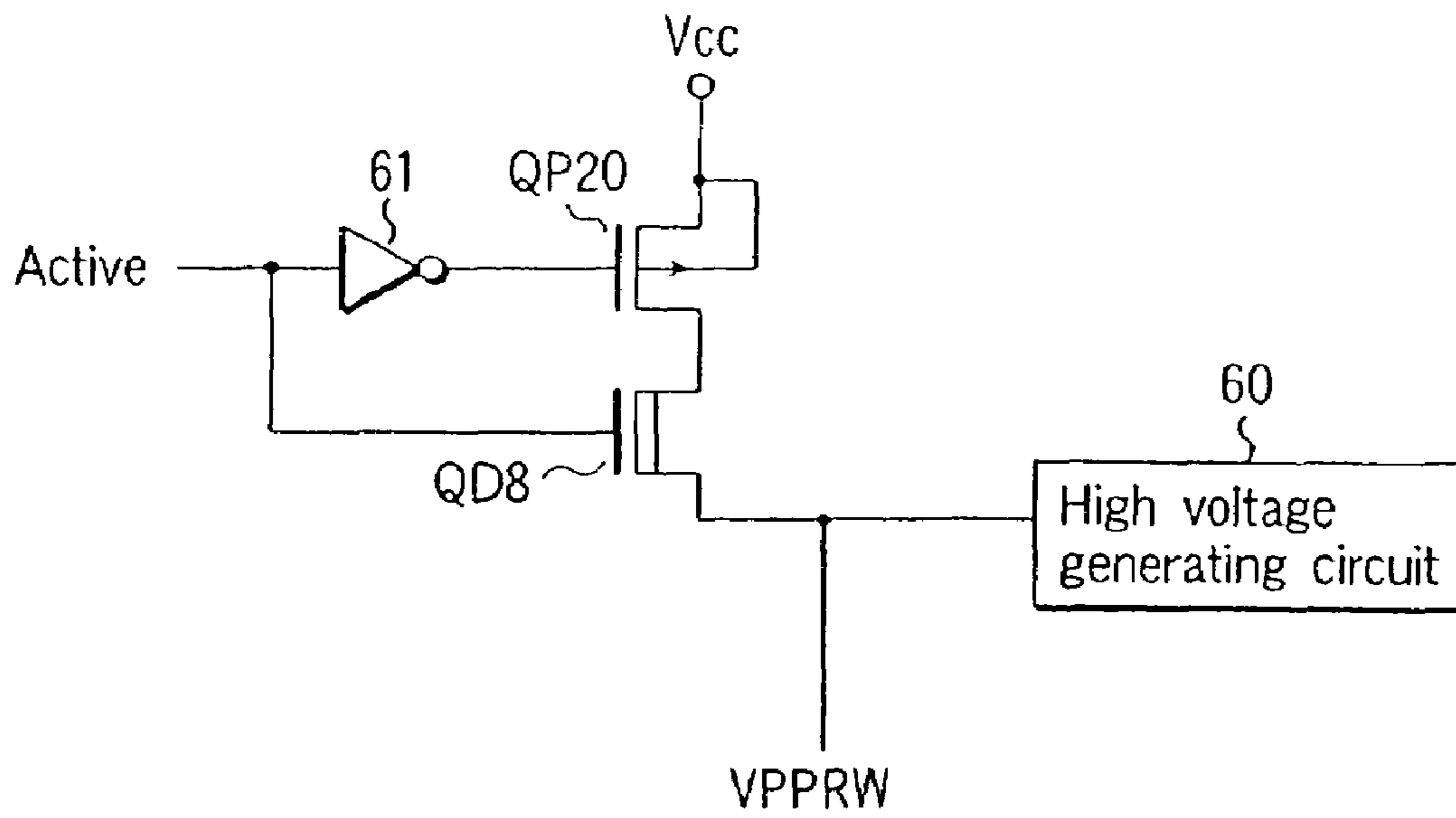
FIG. 34
