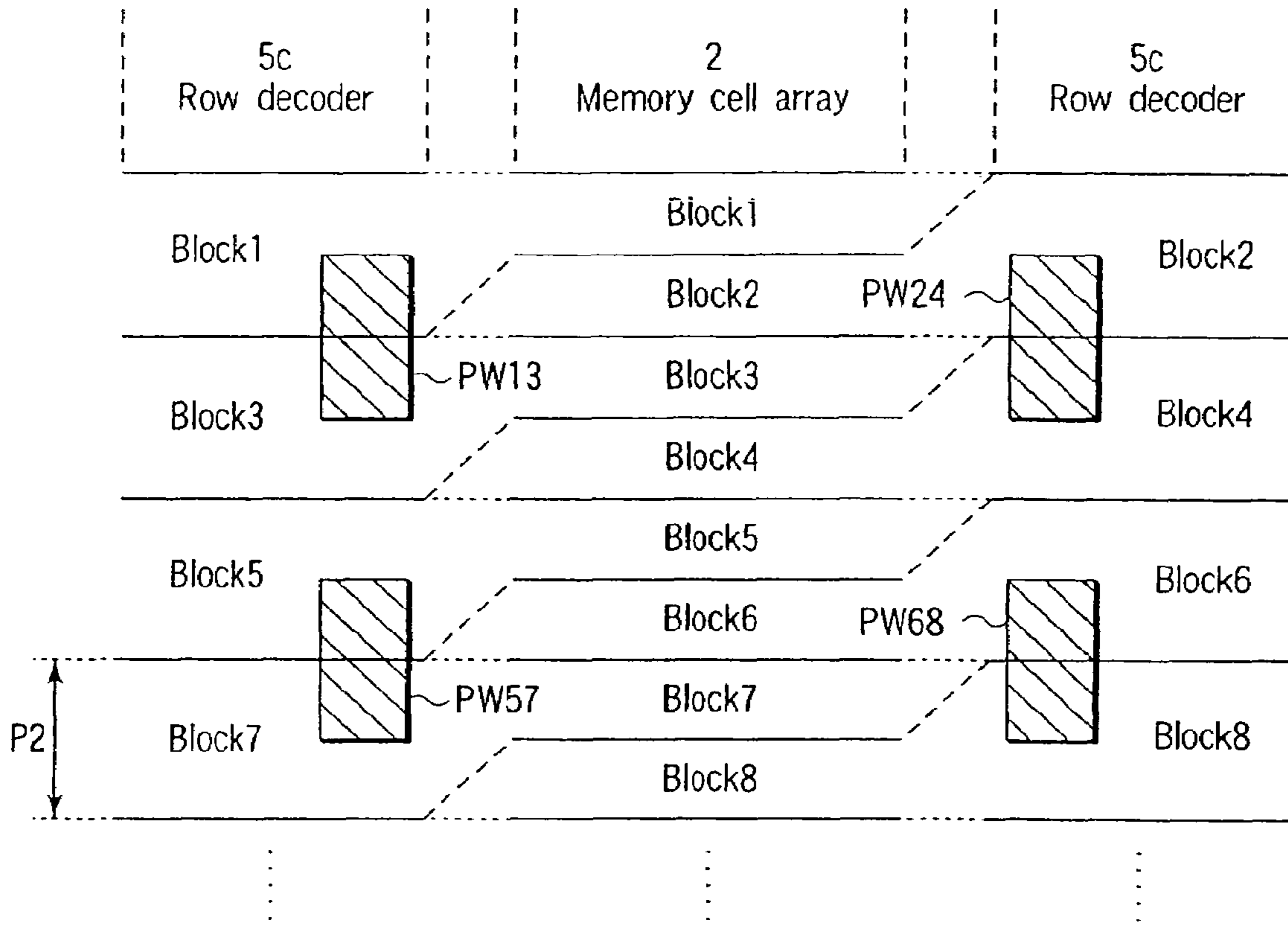
FIG. 28
