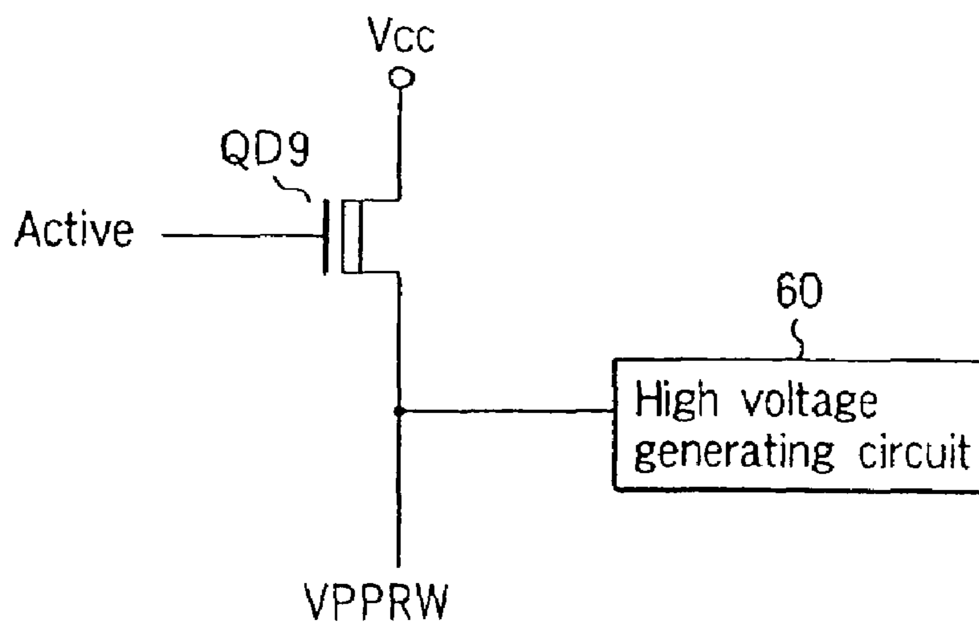
FIG. 35
