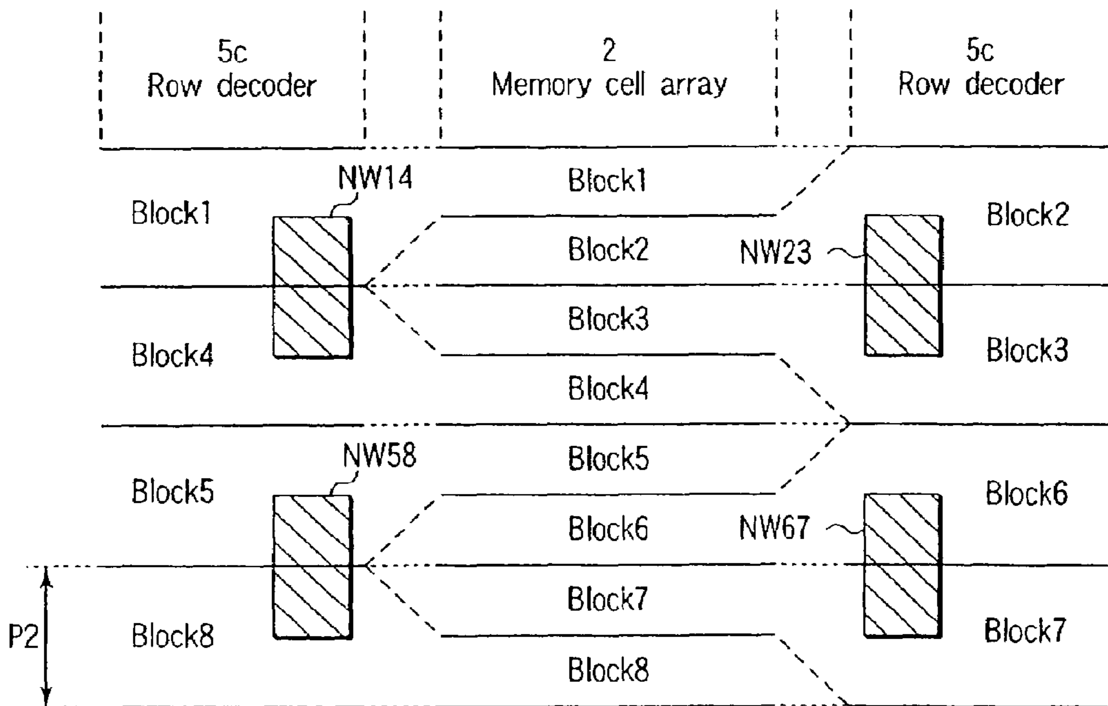
FIG. 27
