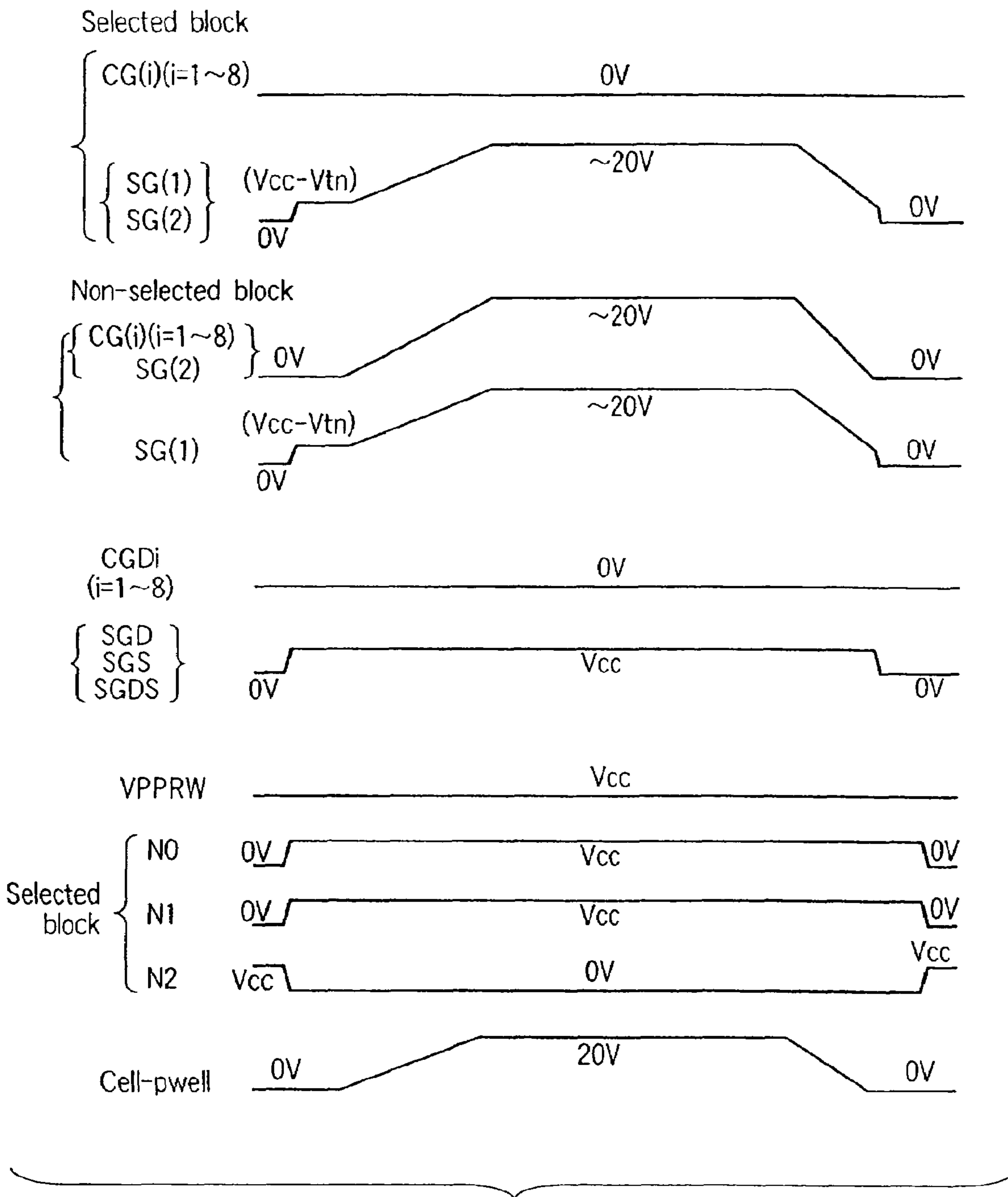
FIG. 10
