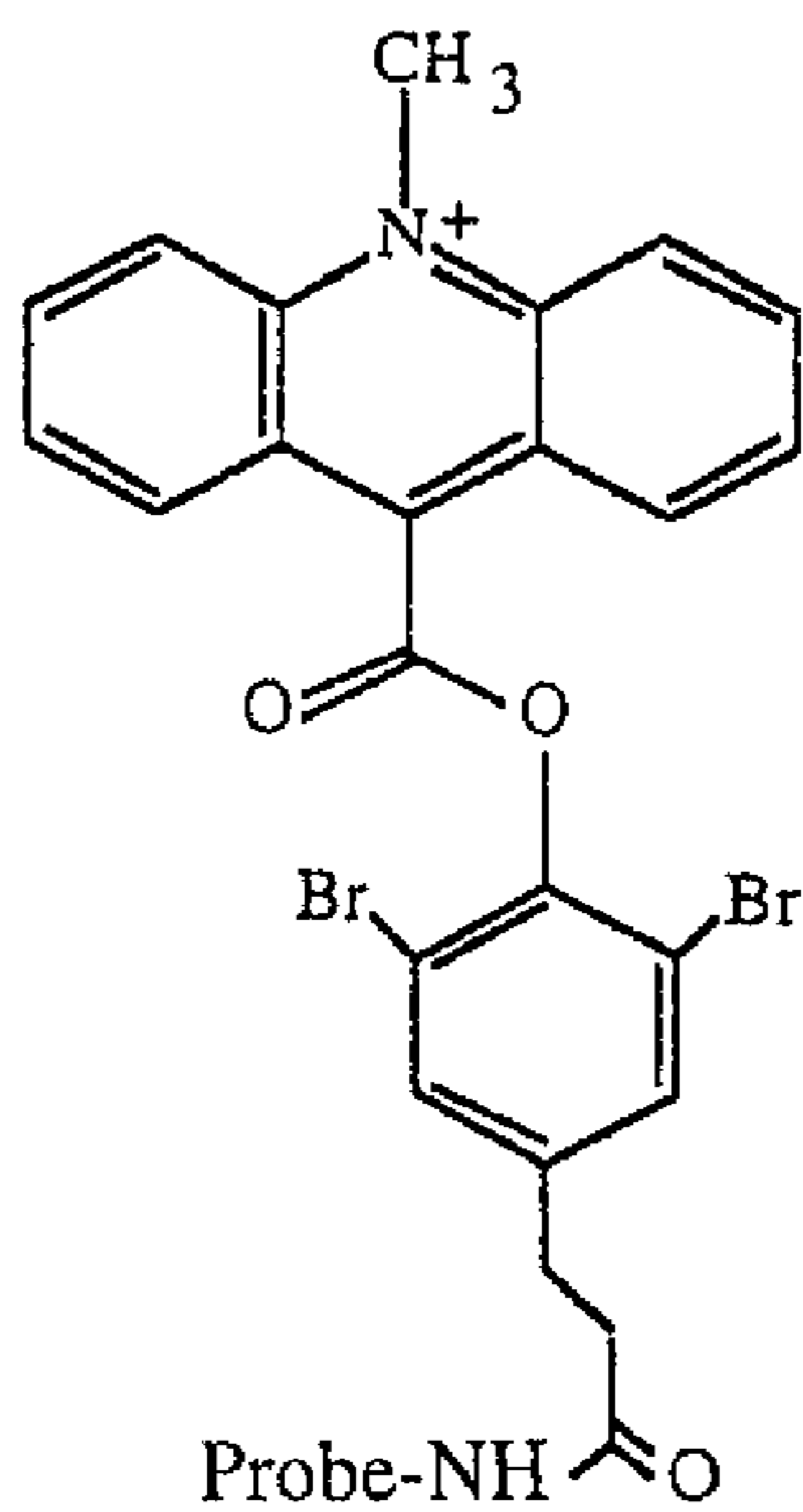
o -diBr-AE
