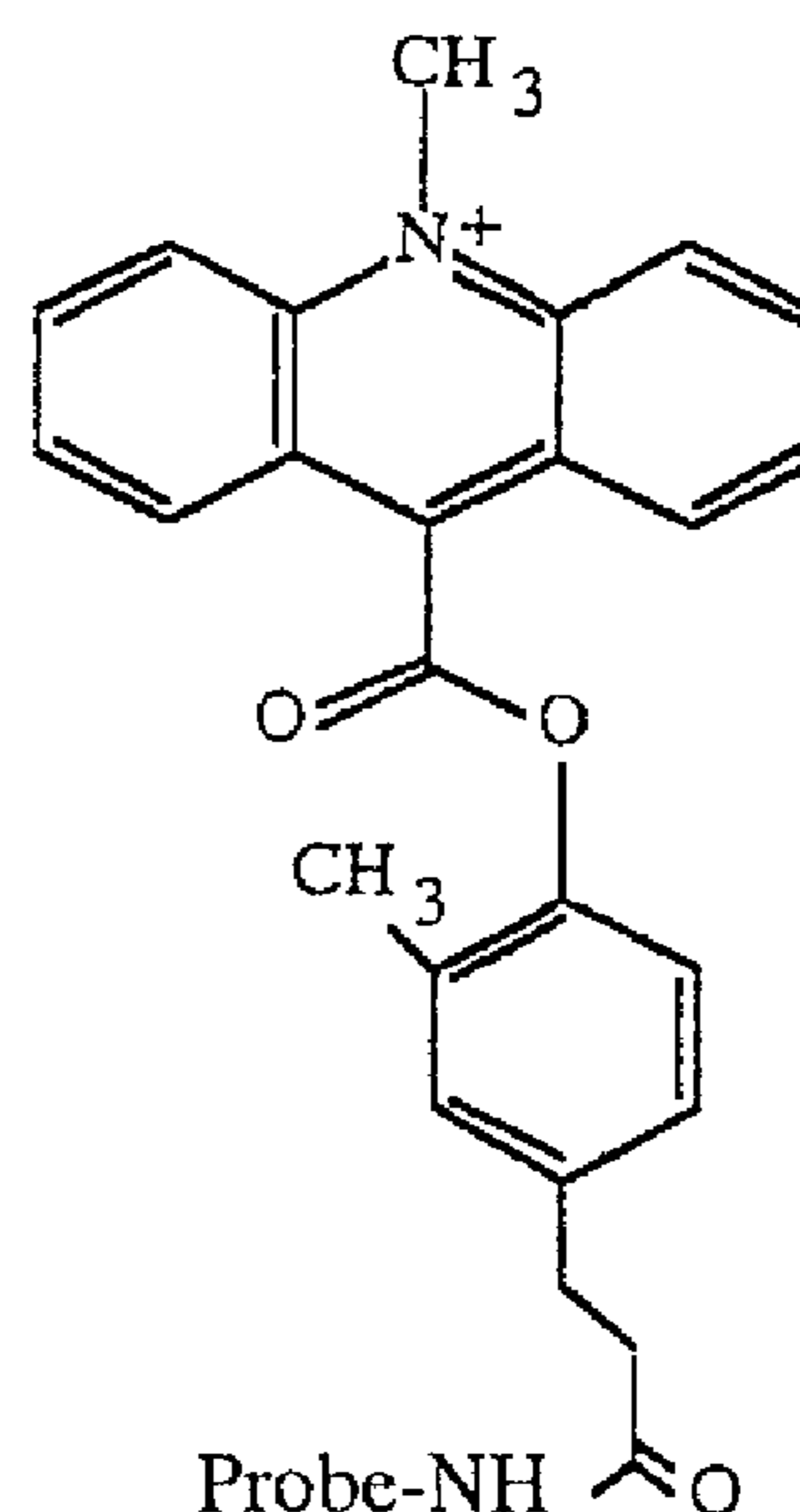
o -Me-AE
