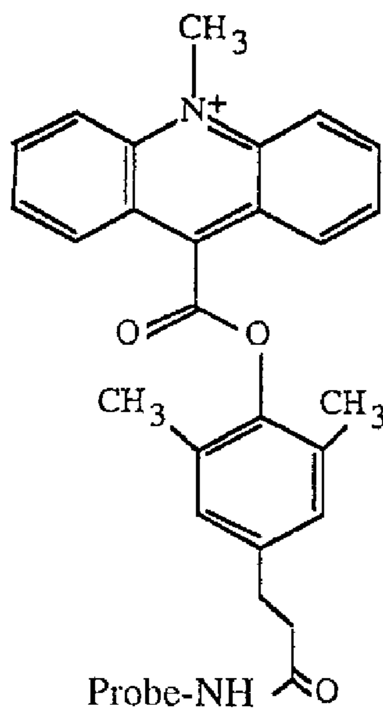
o -diMe-AE
