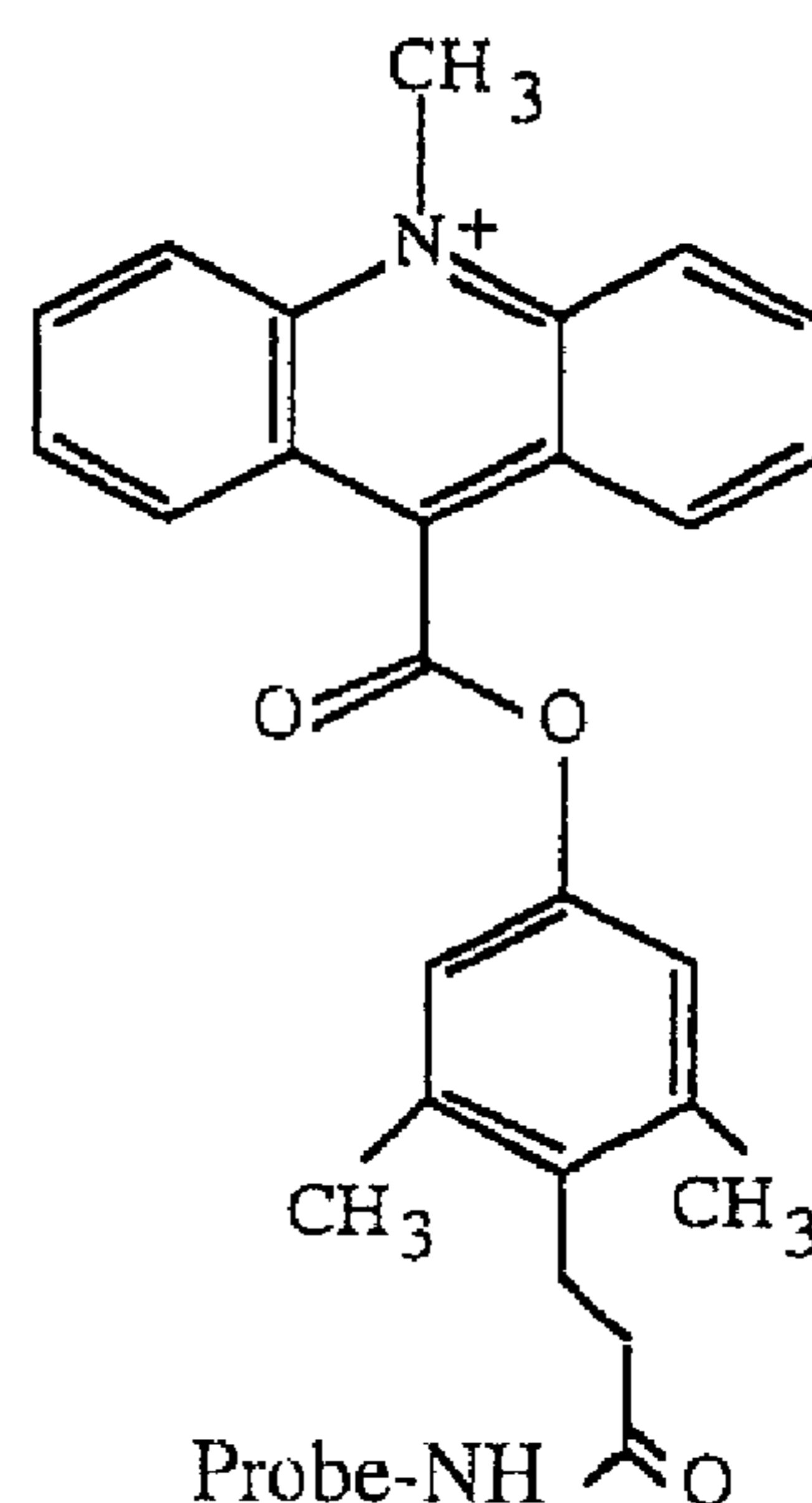
m -diMe-AE
