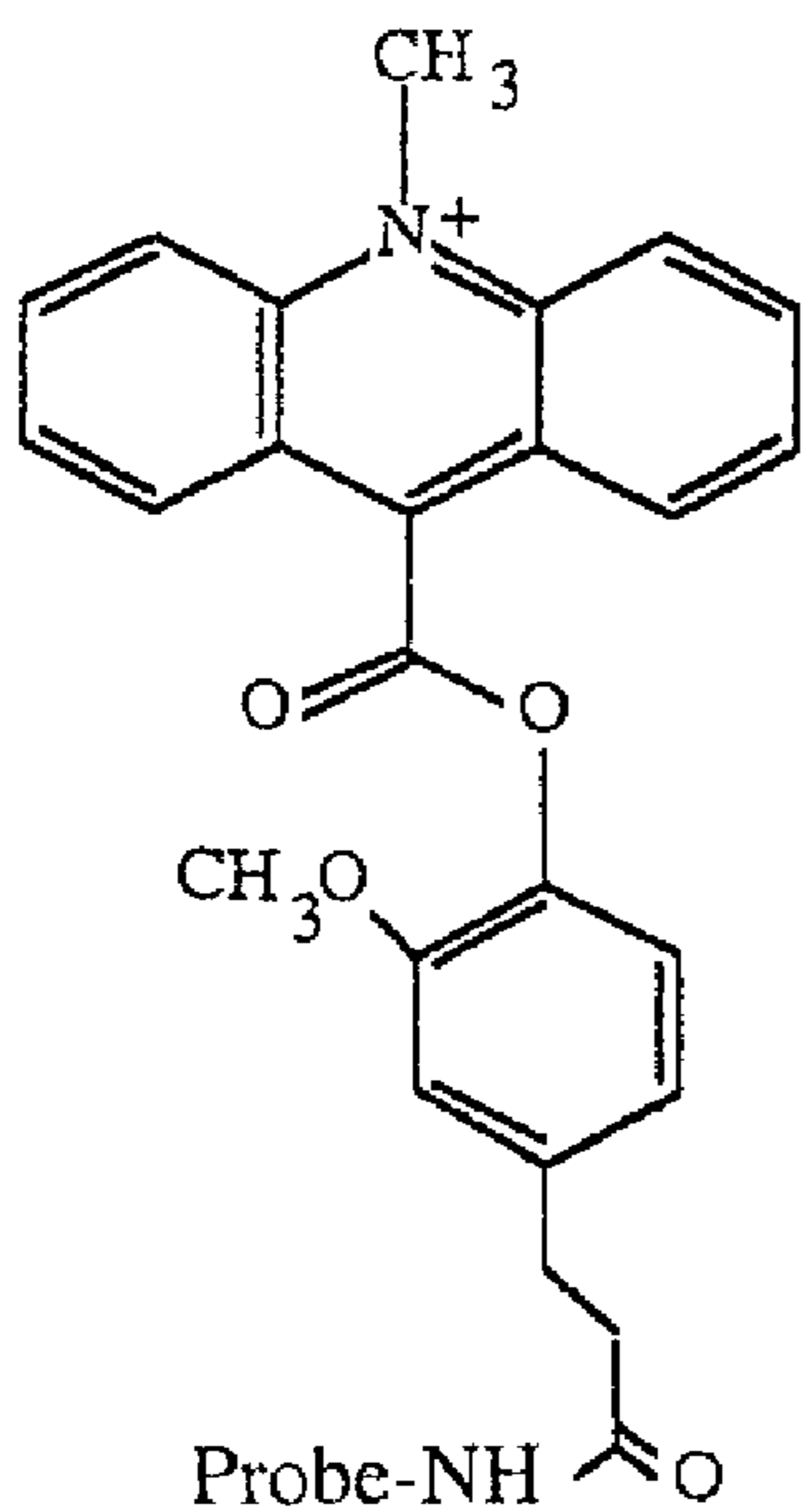
o -MeO-AE
