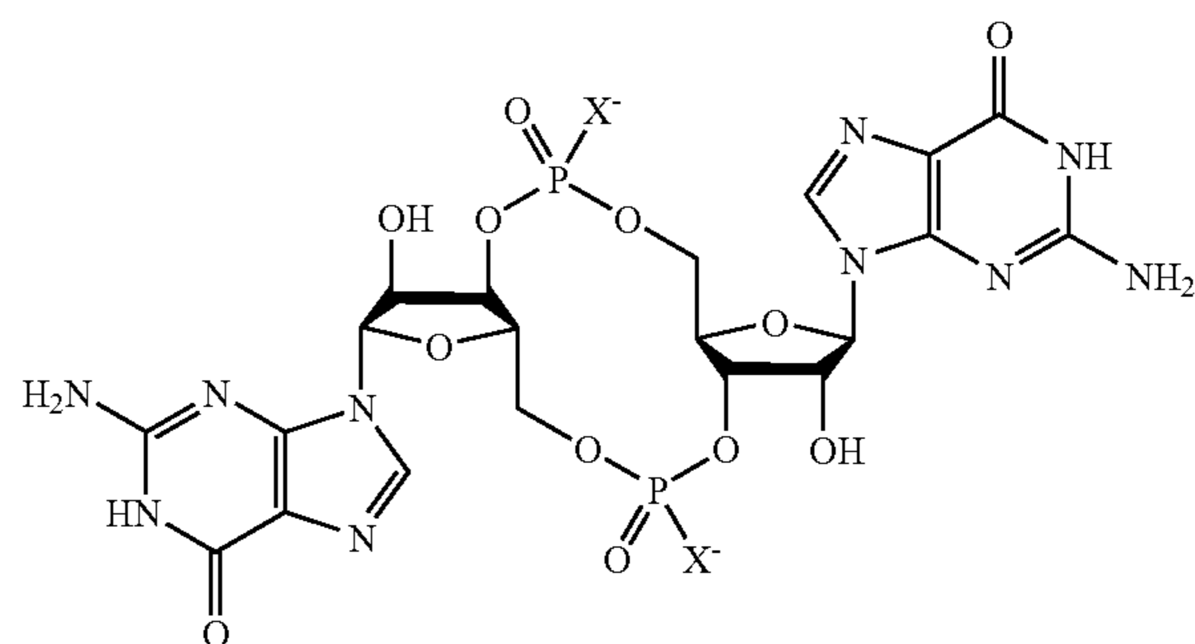
c-GpXGp X = S, Se stereochemically pure
