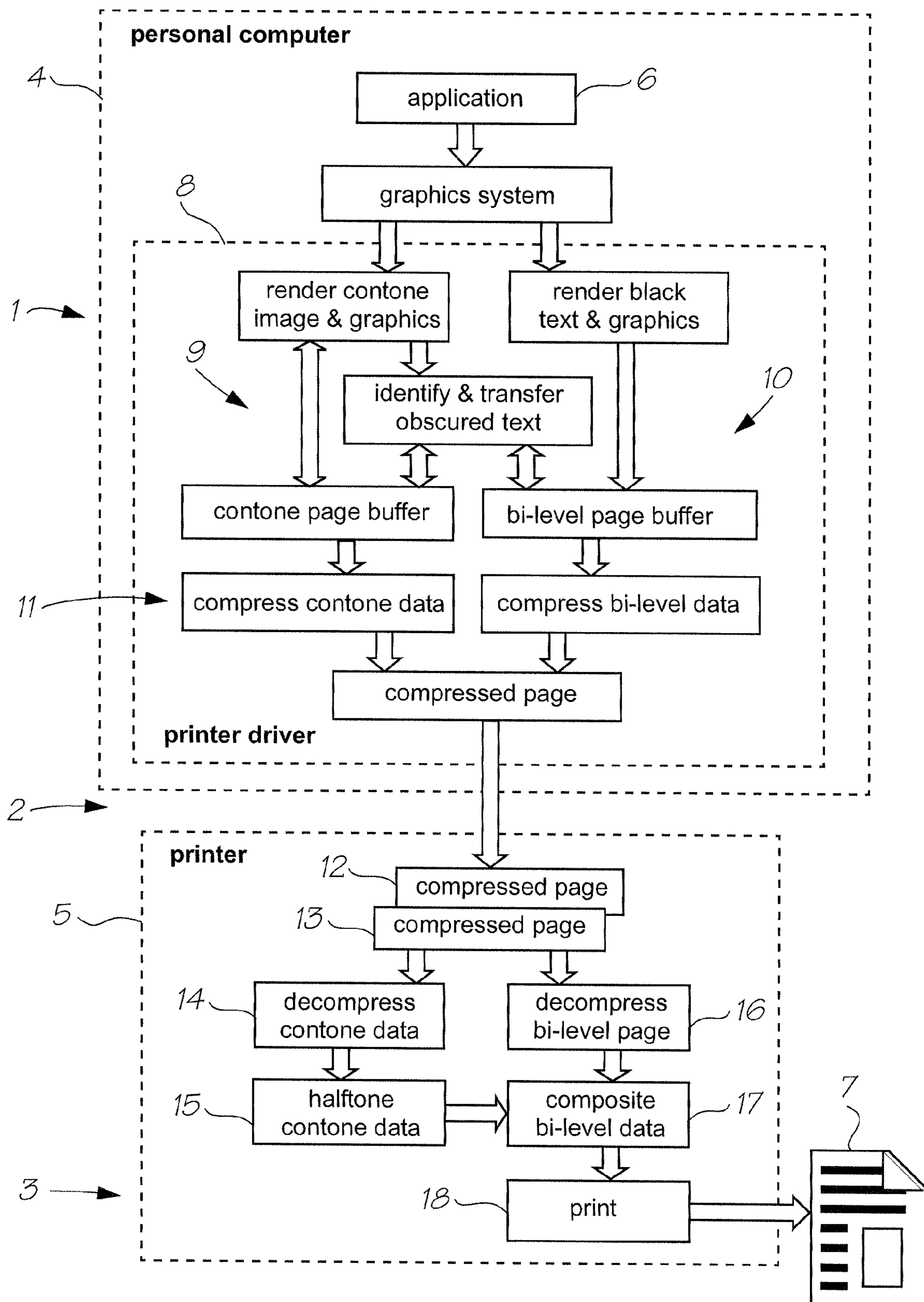
FIG. 2
