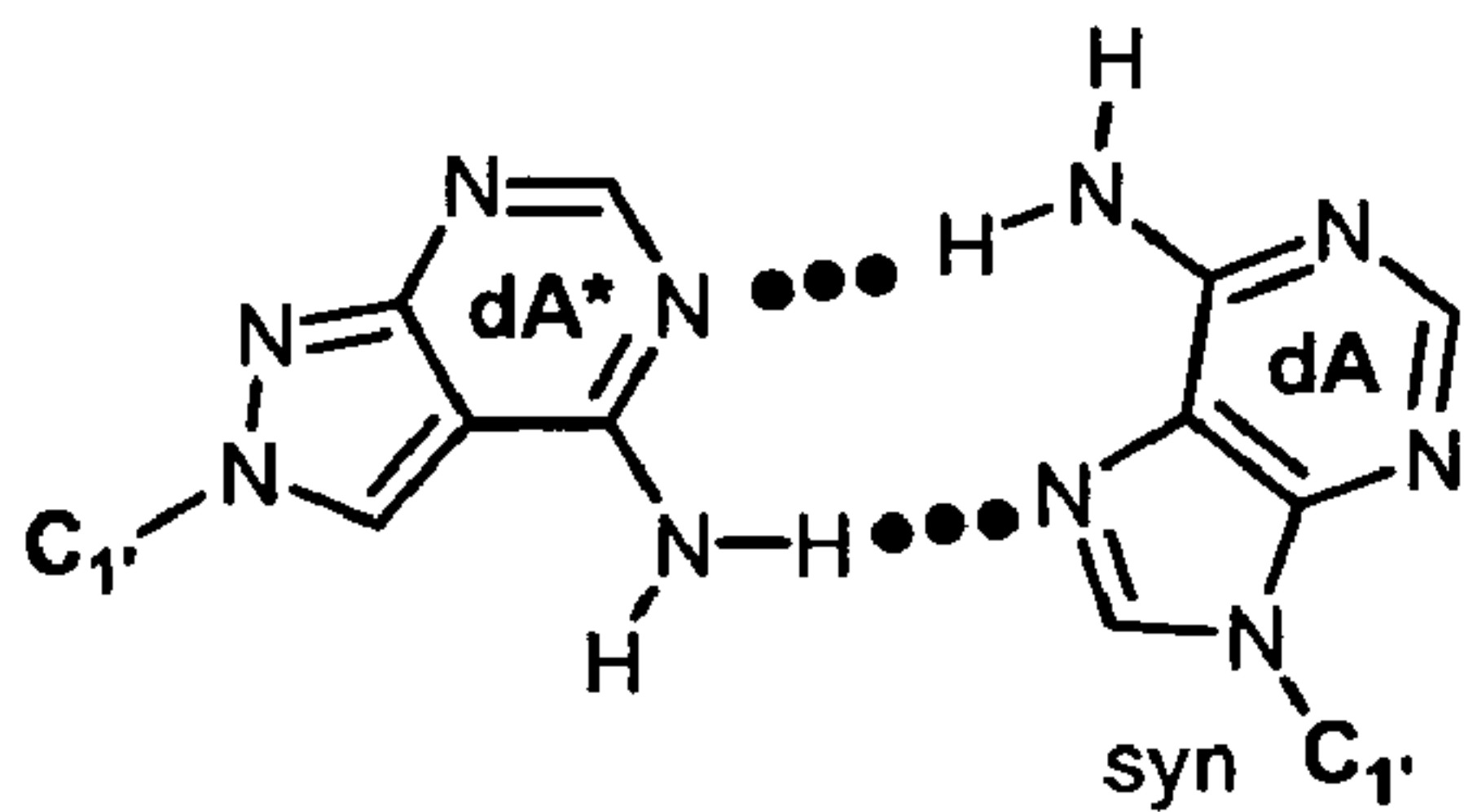
reversed Hoogsteen
