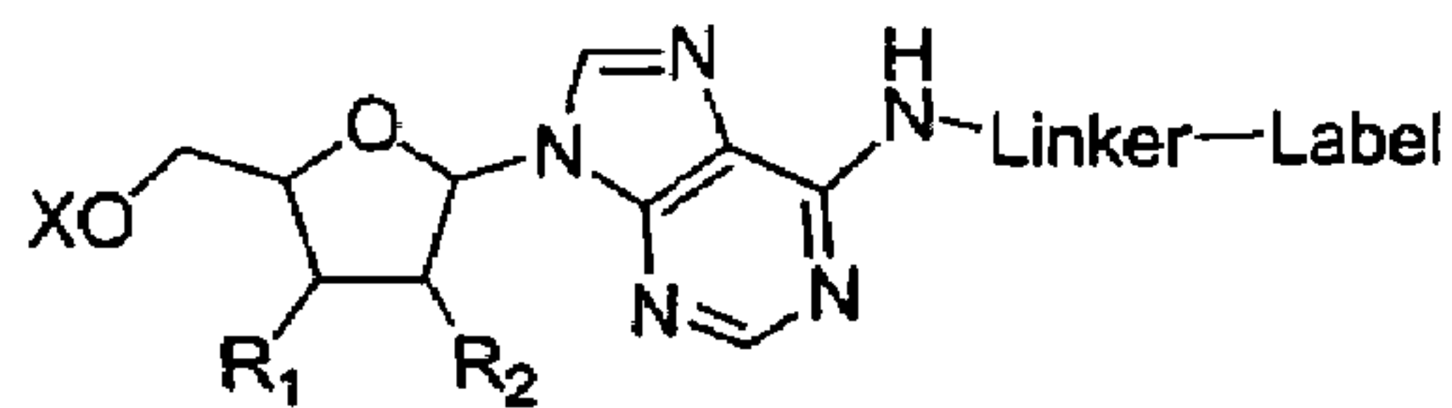
Adenosine N6-linker
