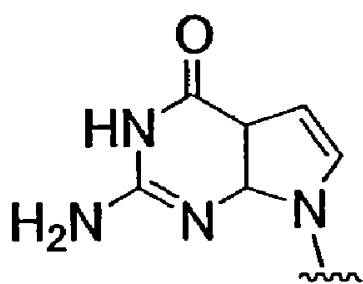
N9-(7-deaza-G)
