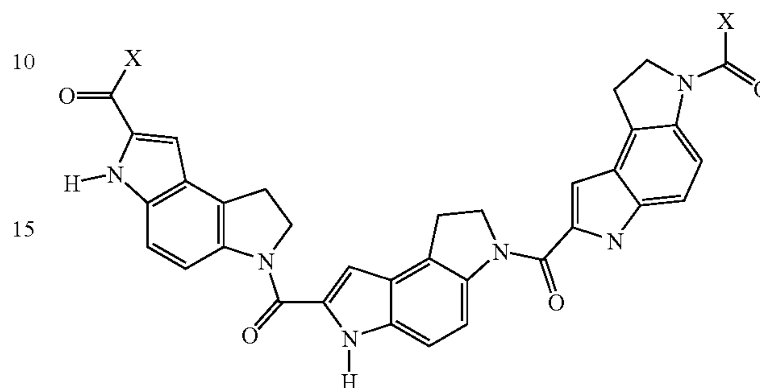
Dabcy1
