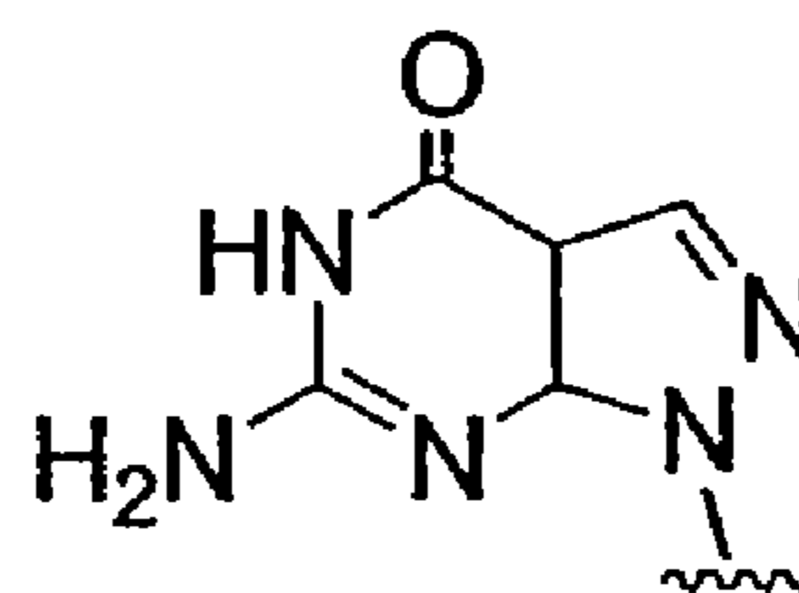
N9-(7-deaza-8-aza-G)
