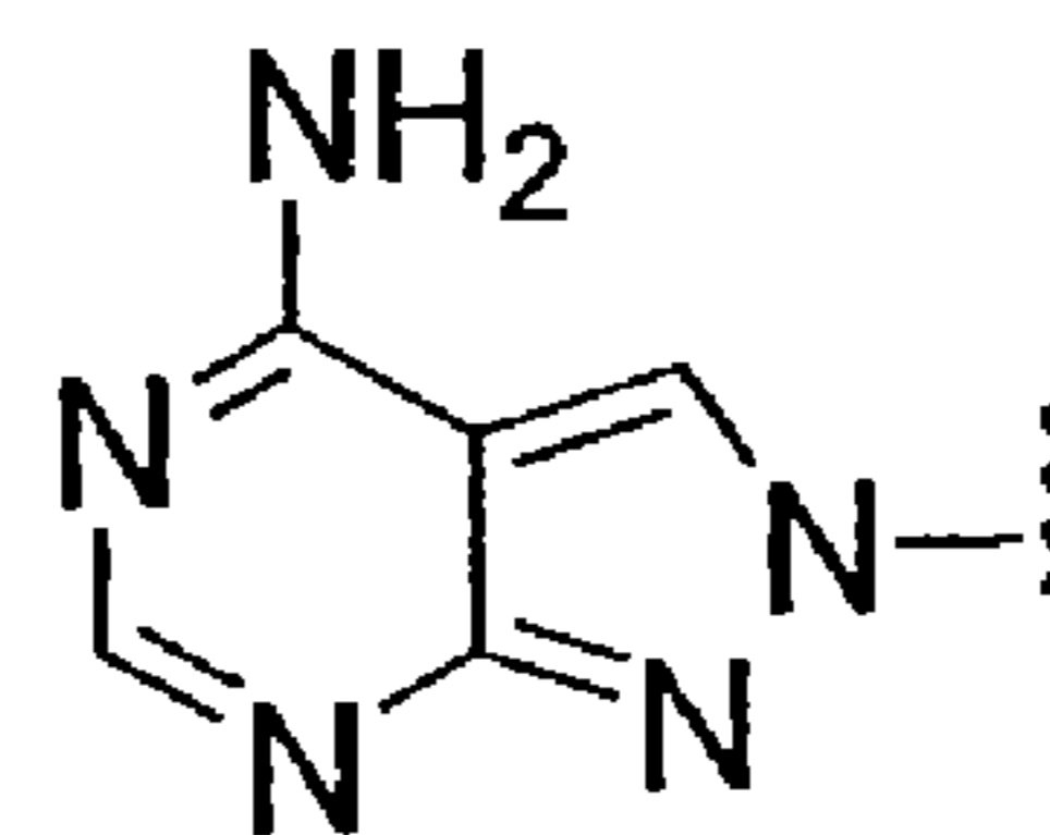
N8-(7-deaza-8-aza-A)
