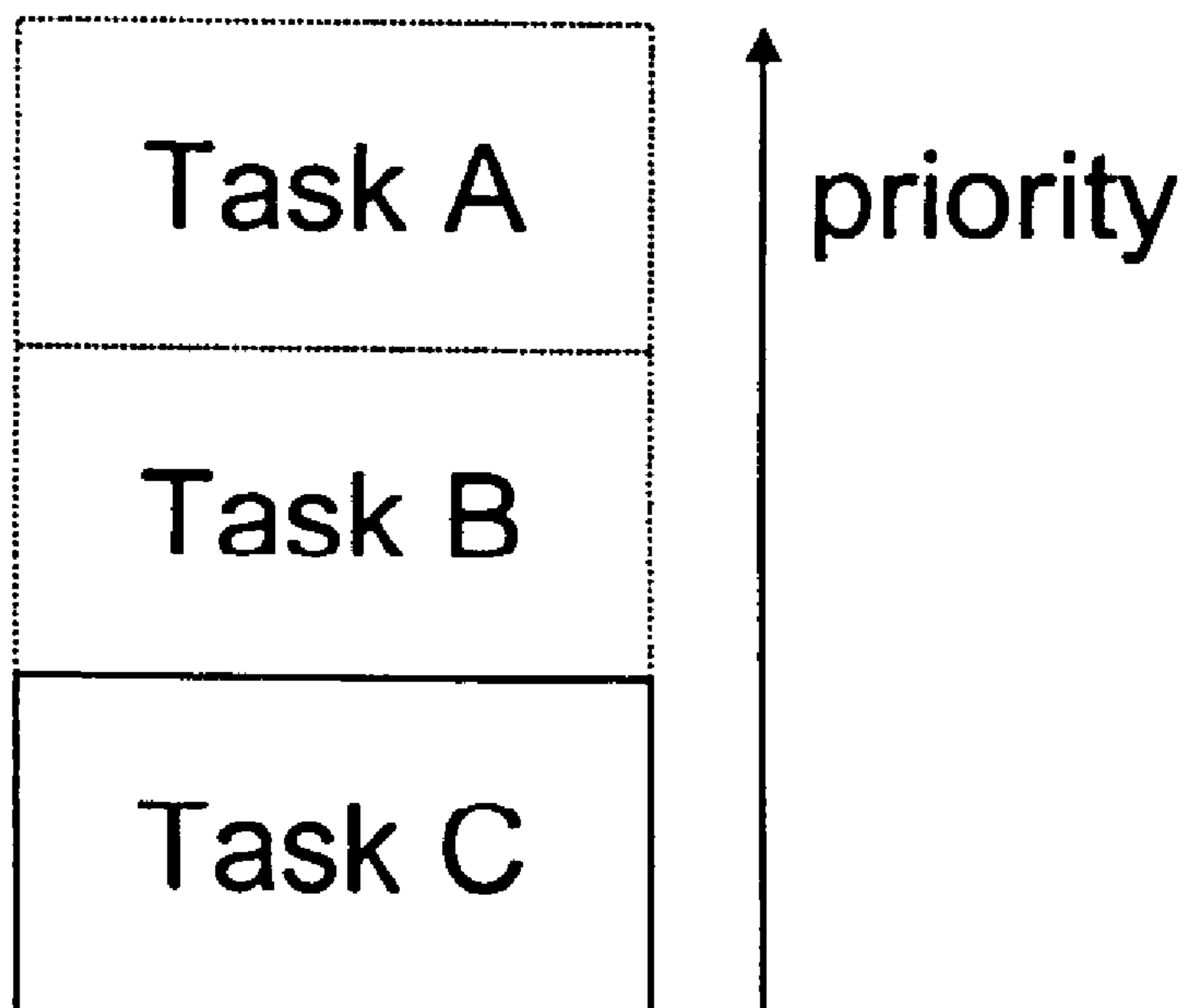
Task table
