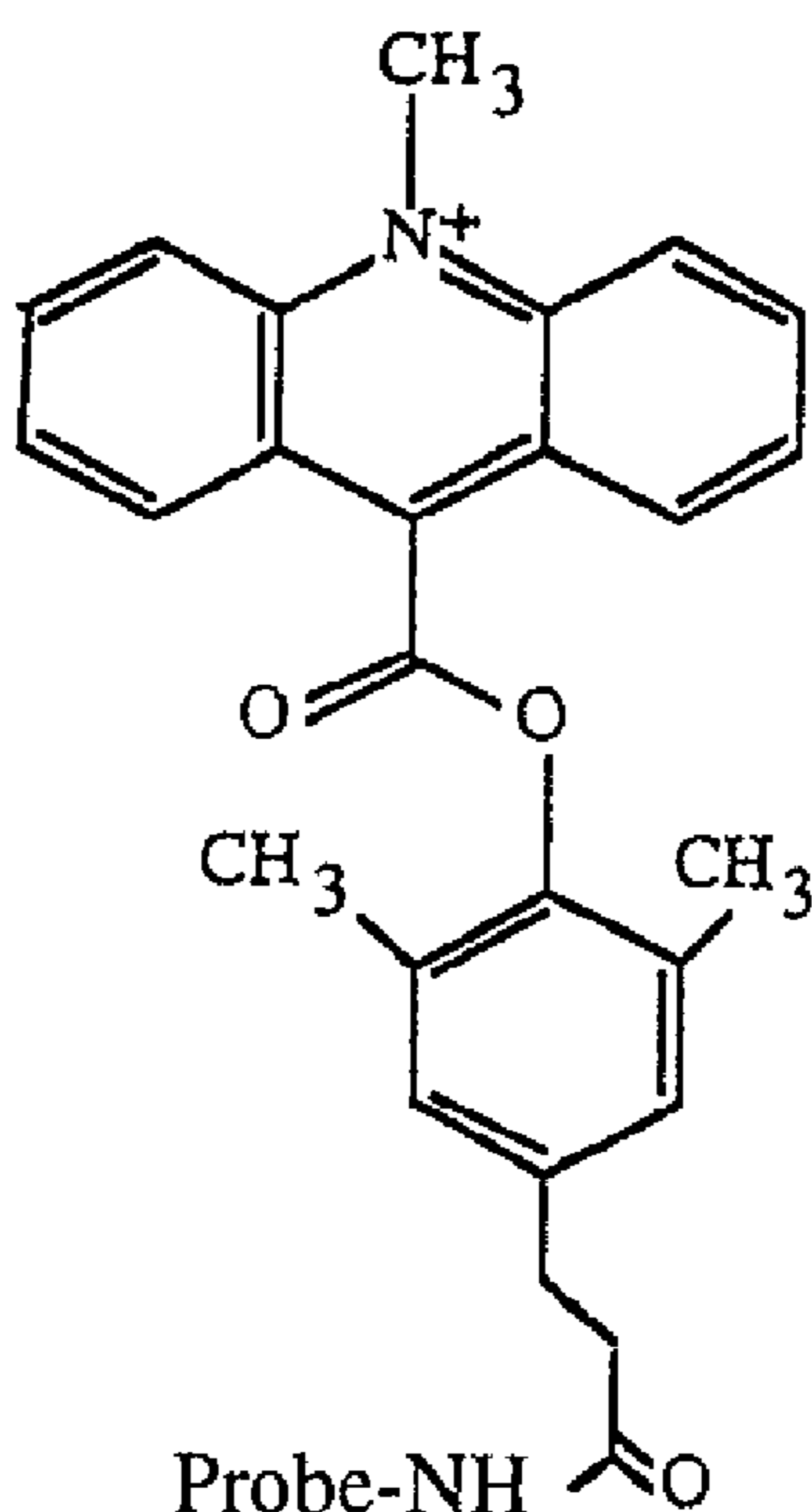
o -diMe-AE
