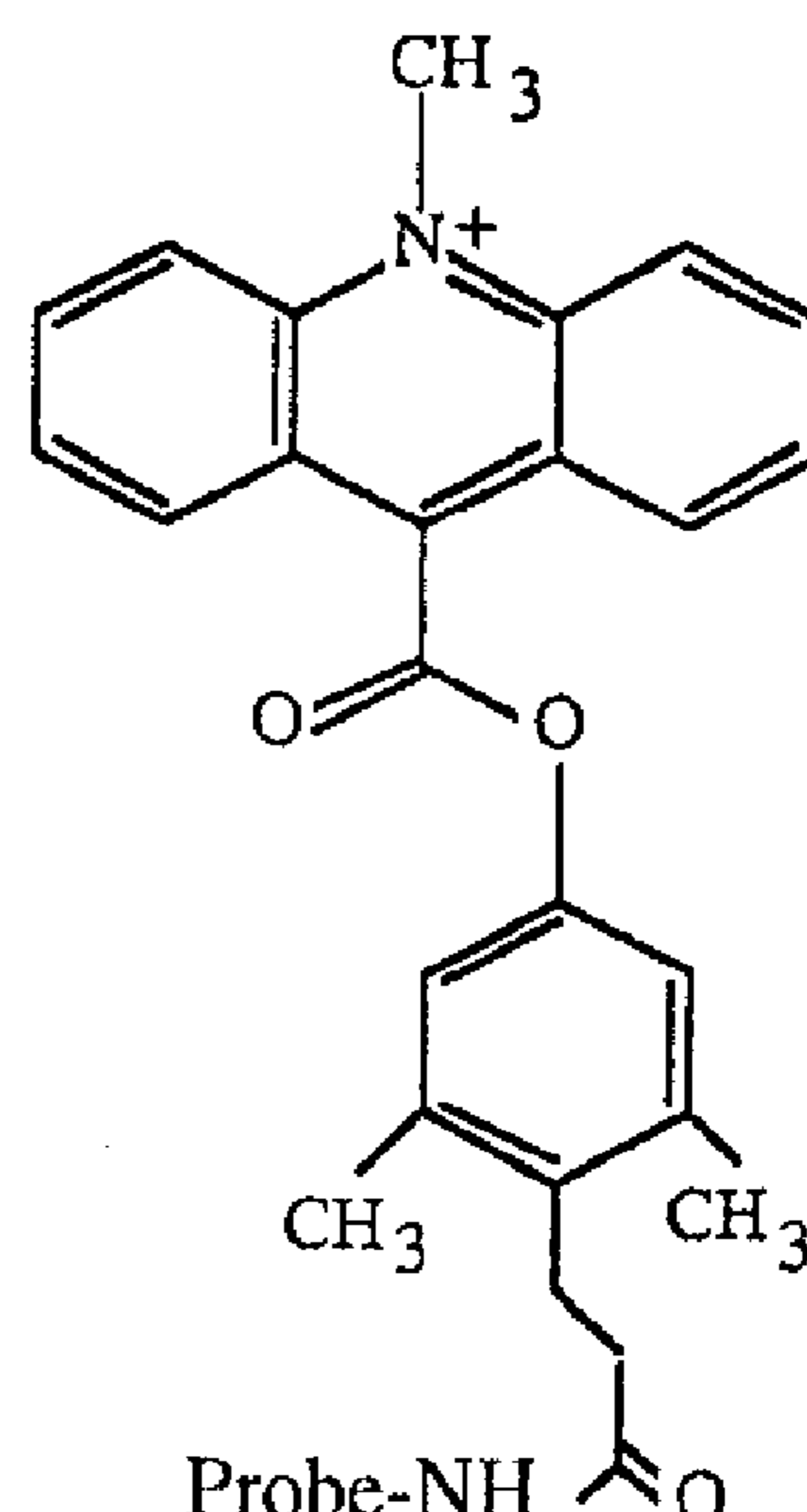
m -diMe-AE
