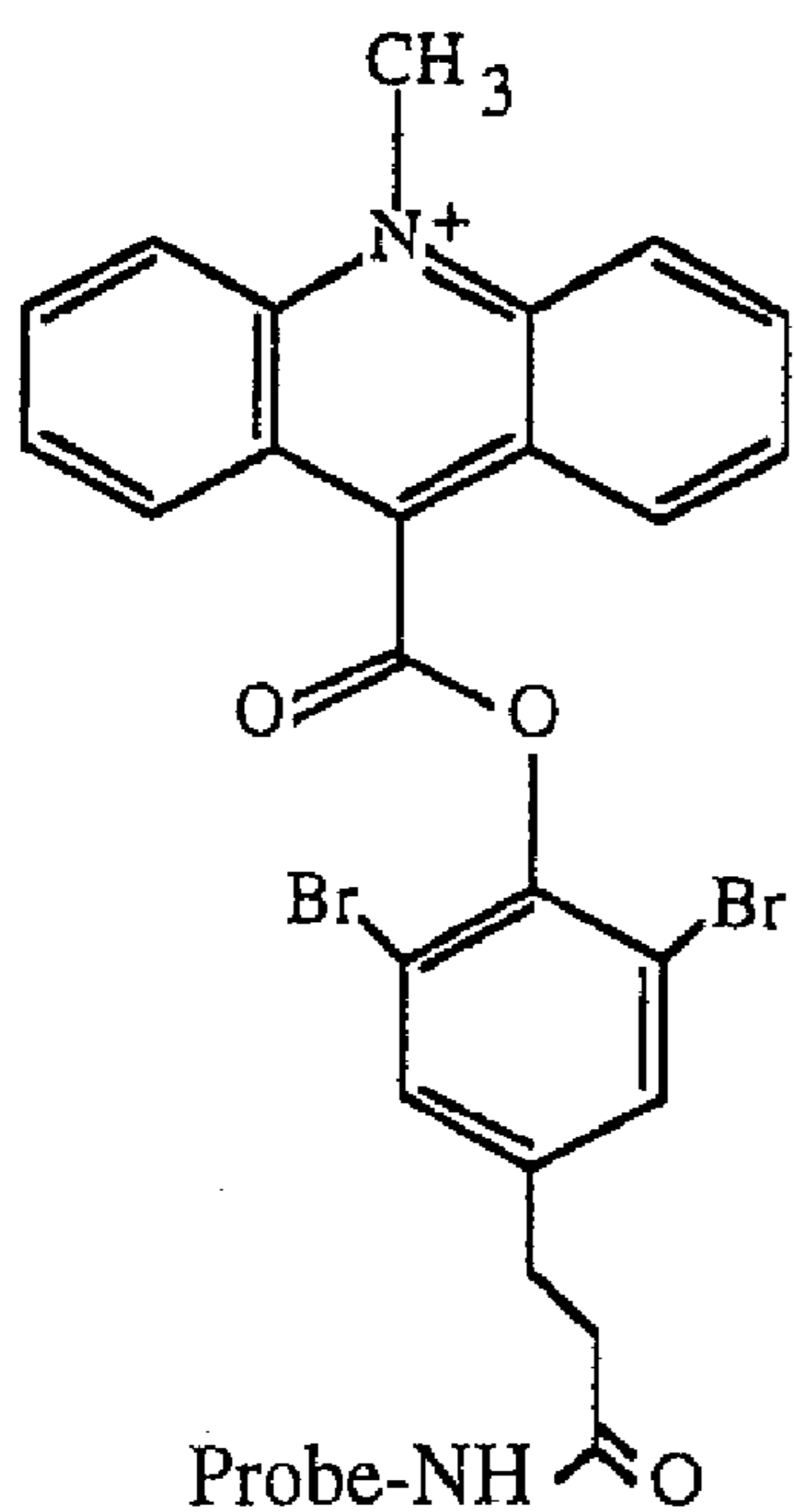
o -diBr-AE
