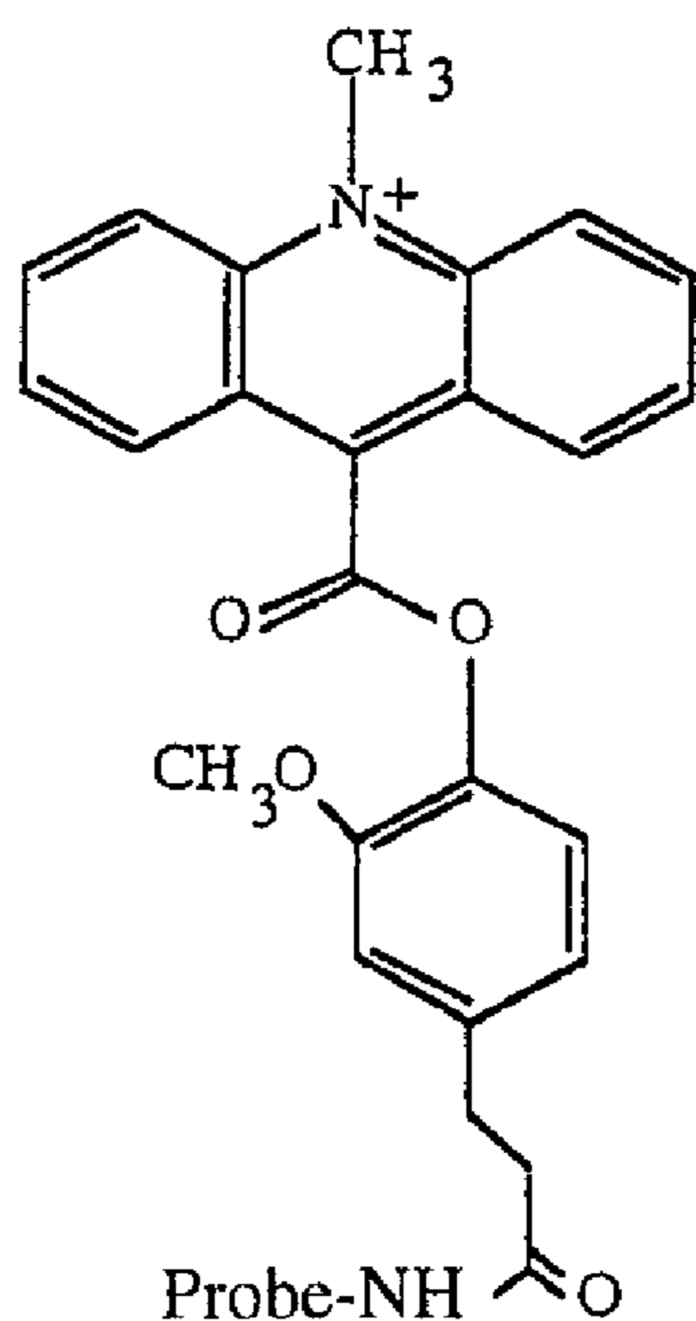
o -MeO-AE
