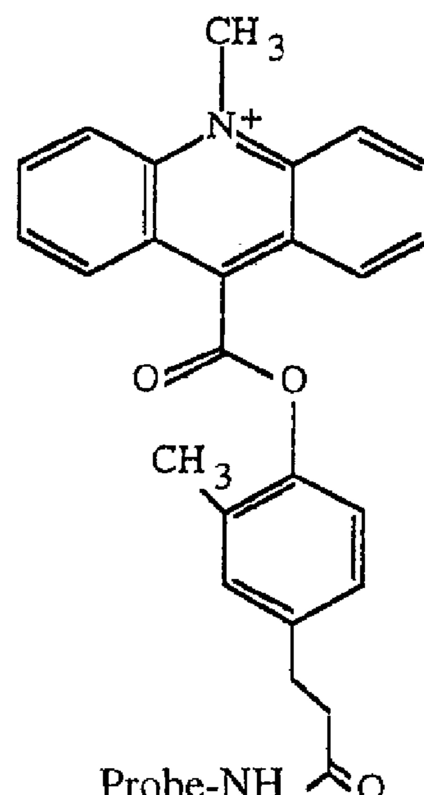
o -Me-AE
