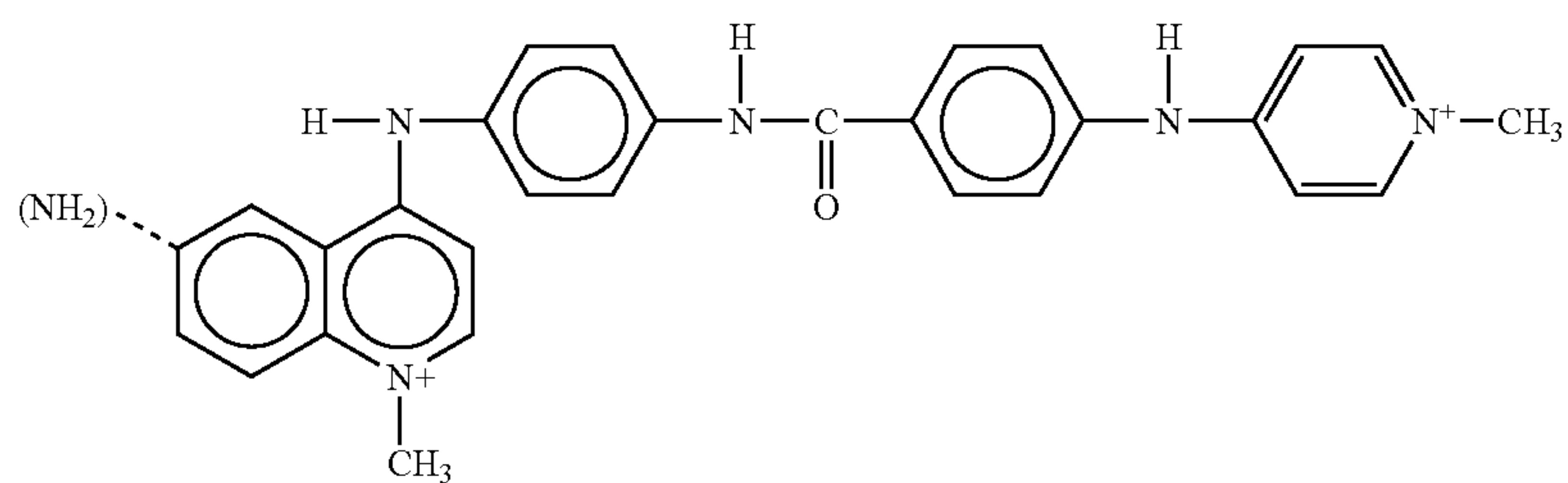
NSC 101327
