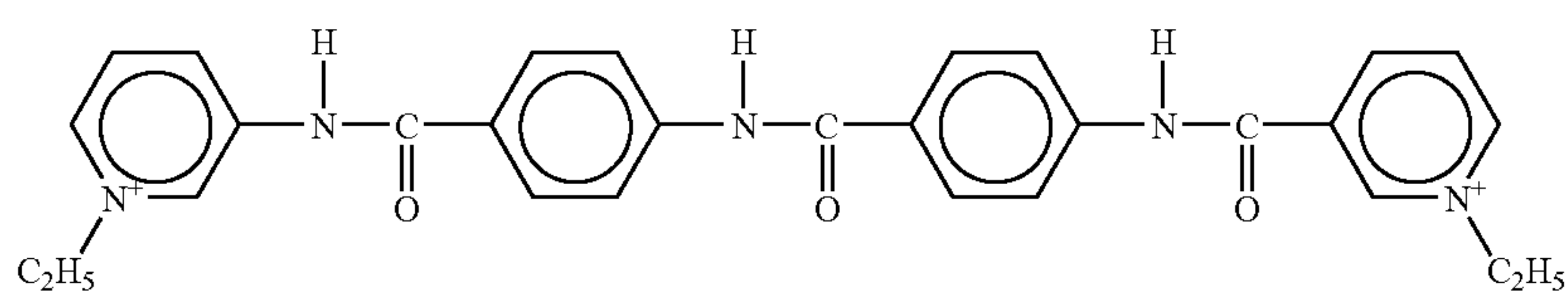
NSC 101327
