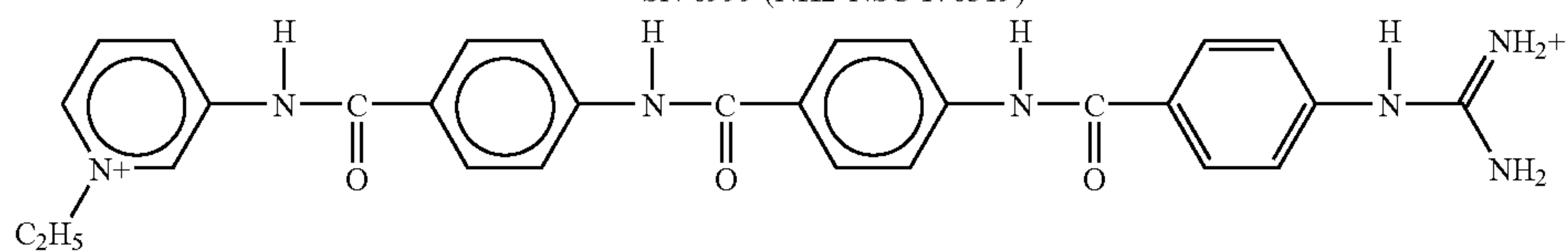
SN 6999 (NH2-NSC 176319)
