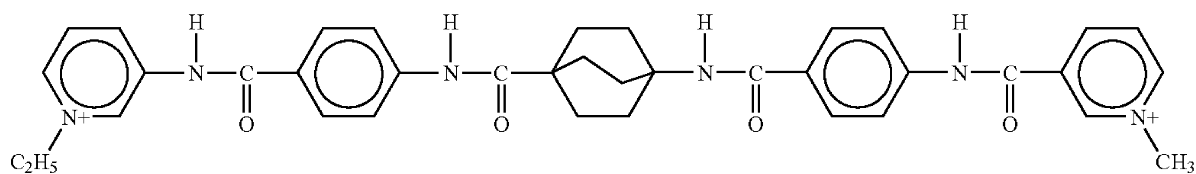
SN 6136
