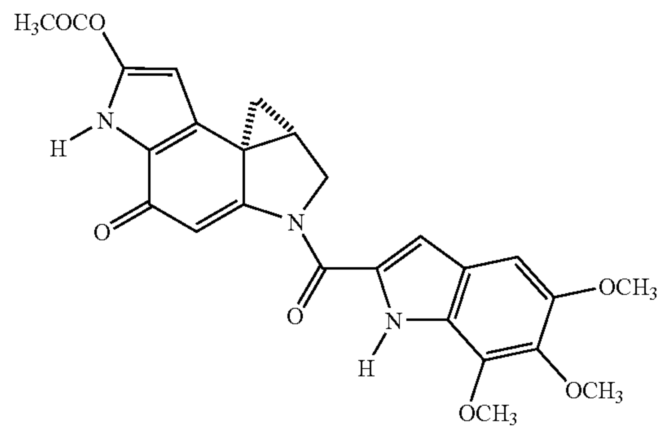
Duocarmycin SA
