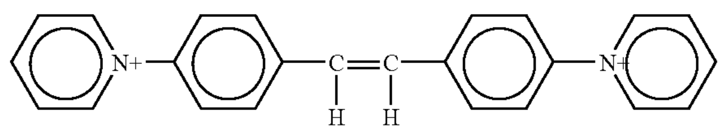
SN 16814
