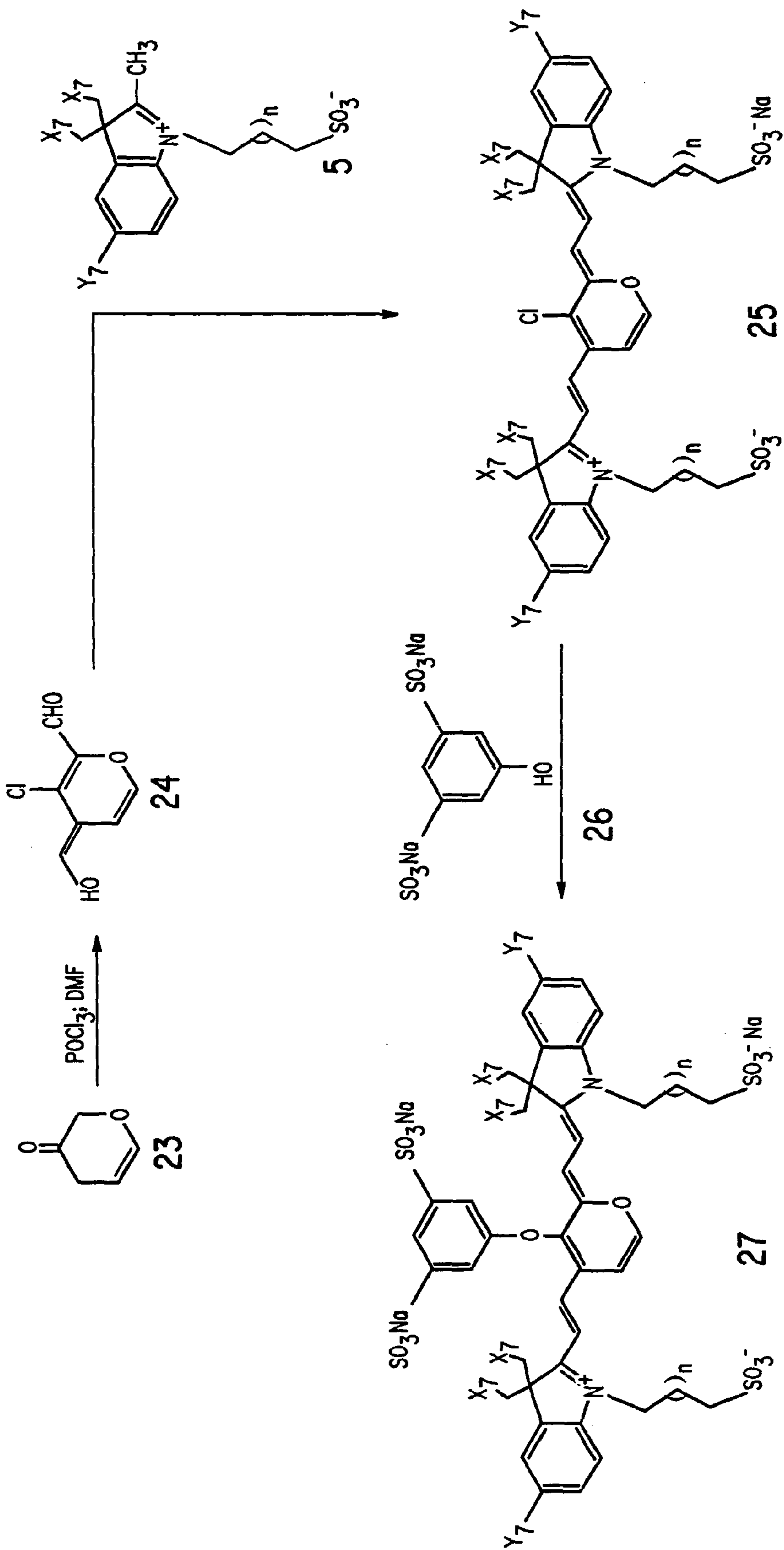
FIG. 7 : n = 1-3; X_7 = H, OH; Y_7, Y_8 = H, SO_3^-, CO_2H, CH_2CO_2H, CH_2OH
