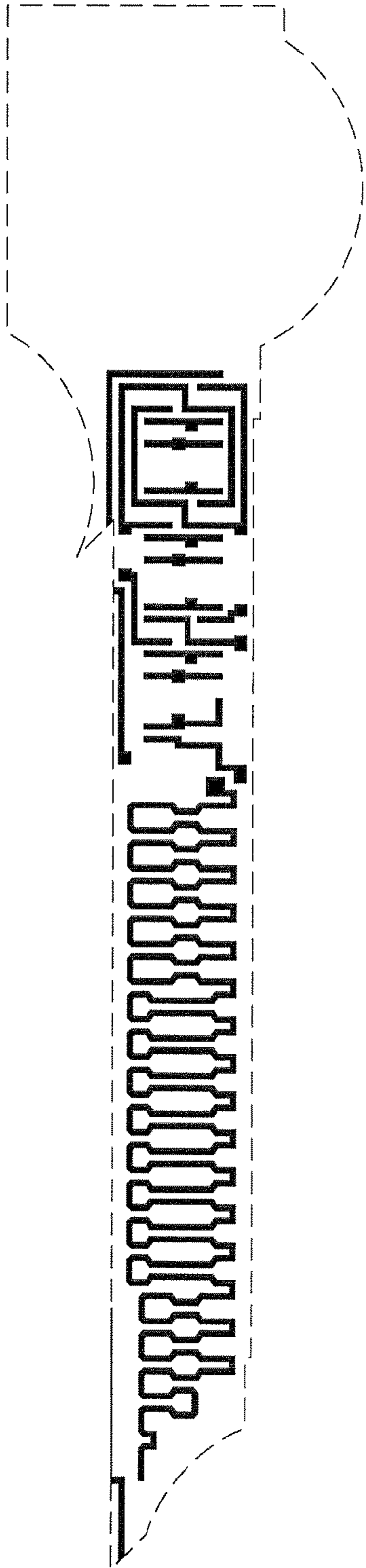
Poly mask
