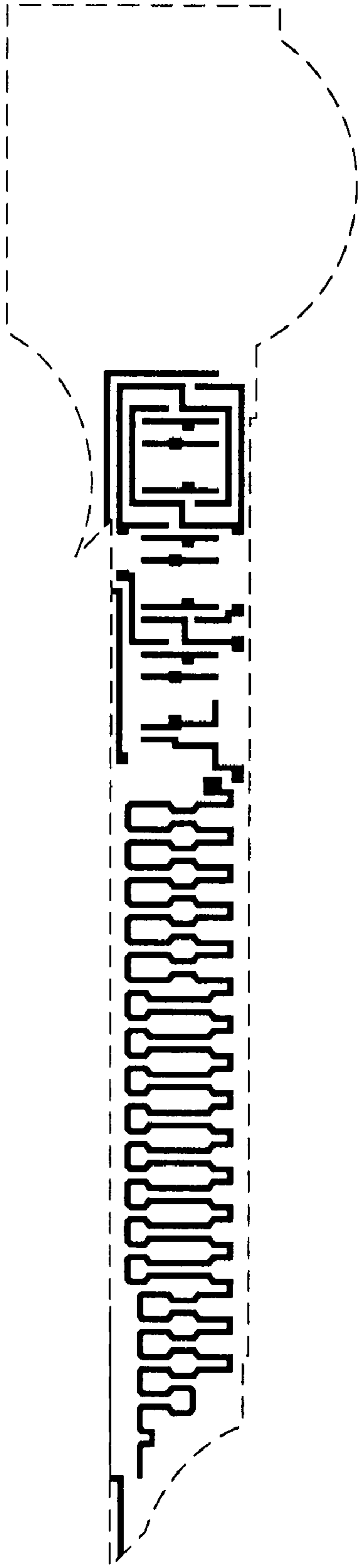
Poly mask
