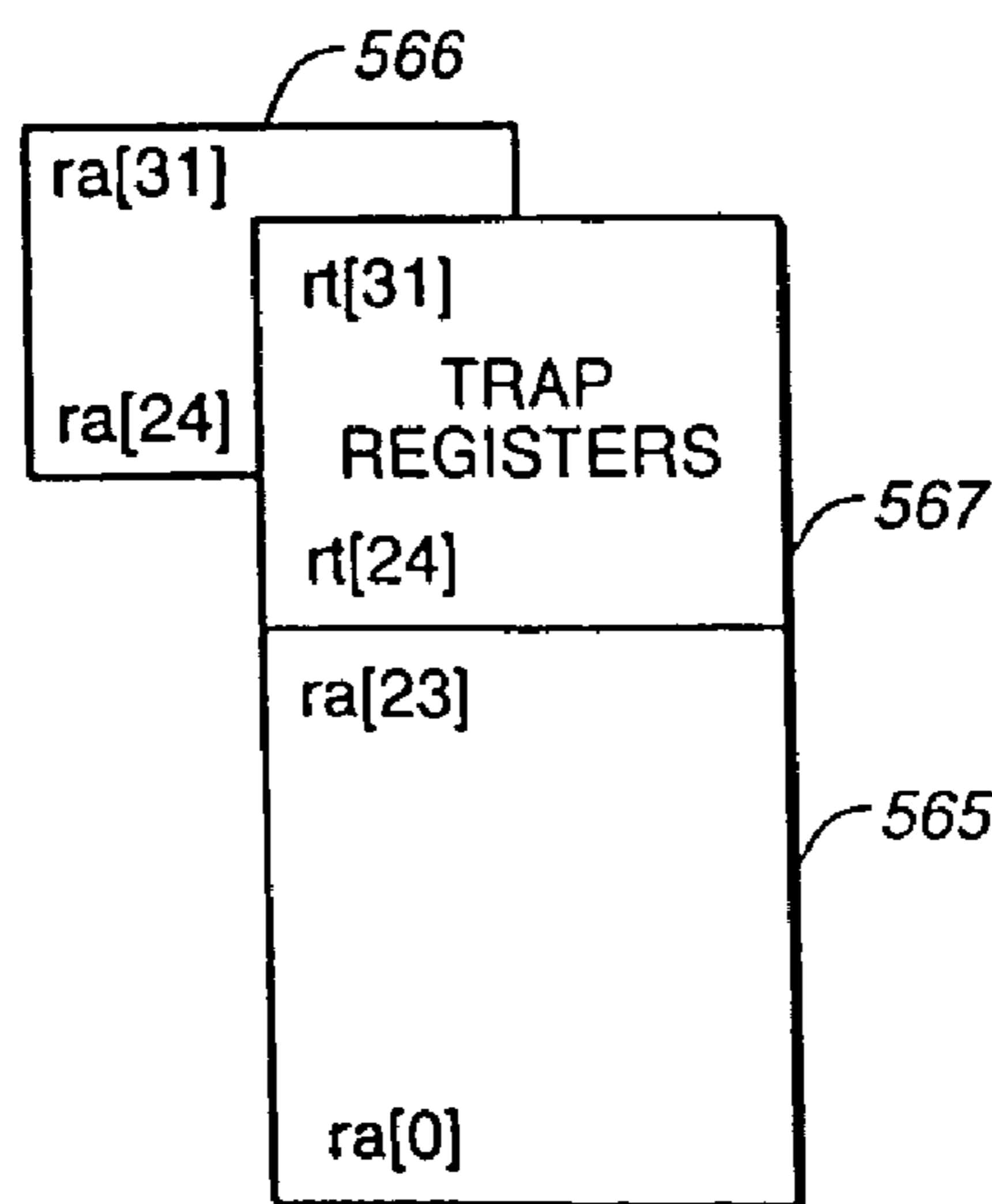
FIG. 7B
