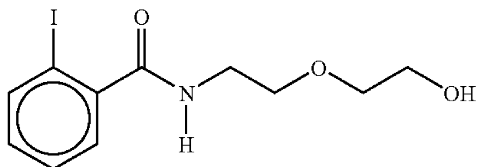
2-[N-(2-iodobenzoyl)aminoethoxy]ethanol
