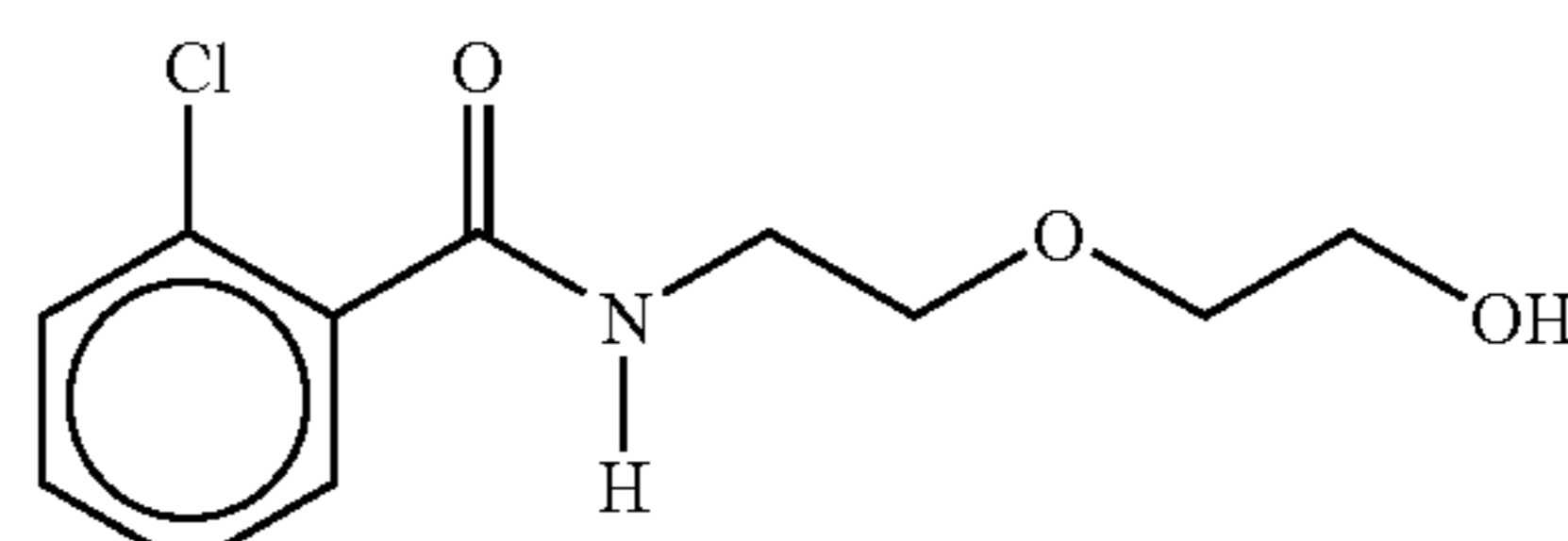
2-[2-N-(2-chlorobenzoyl)aminoethoxy]ethanol
