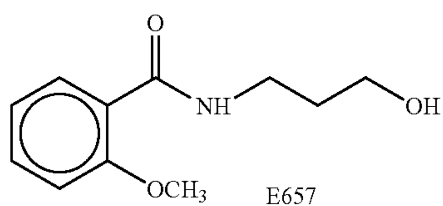
3-(2-methoxybenzoylamino)-1-propanol E657
