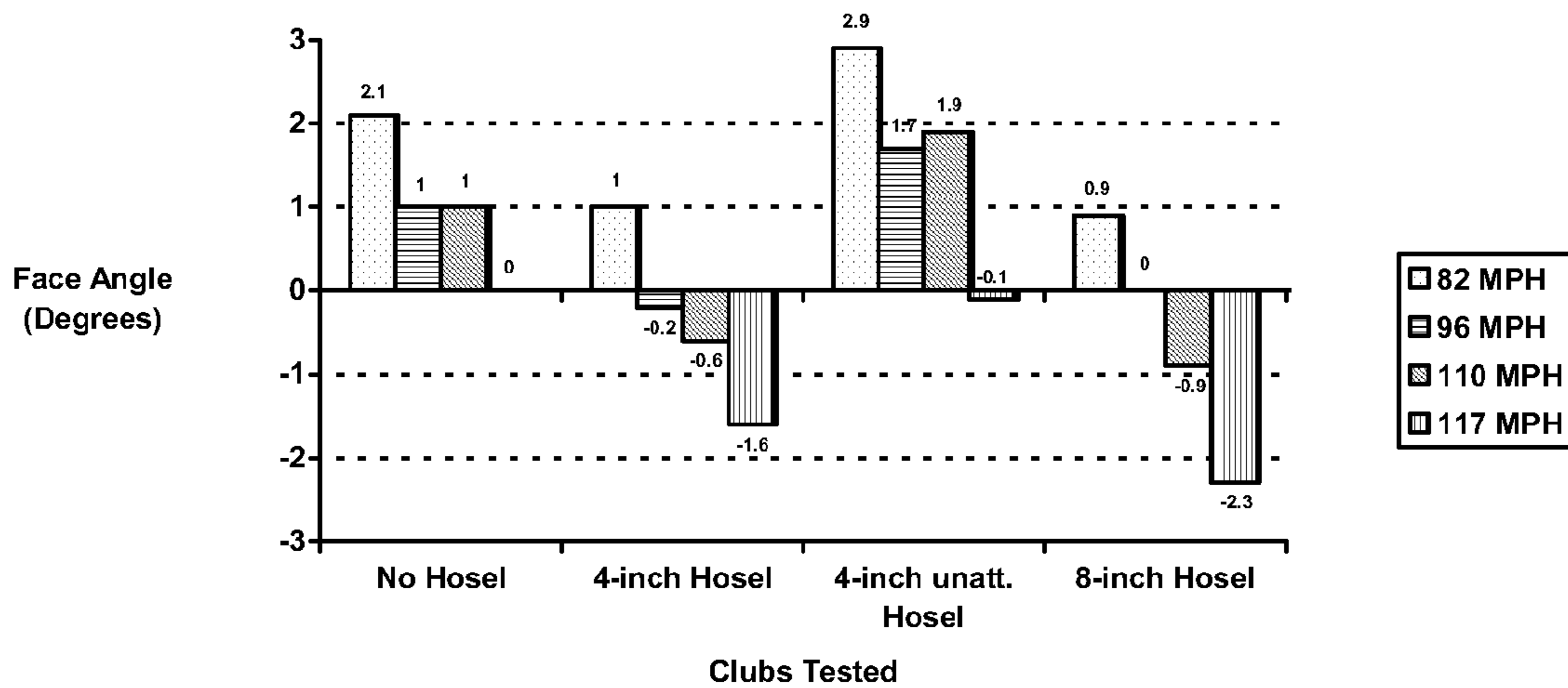
Fig. 13 Face Angle
