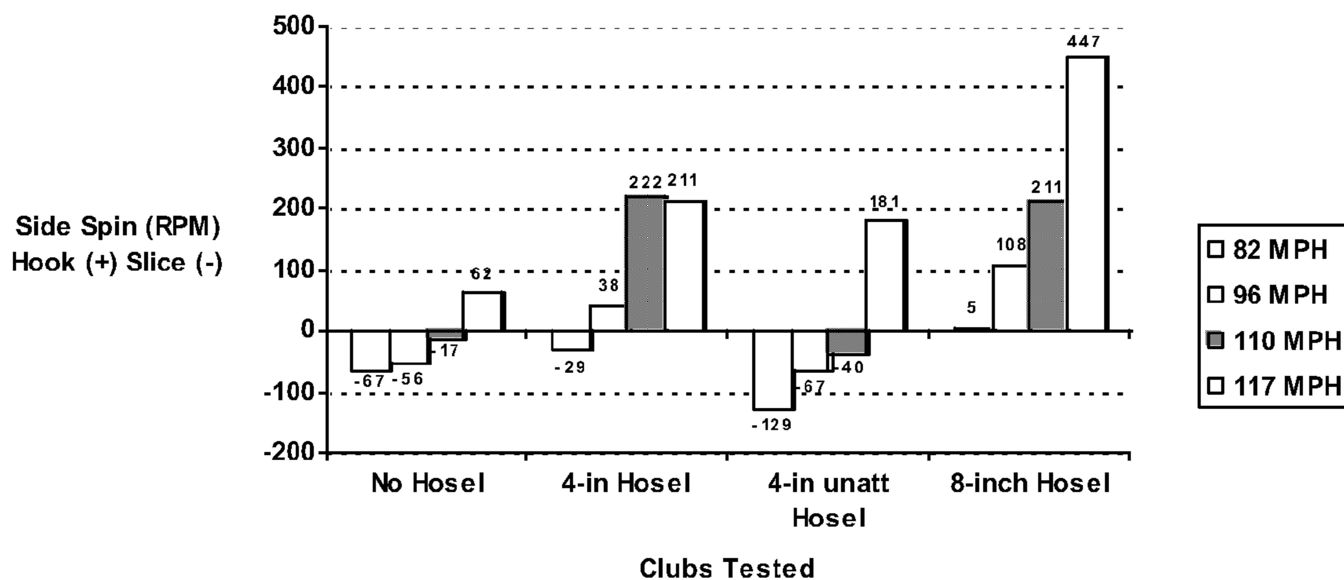
Fig. 12 Side Spin
