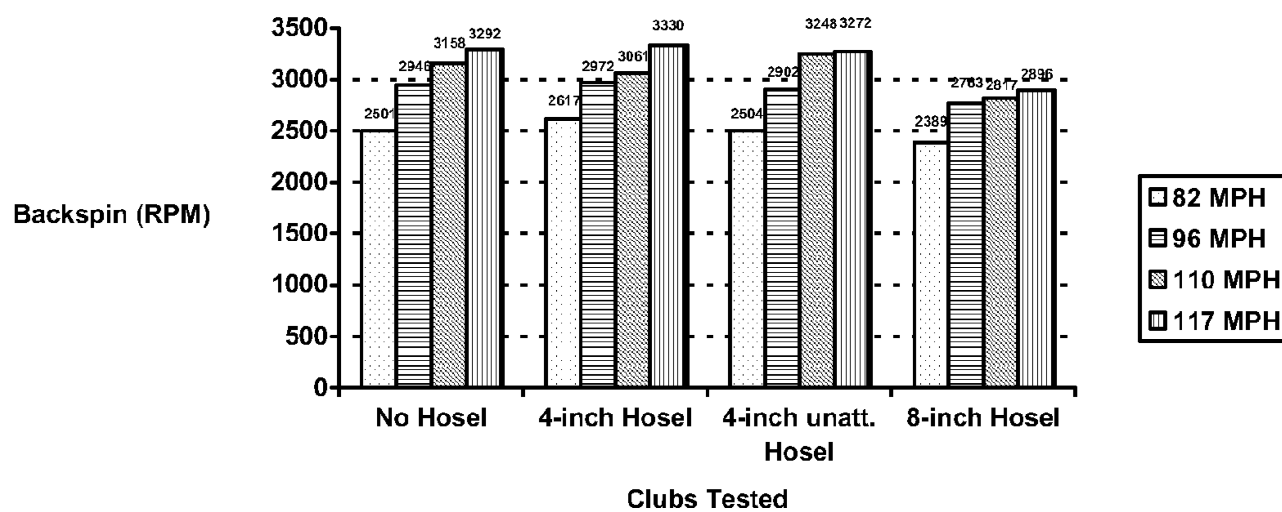
Fig. 16 Backspin
