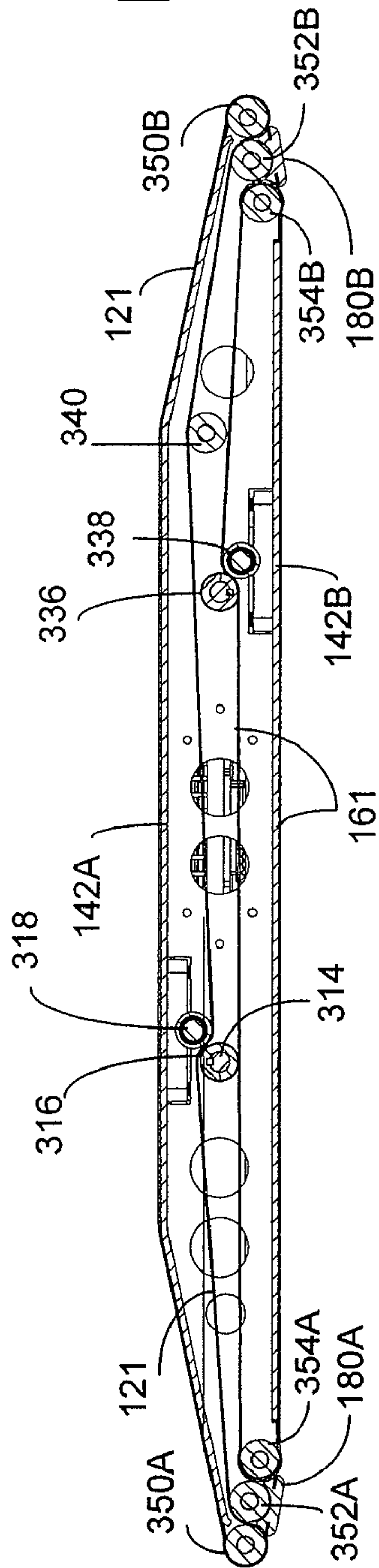
FIG. 3B
