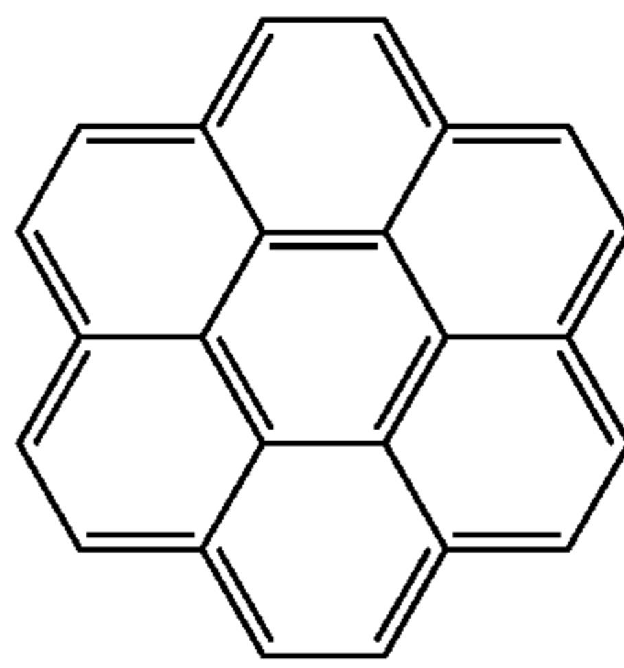
Coronene
