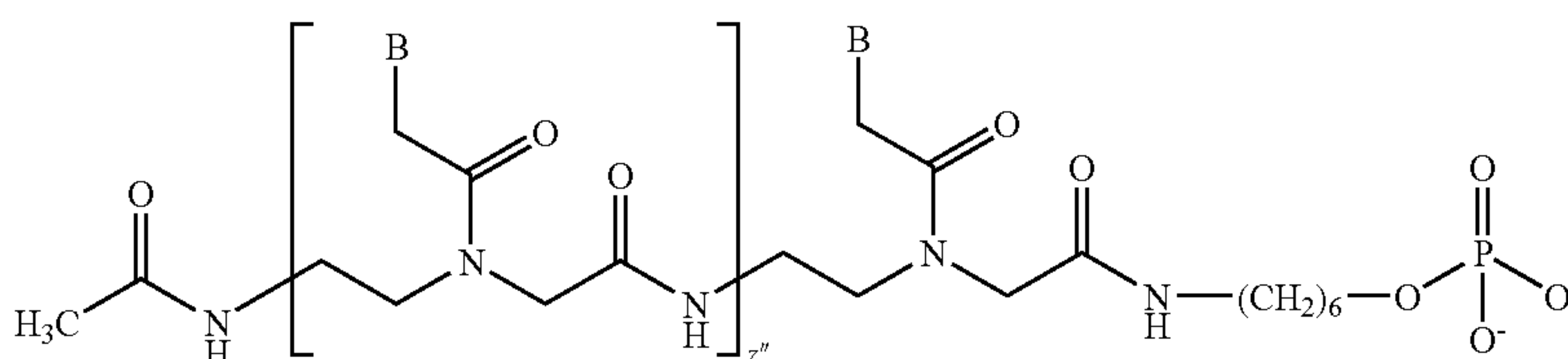
PNA-1:
