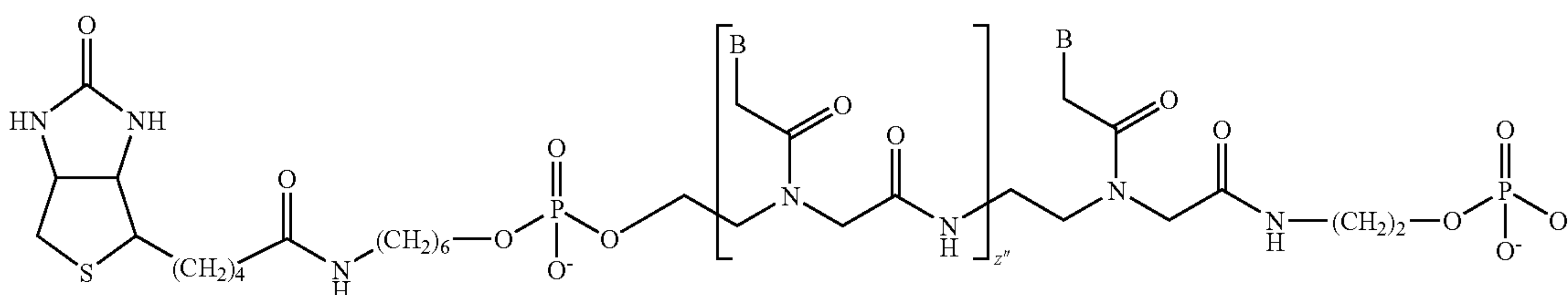
PNA-4:
