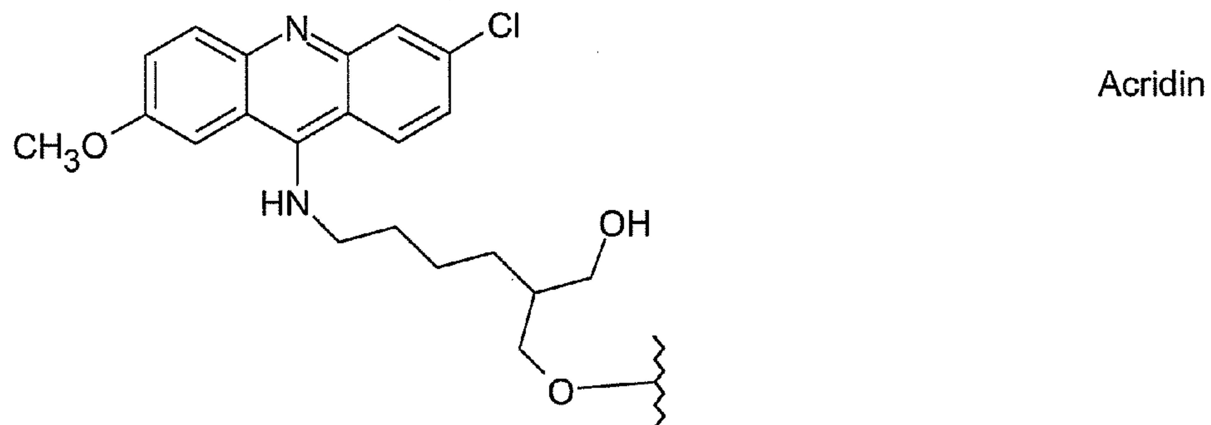
DNP
