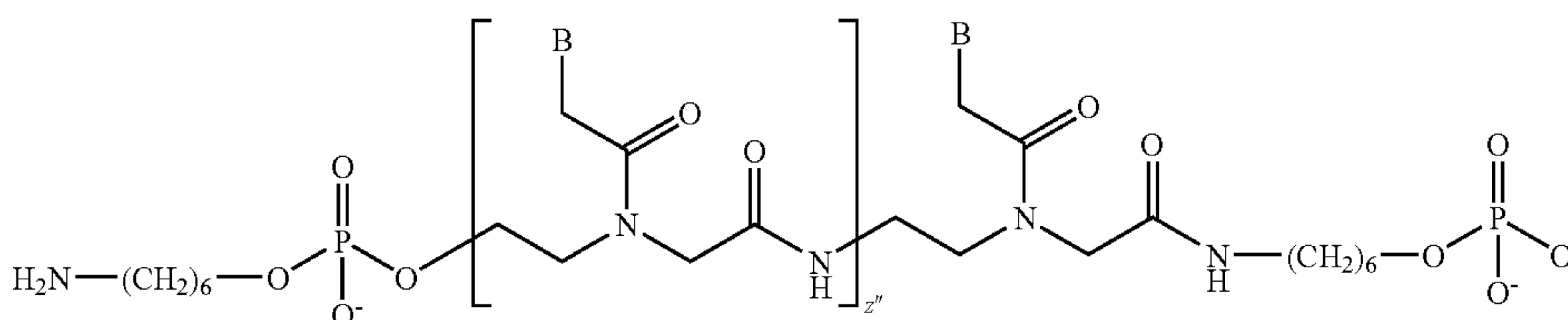
PNA-3:
