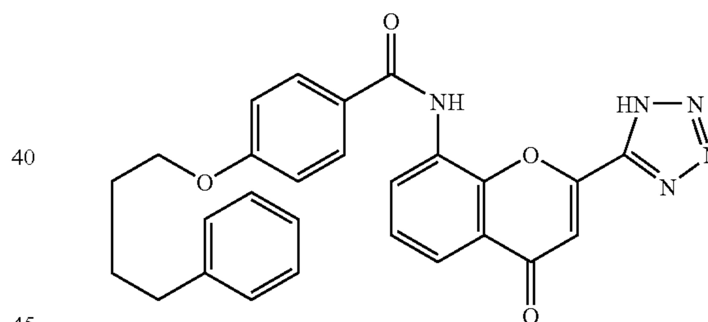
Pranlukast
