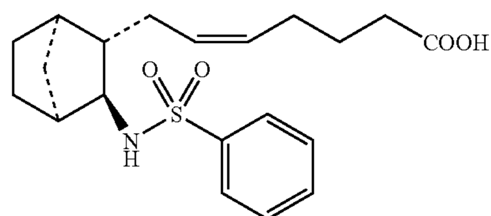
Domitroban
