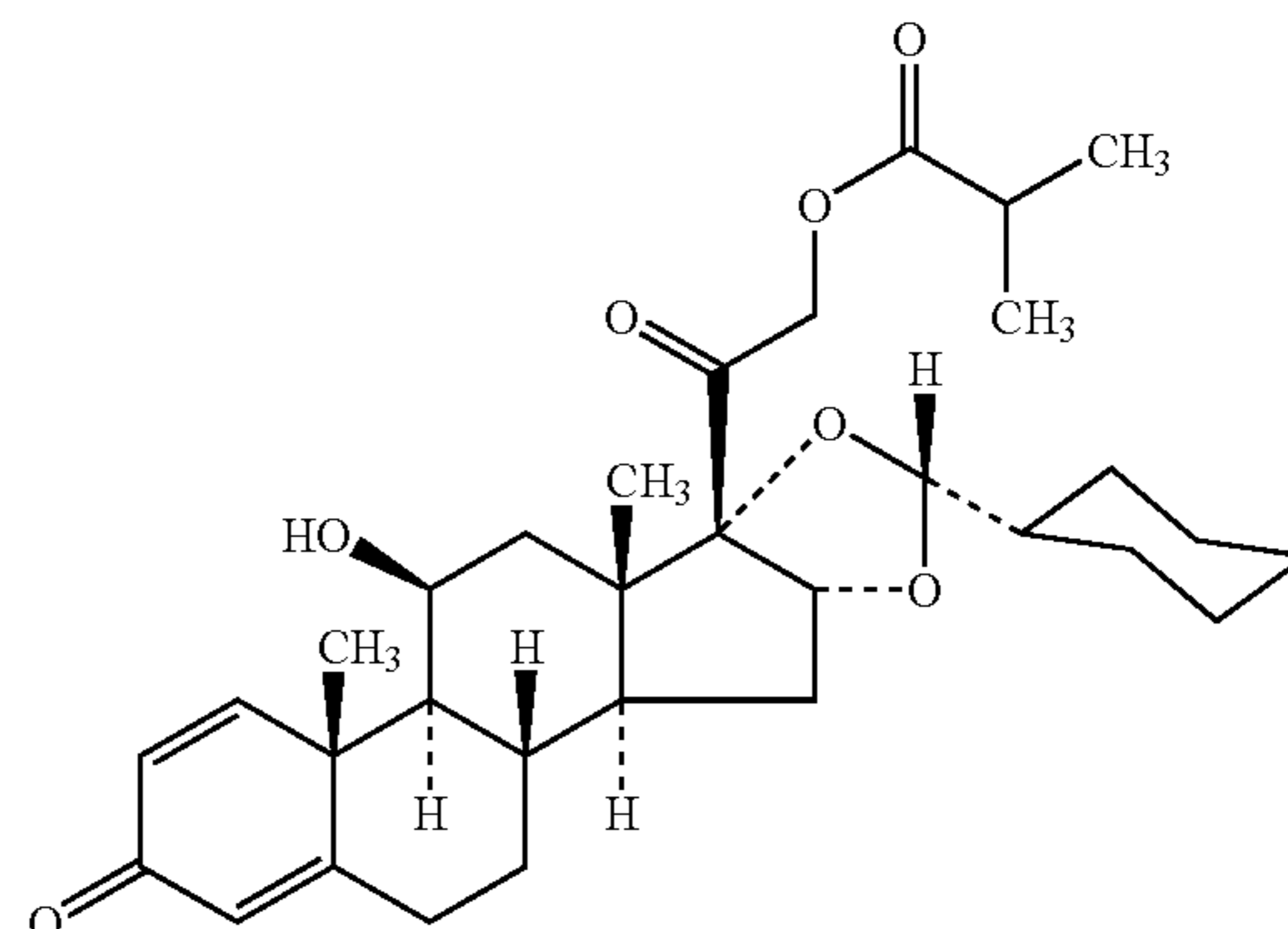
Ciclesonide
