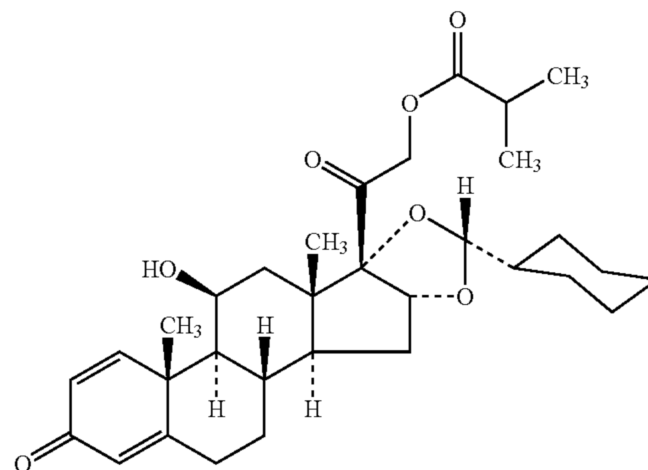
Ciclesonide
