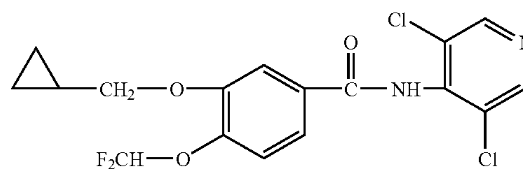
Roflumilast
