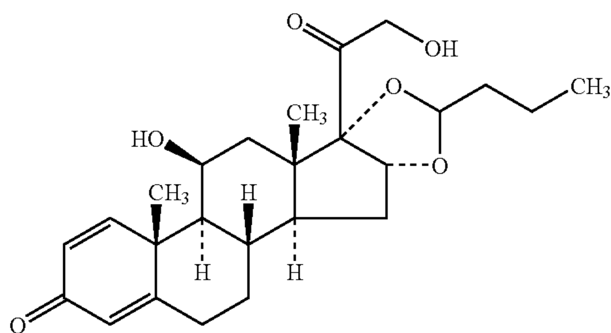
Budesonide
