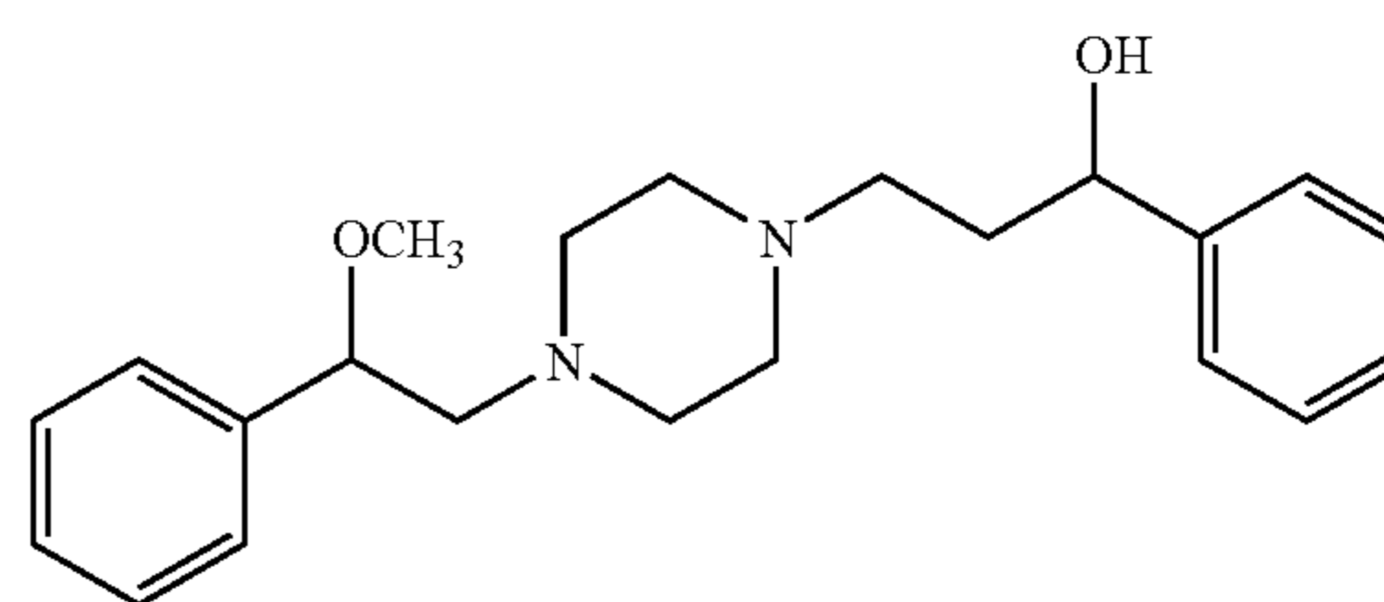
Eprozinol
