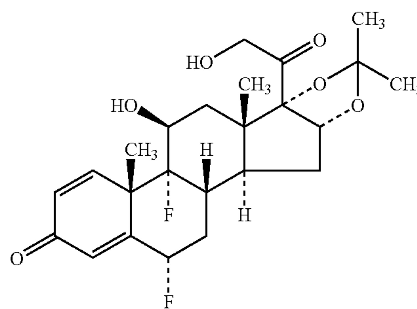
Flunisolide
