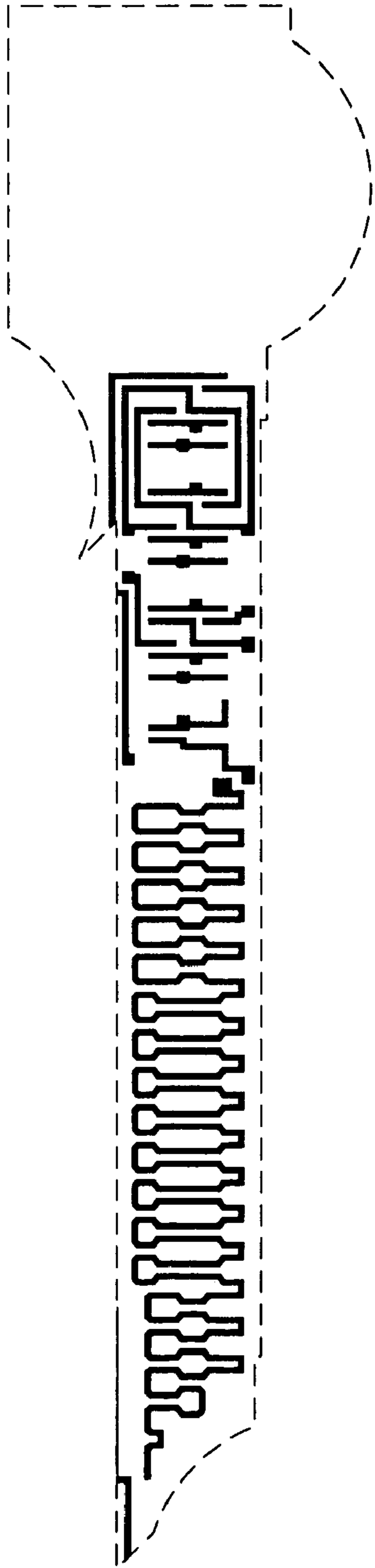
Poly mask
