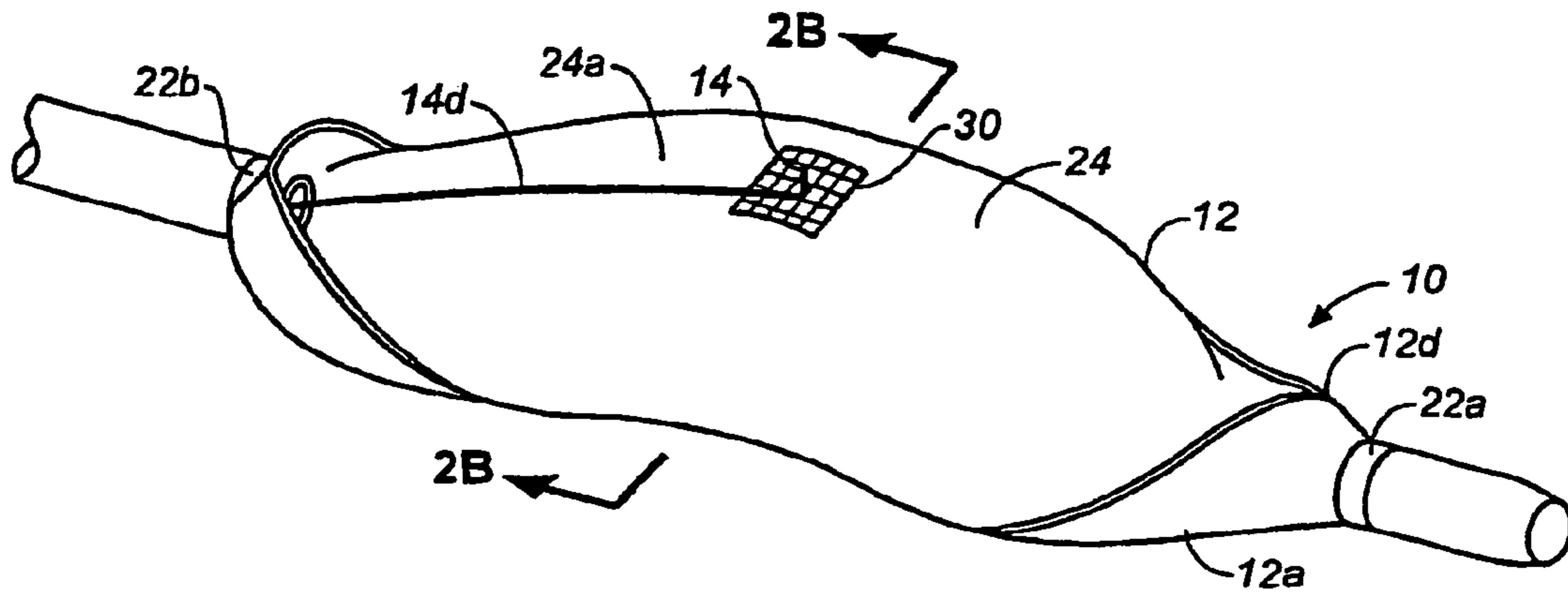
FIG. 2A
