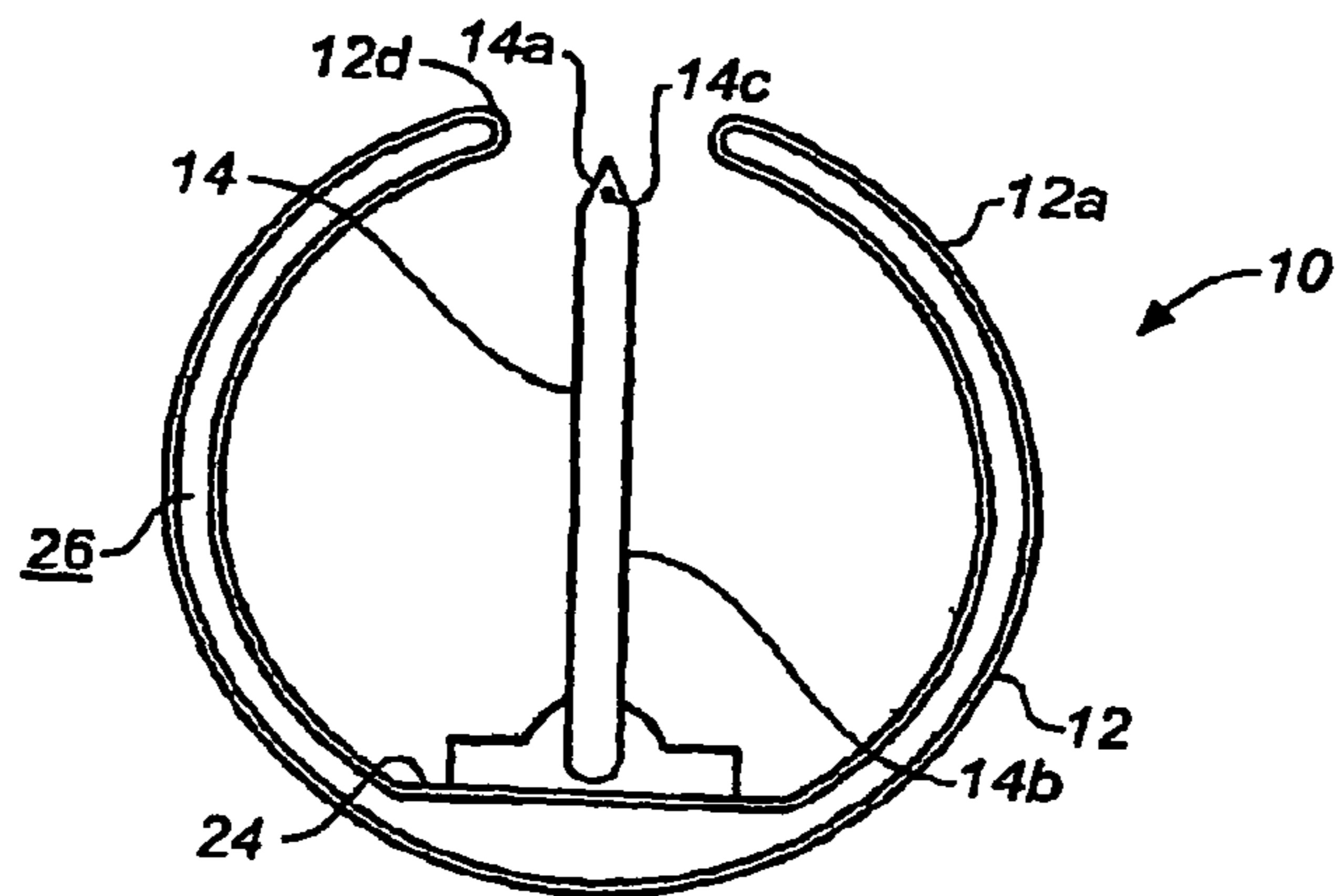
FIG. 1B
