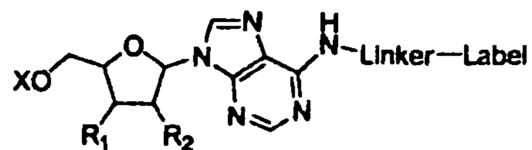
Adenosine N6-linker
