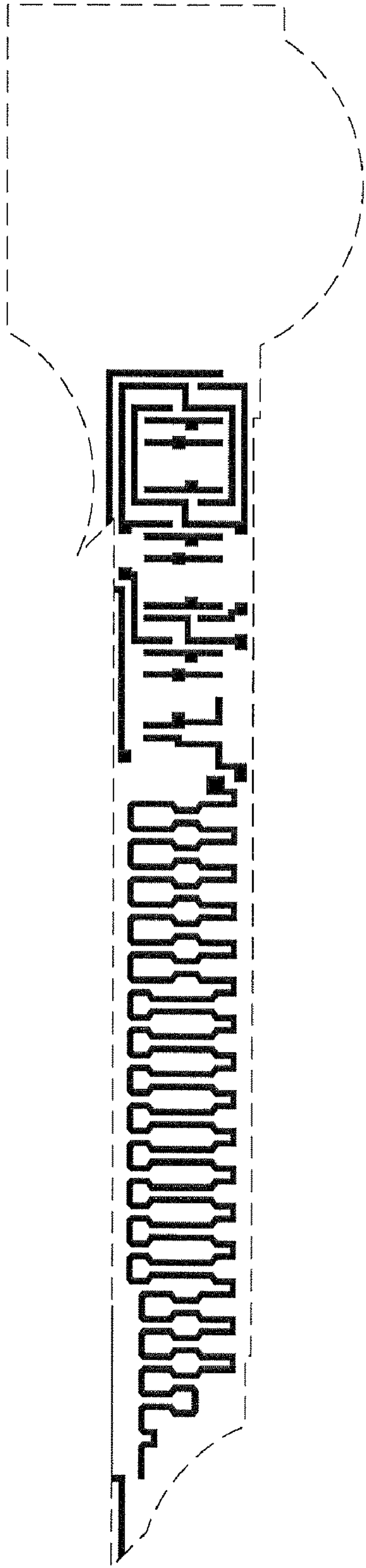
Poly mask
