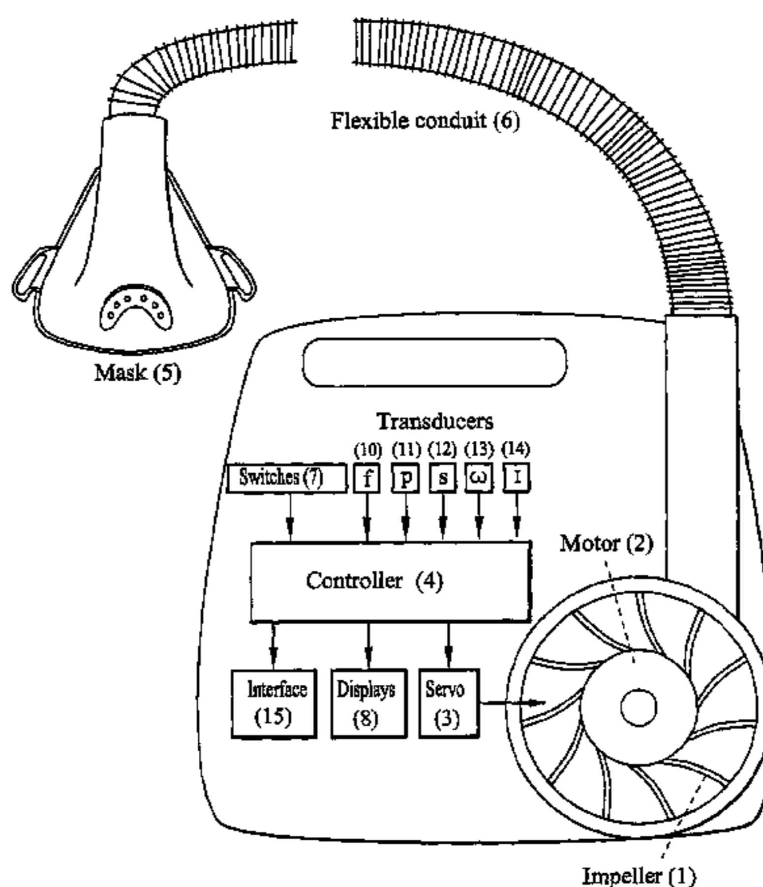
CPAP apparatus
