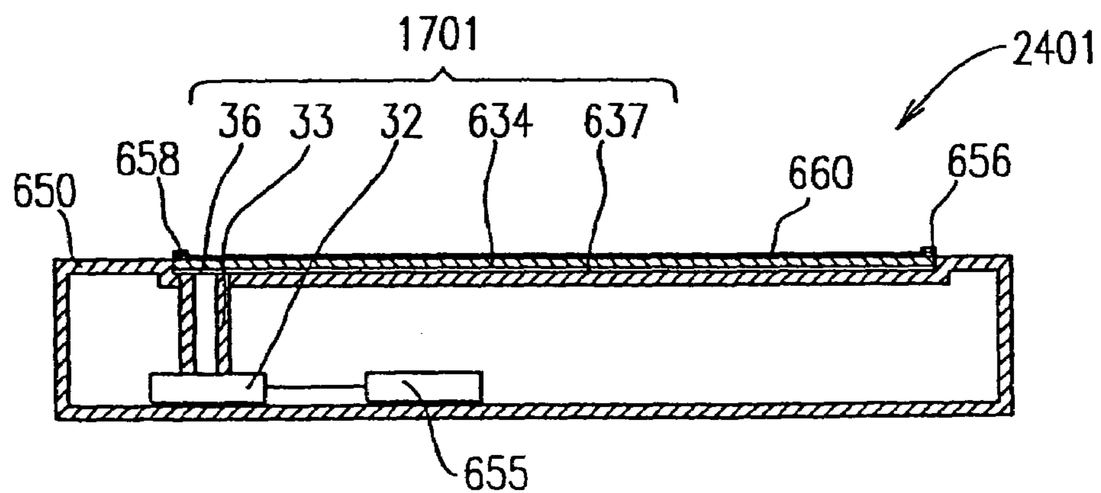
FIG. 23B
