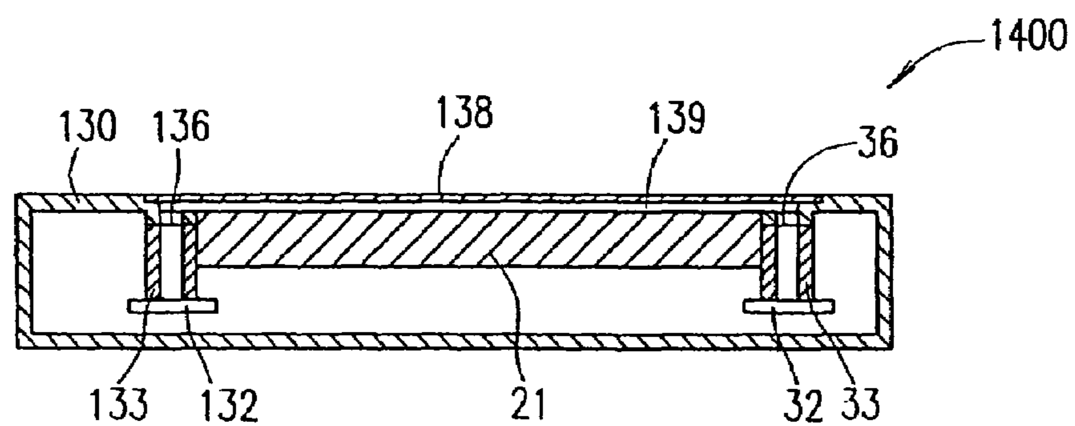
FIG. 10B
