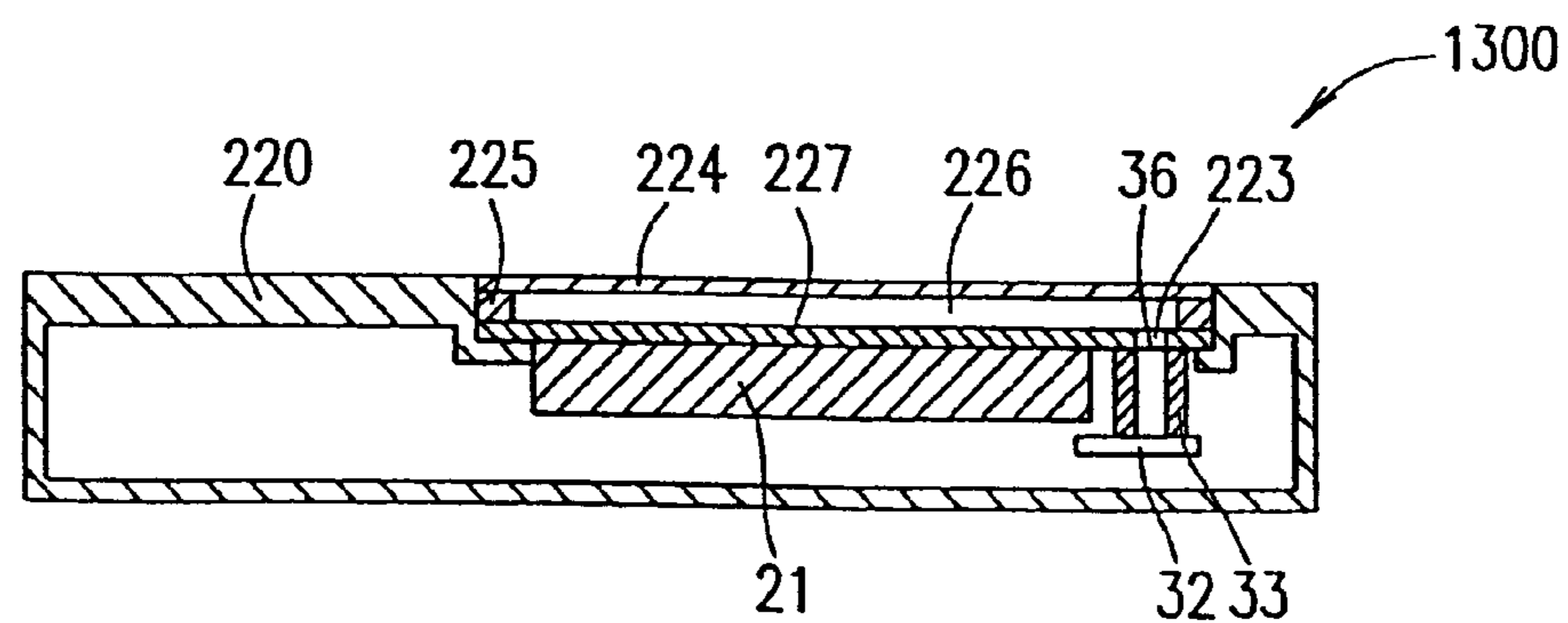
FIG. 9B
