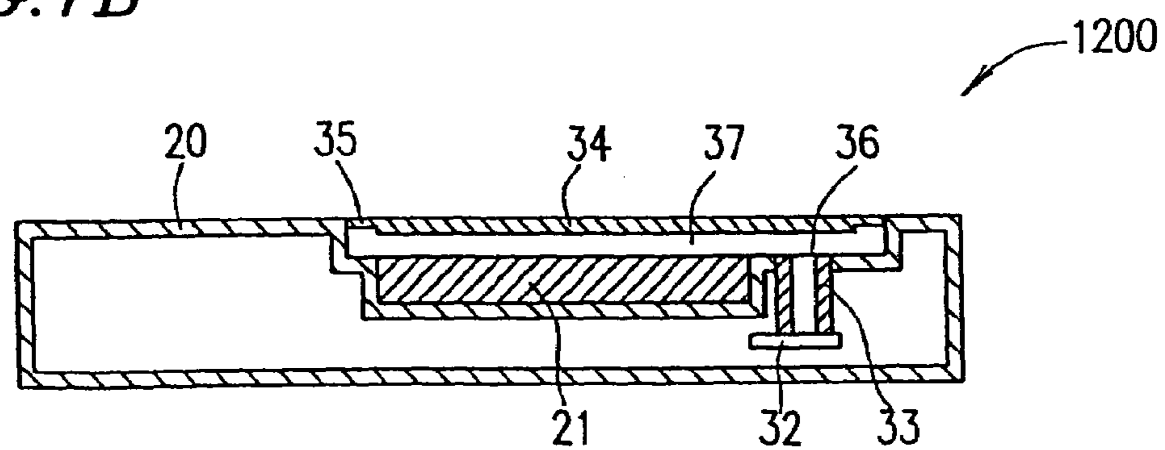
FIG. 7B
