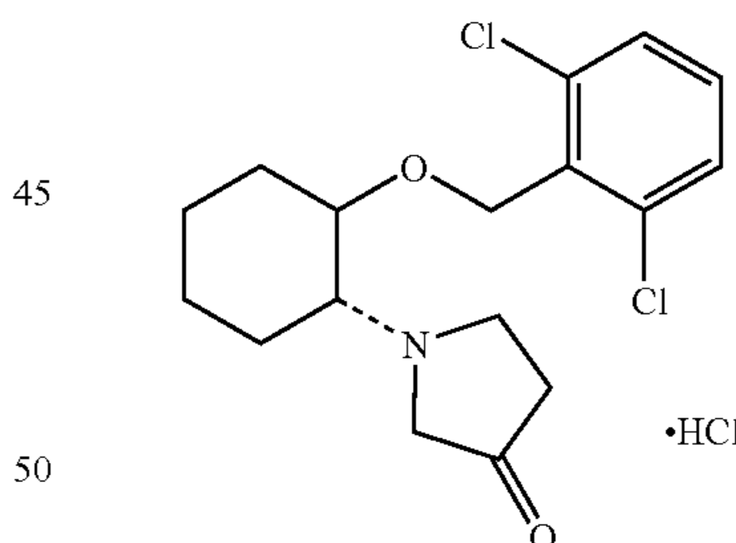
(1R,2R)/(1S,2S)-2-(3-ketopyrrolidinyl)-1-[(2,6-dichlorophenyl)methoxy]cyclohexane monohydrochloride
