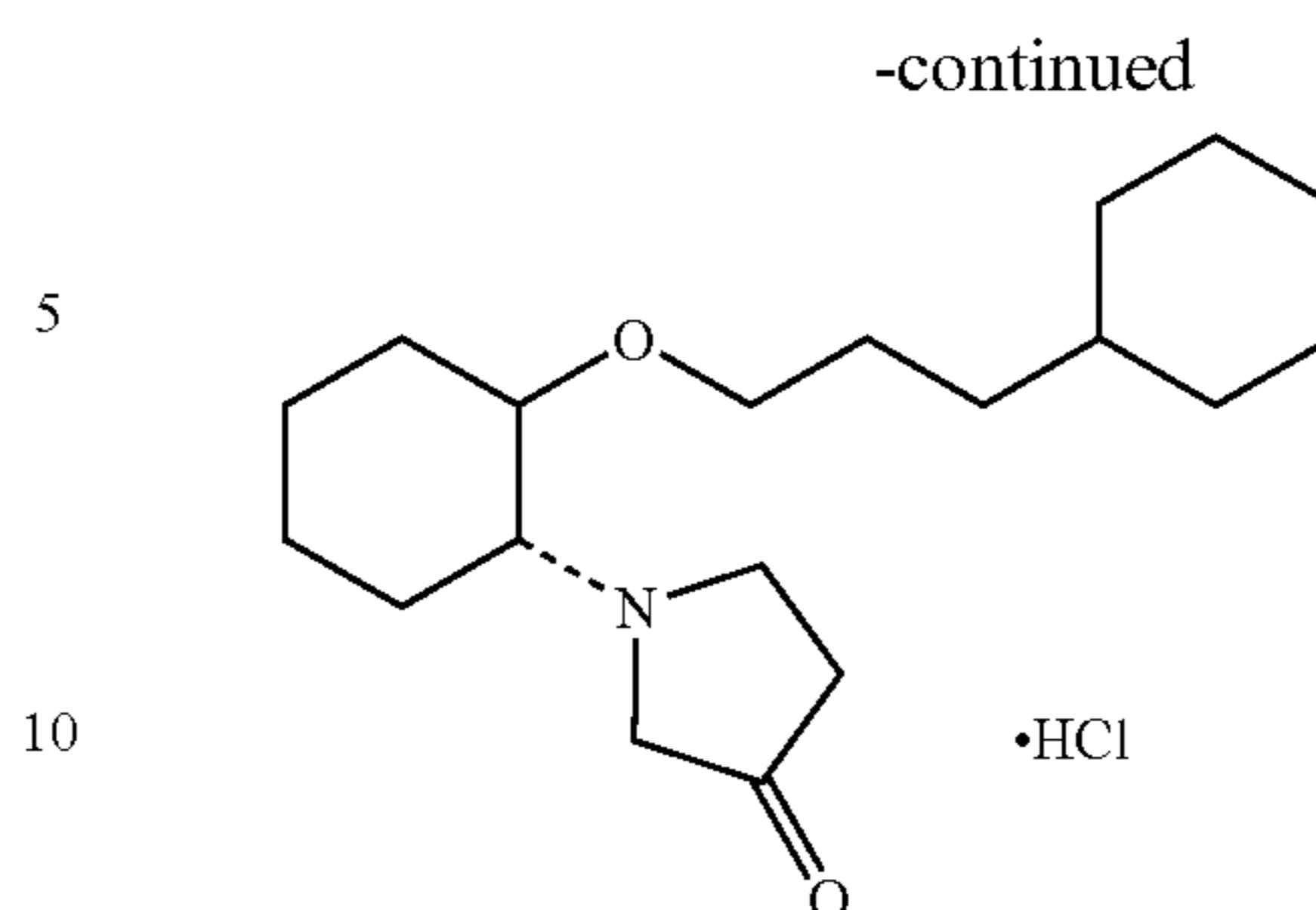
(1R,2R)/(1S,2S)-2-(3-ketopyrrolidinyl)-1-[3-(cyclohexyl)propoxy]cyclohexane monohydrochloride
