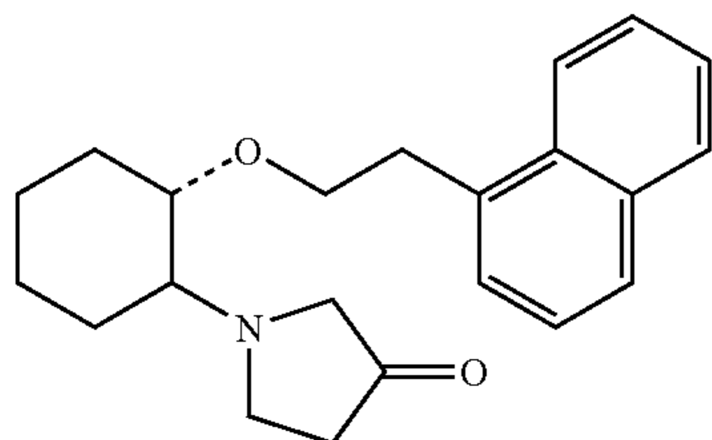
(1R,2R)/(1S,2S)-2-(3-ketopyrrolidinyl)-1-(1-naphthenoxy)cyclohexane
