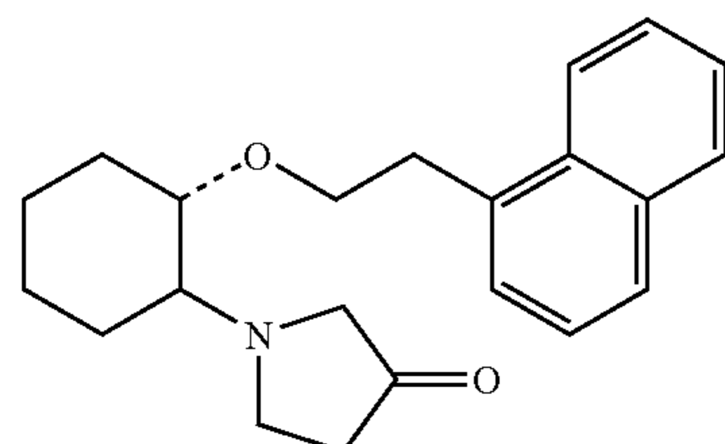
(1R,2R)/(1S,2S)-2-(3-ketopyrrolidinyl)-1-(1-naphthenoxy)cyclohexane
