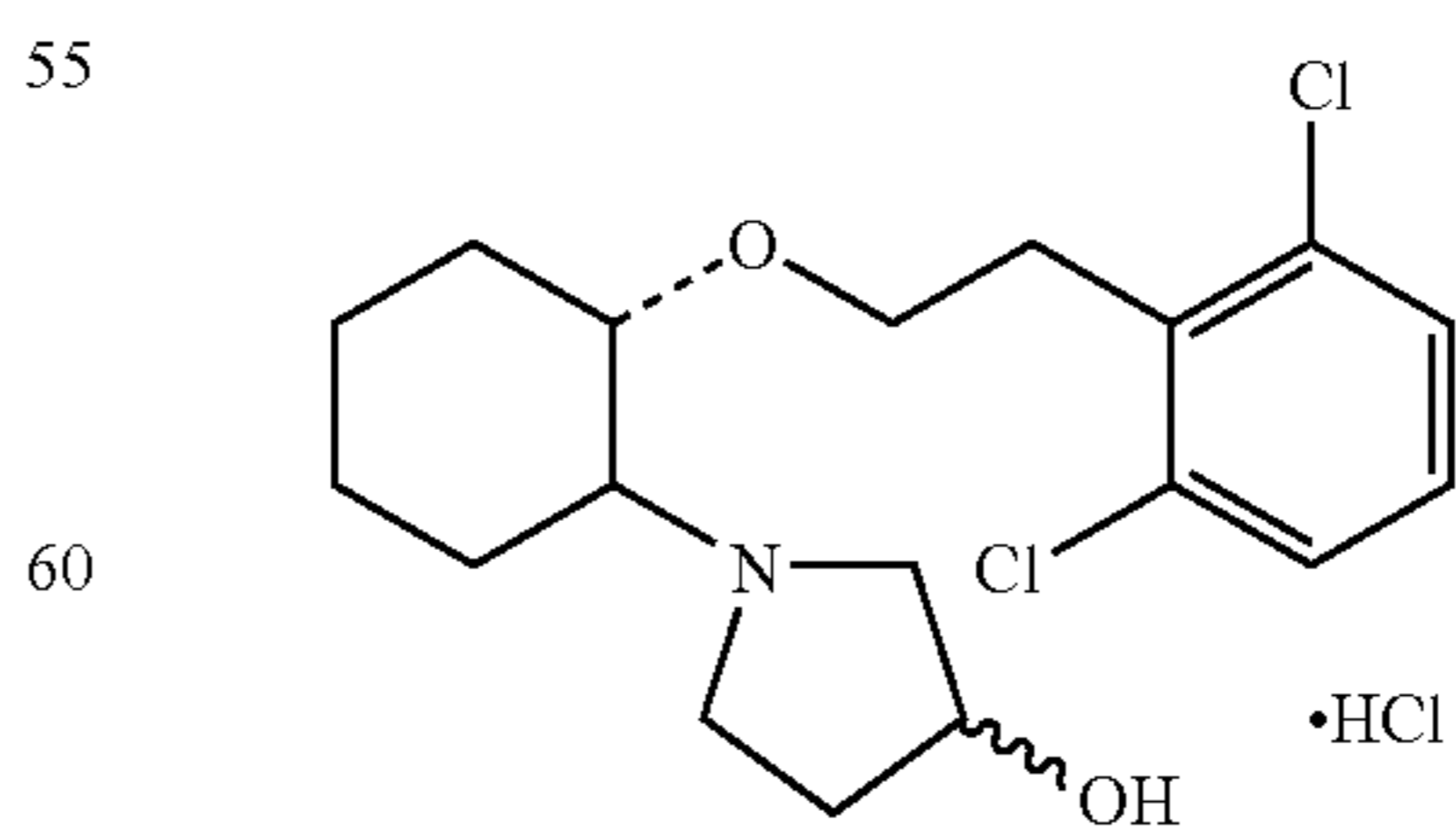
(1R,2R)/(1S,2S)-2-(3-ketopyrrolidinyl)-1-[(2,6-dichlorophenyl)methoxy]cyclohexane monohydrochloride
