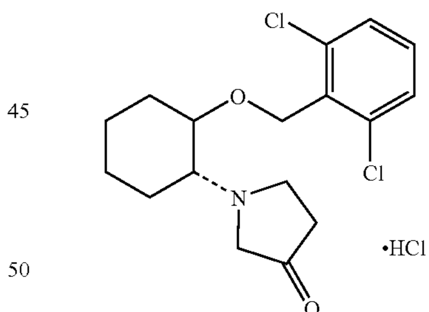
(1R,2R)/(1S,2S)-2-(3-ketopyrrolidinyl)-1-[(2,6-dichlorophenyl)methoxy]cyclohexane monohydrochloride
