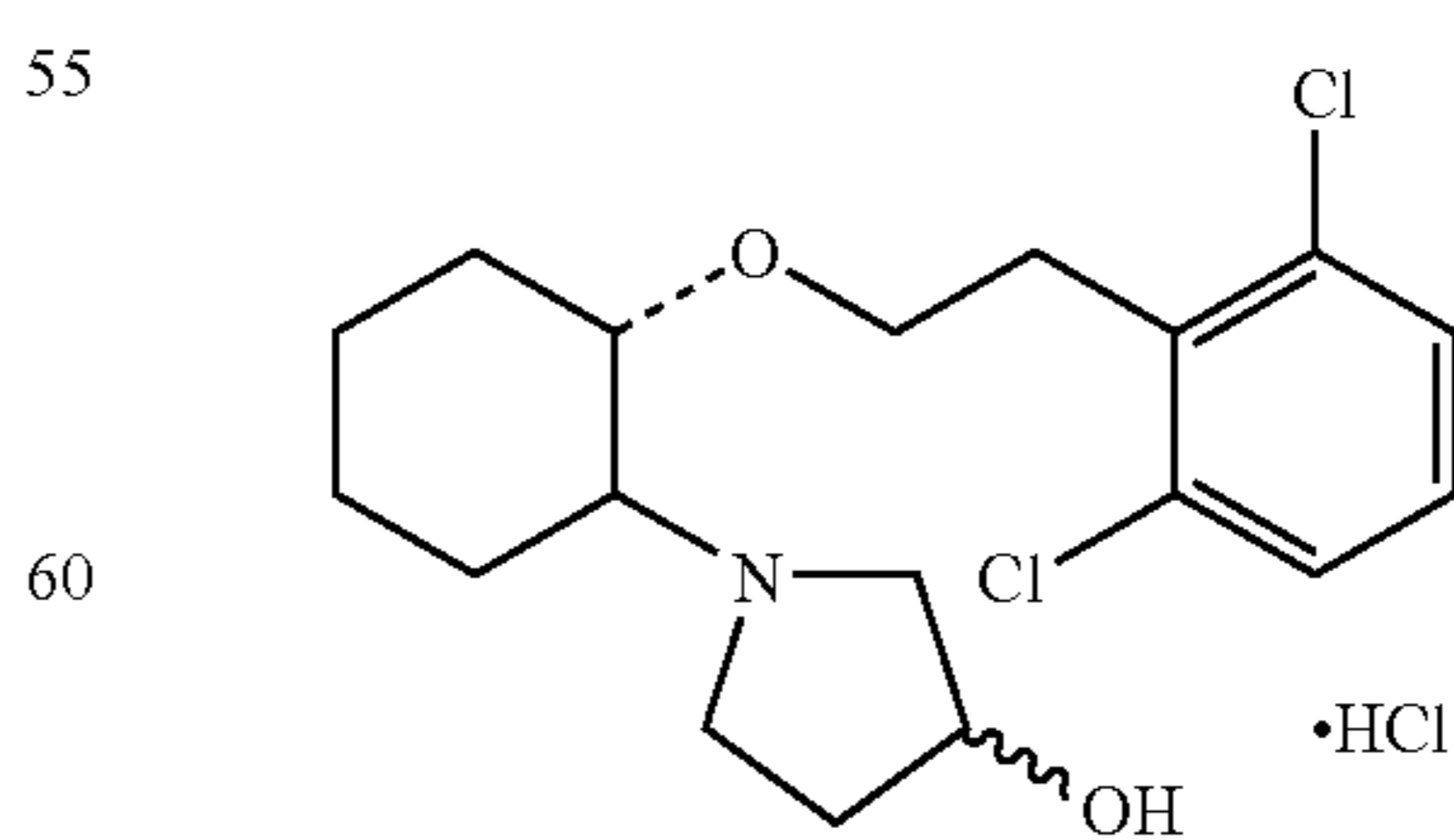
(1R,2R)/(1S,2S)-2-(3-ketopyrrolidinyl)-1-[(2,6-dichlorophenyl)methoxy]cyclohexane monohydrochloride
