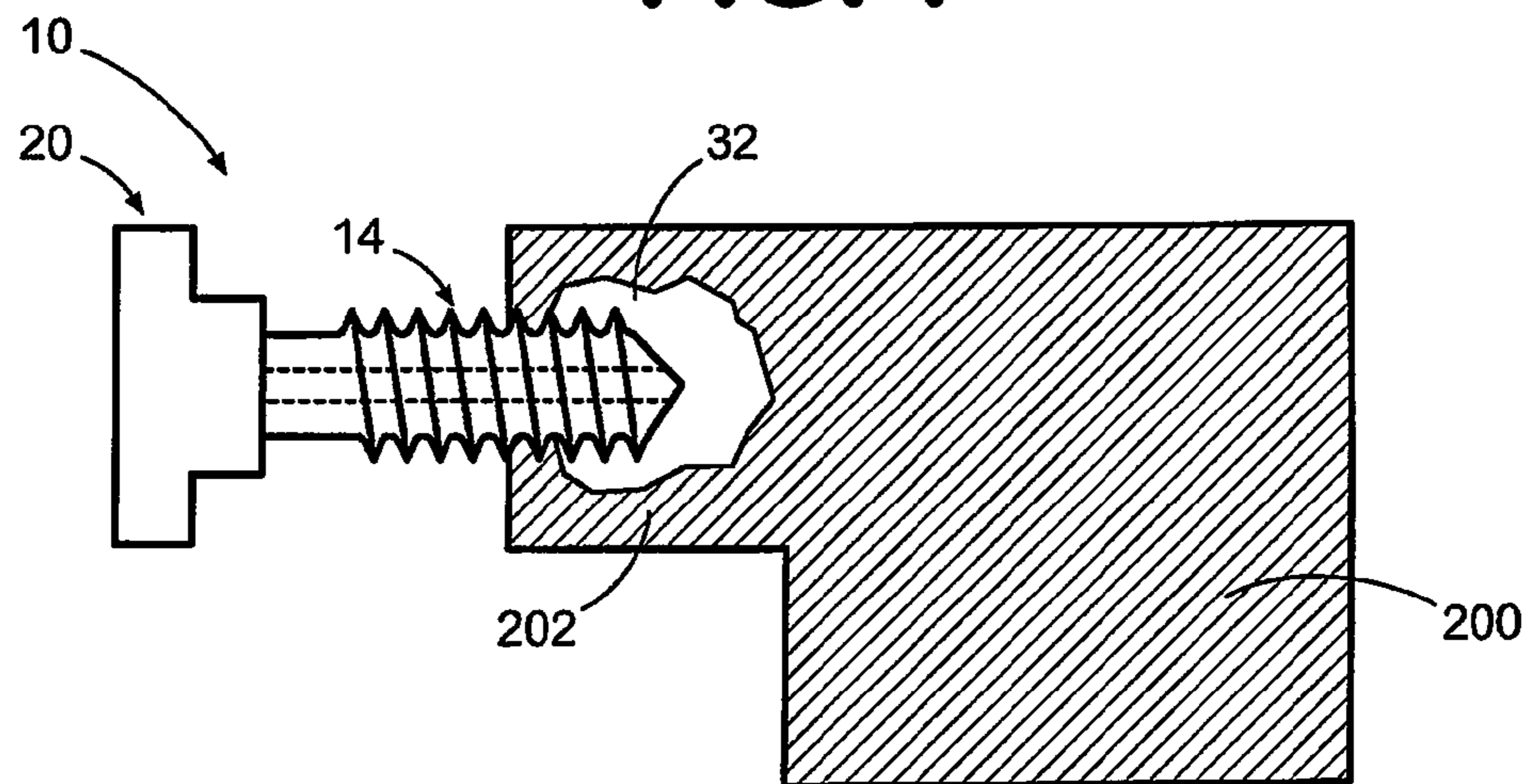
FIG. 7A
