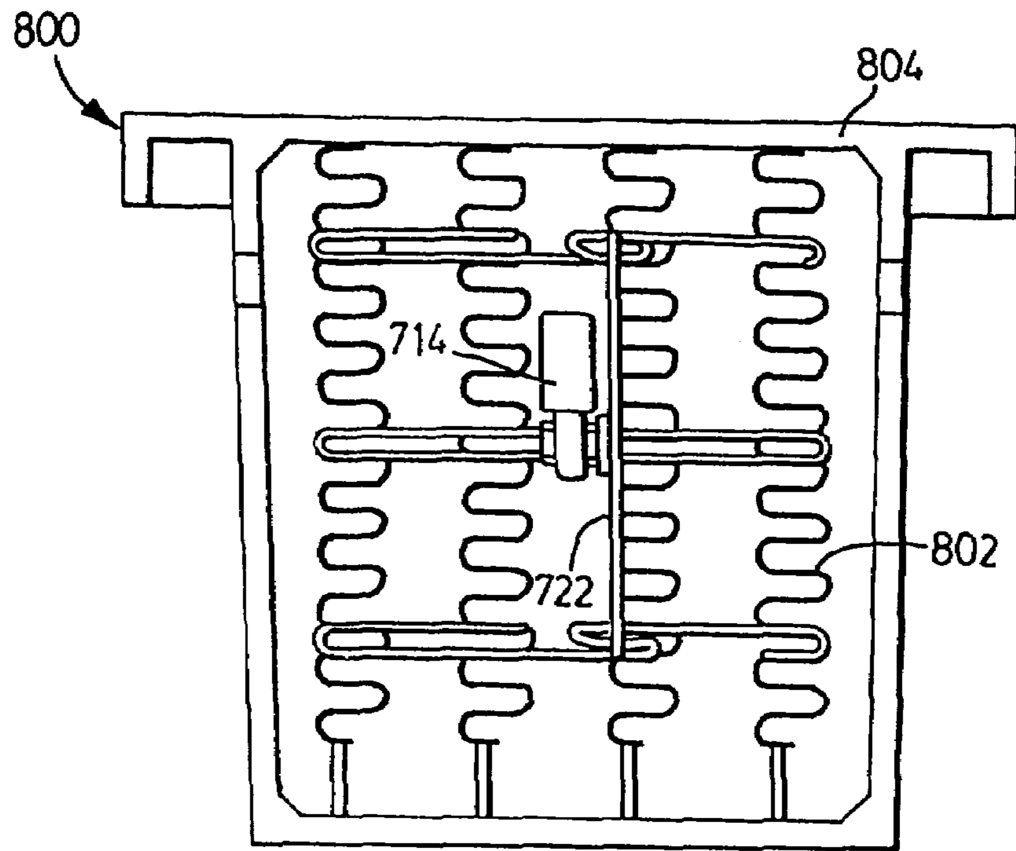
FIG. 36b
