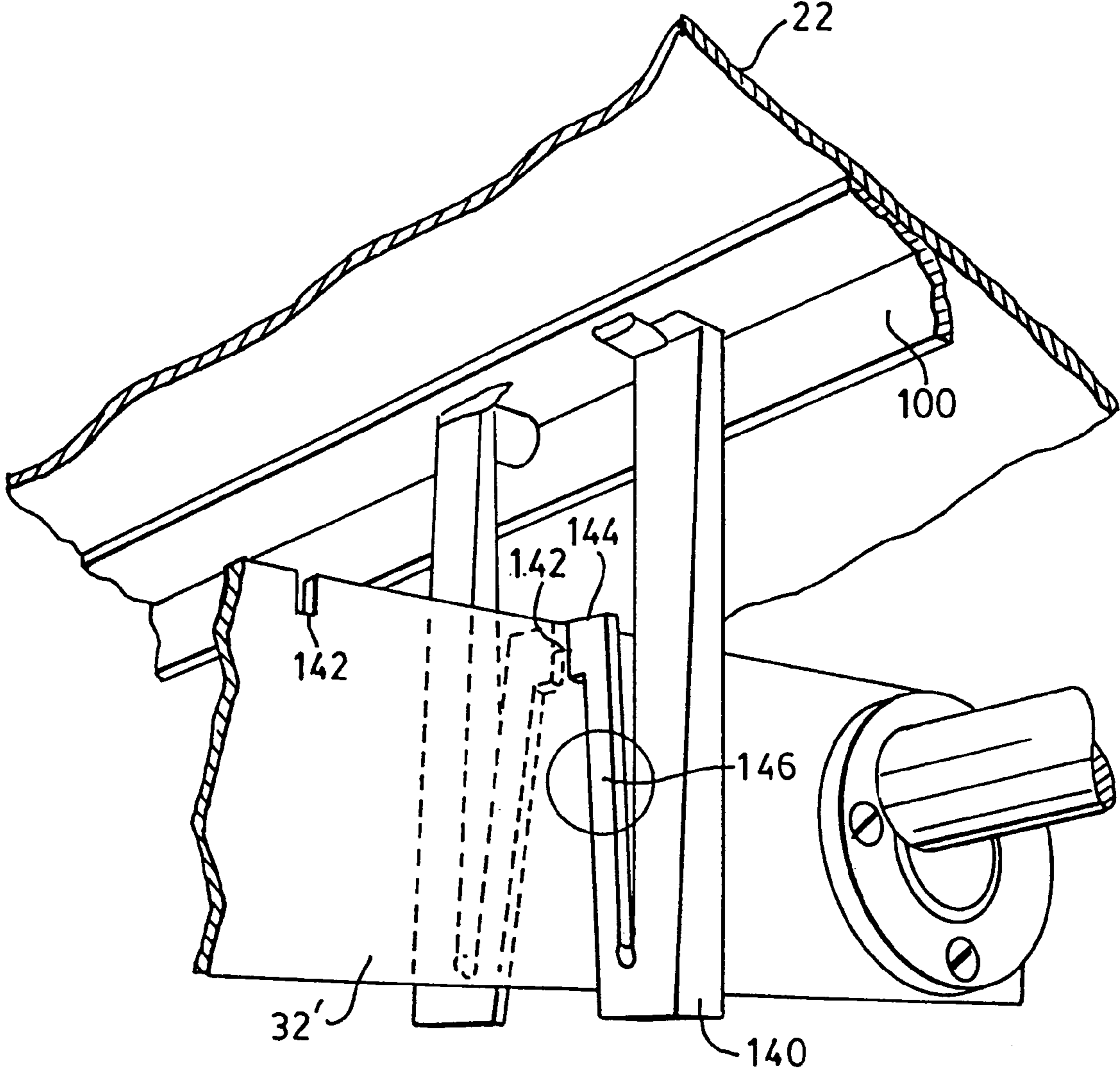
FIG. 19
