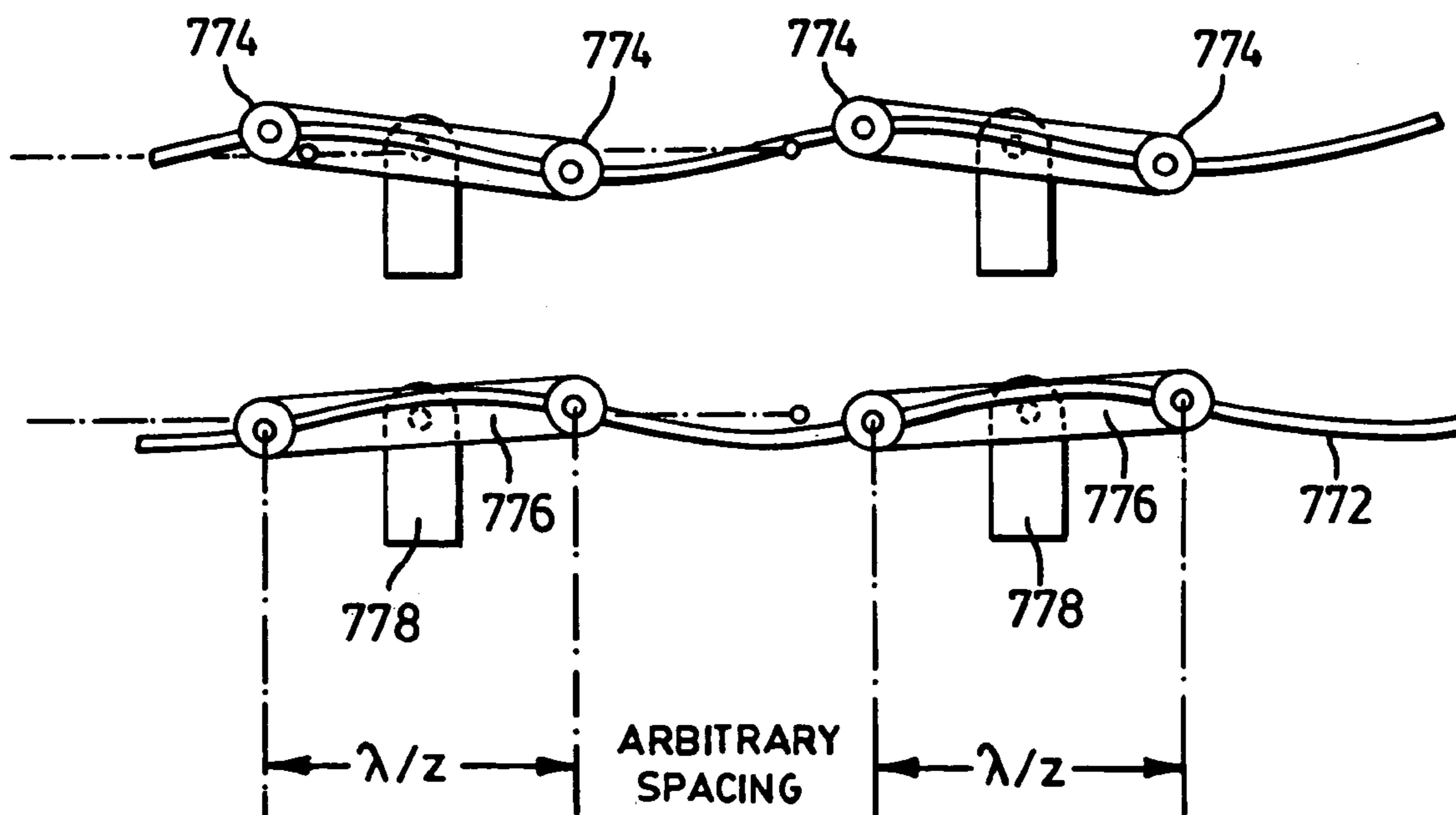
FIG. 44b
