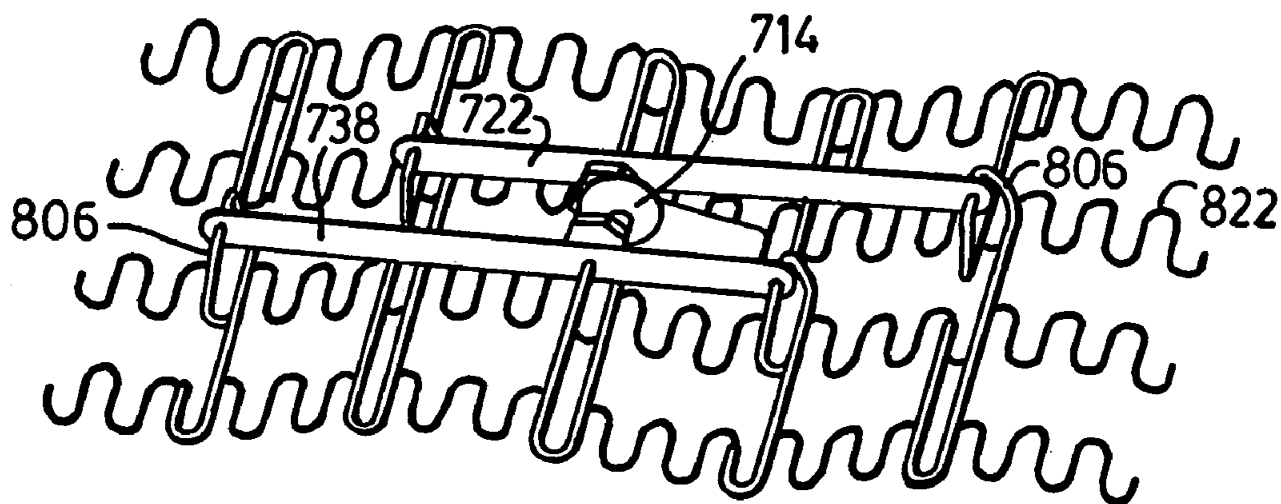
FIG. 37a
