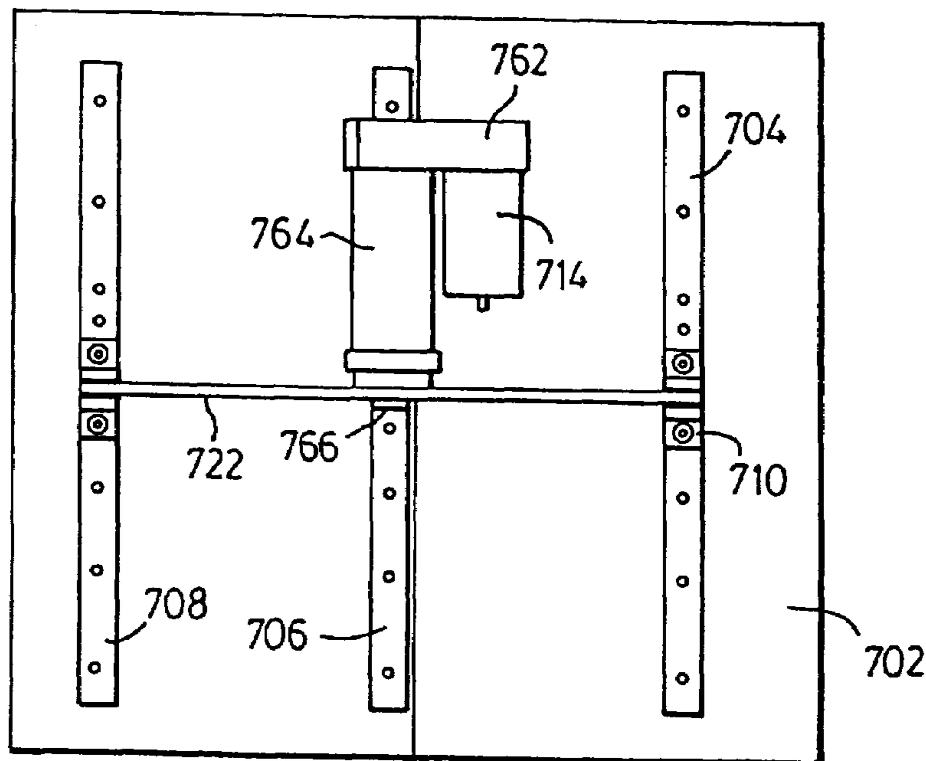
FIG. 35b
