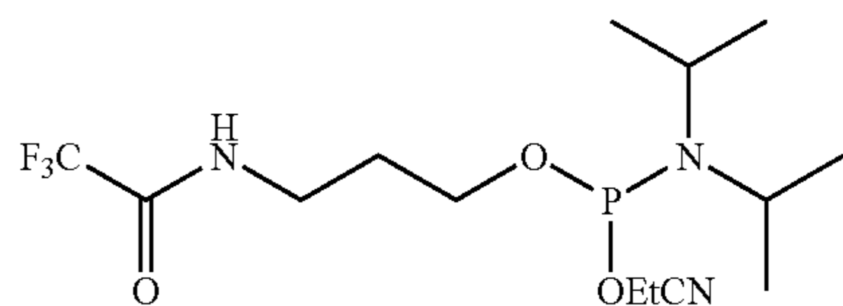
5'-Amino-Modifier C3-TFA
