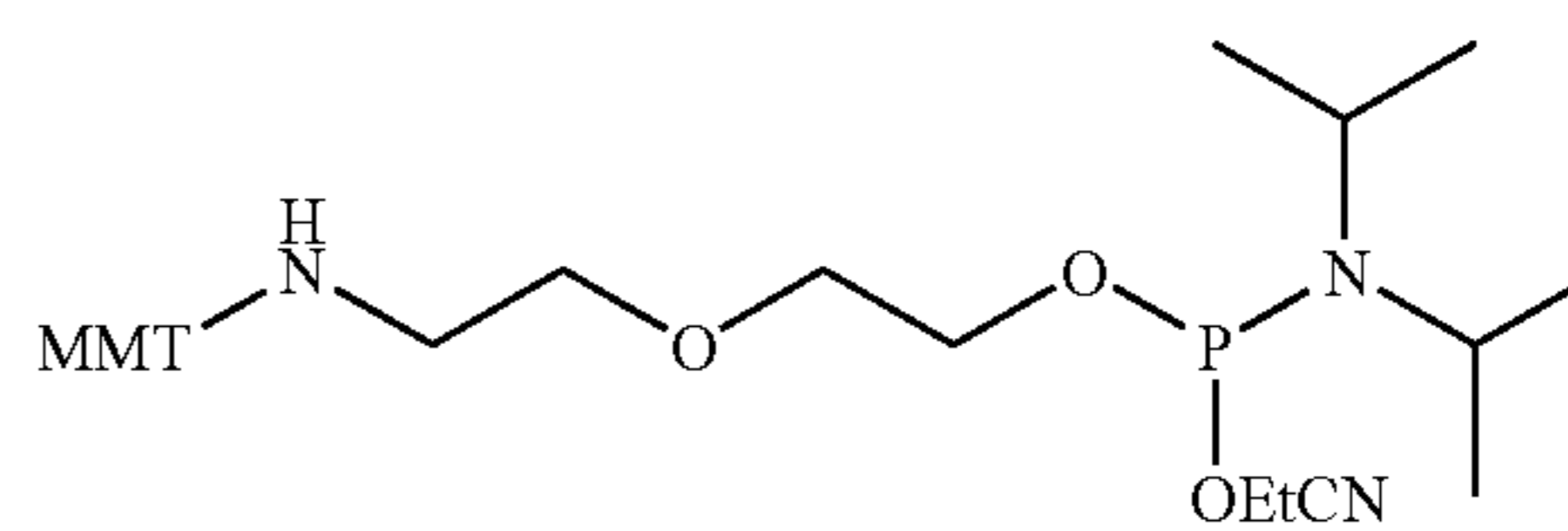
MMT:4-Monomethoxytrityl 5'-Amino-Modifier 5,
