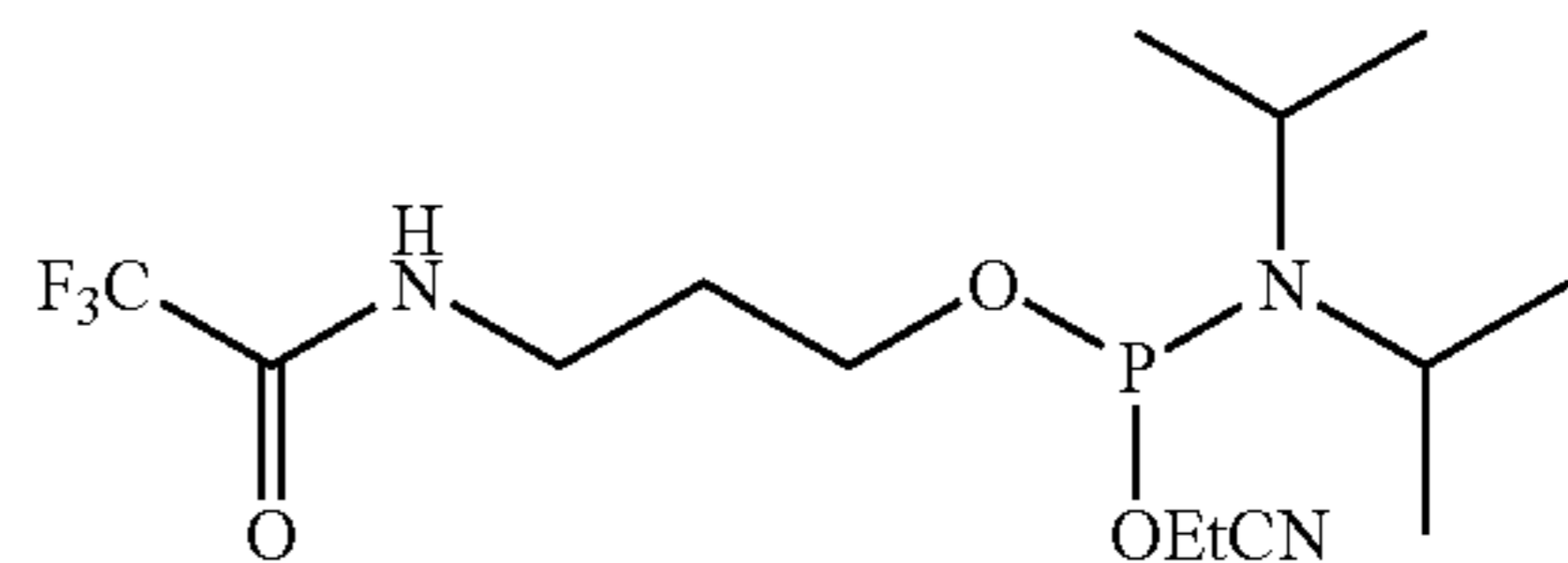
5'-Amino-Modifier C3-TFA
