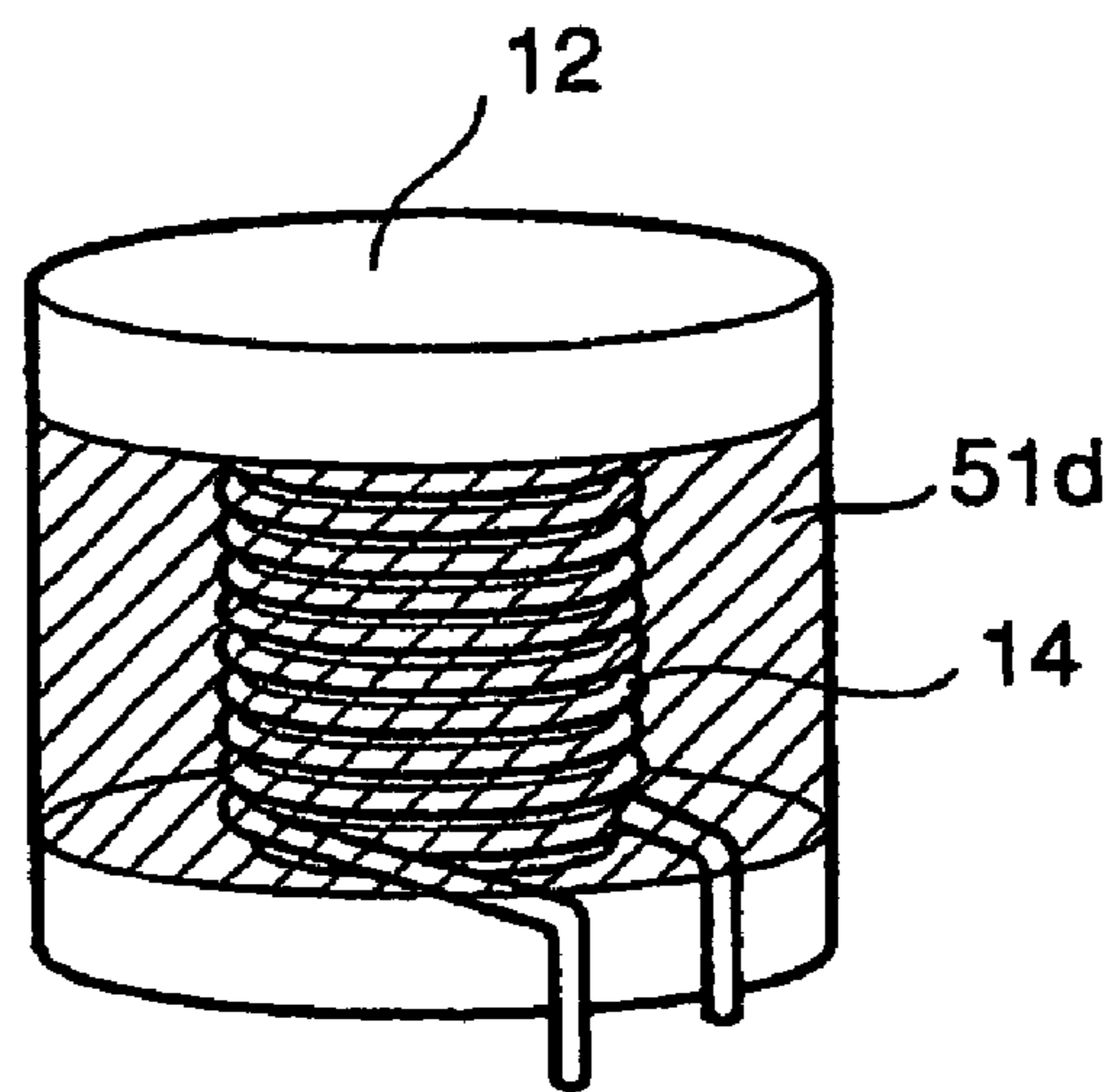
(d) OPEN MAGNETIC PATH TYPE
