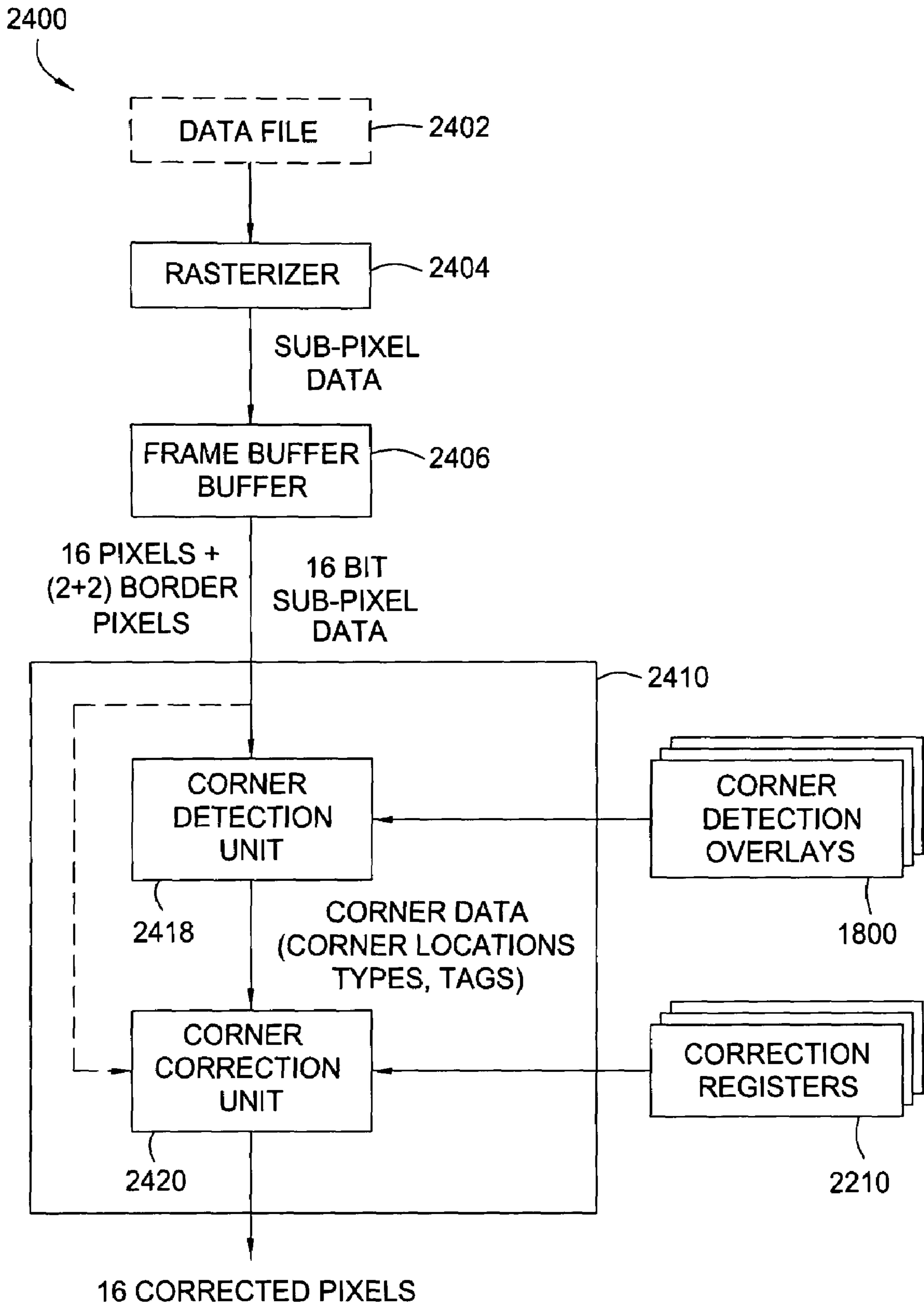
FIG. 24
