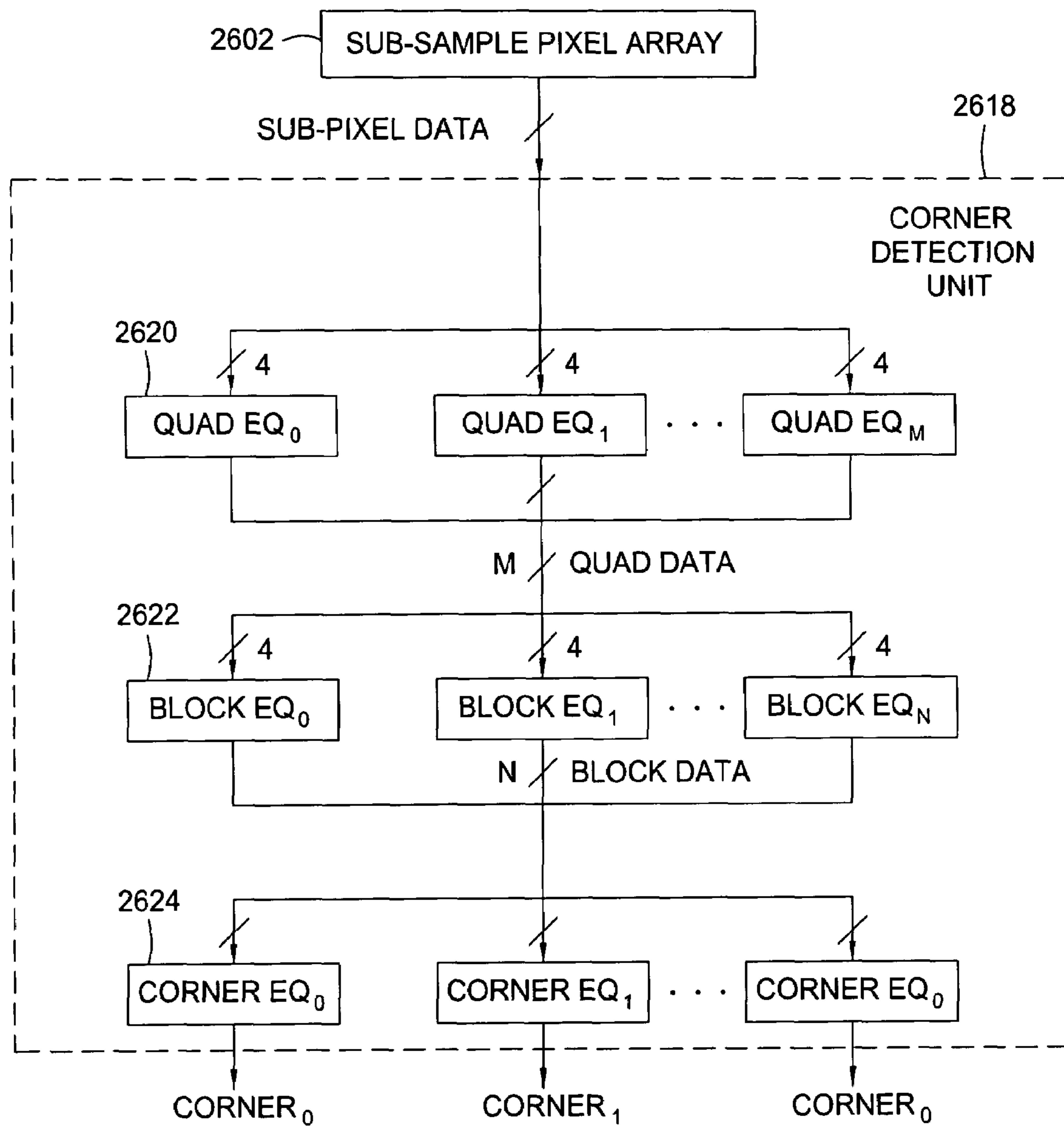
FIG. 26
