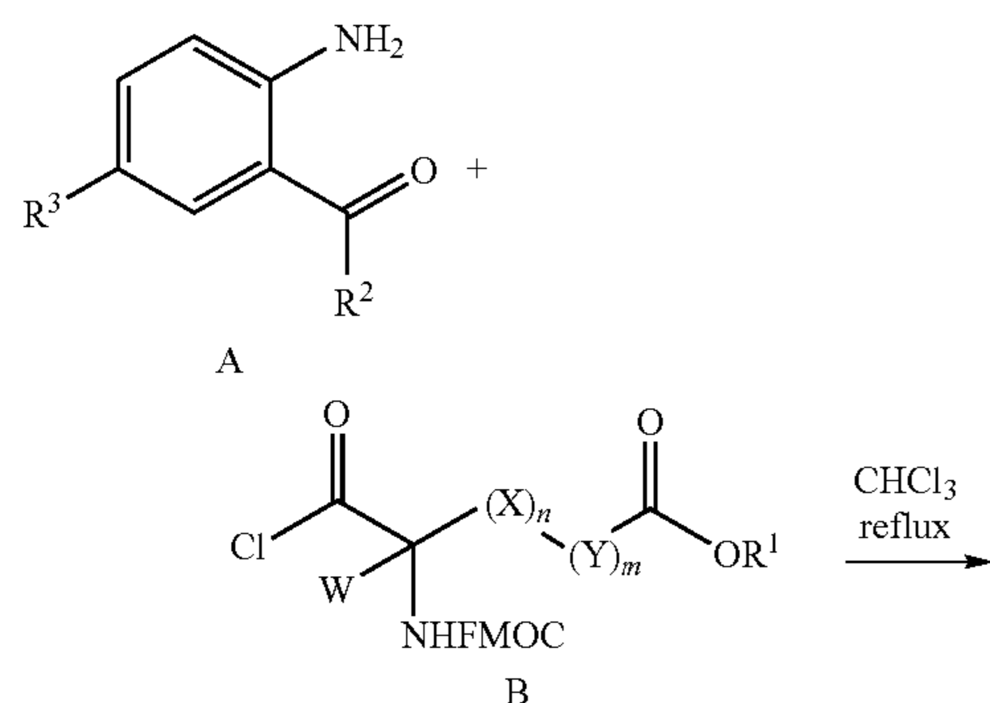
SCHEME 1a
