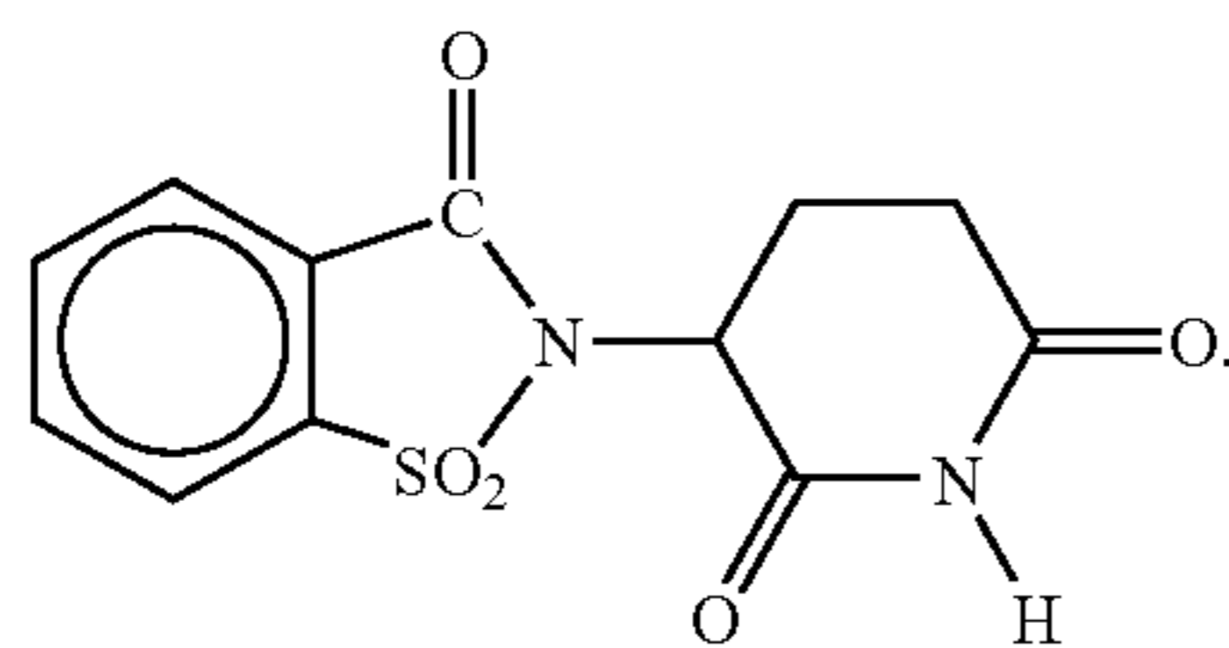
supidimide
