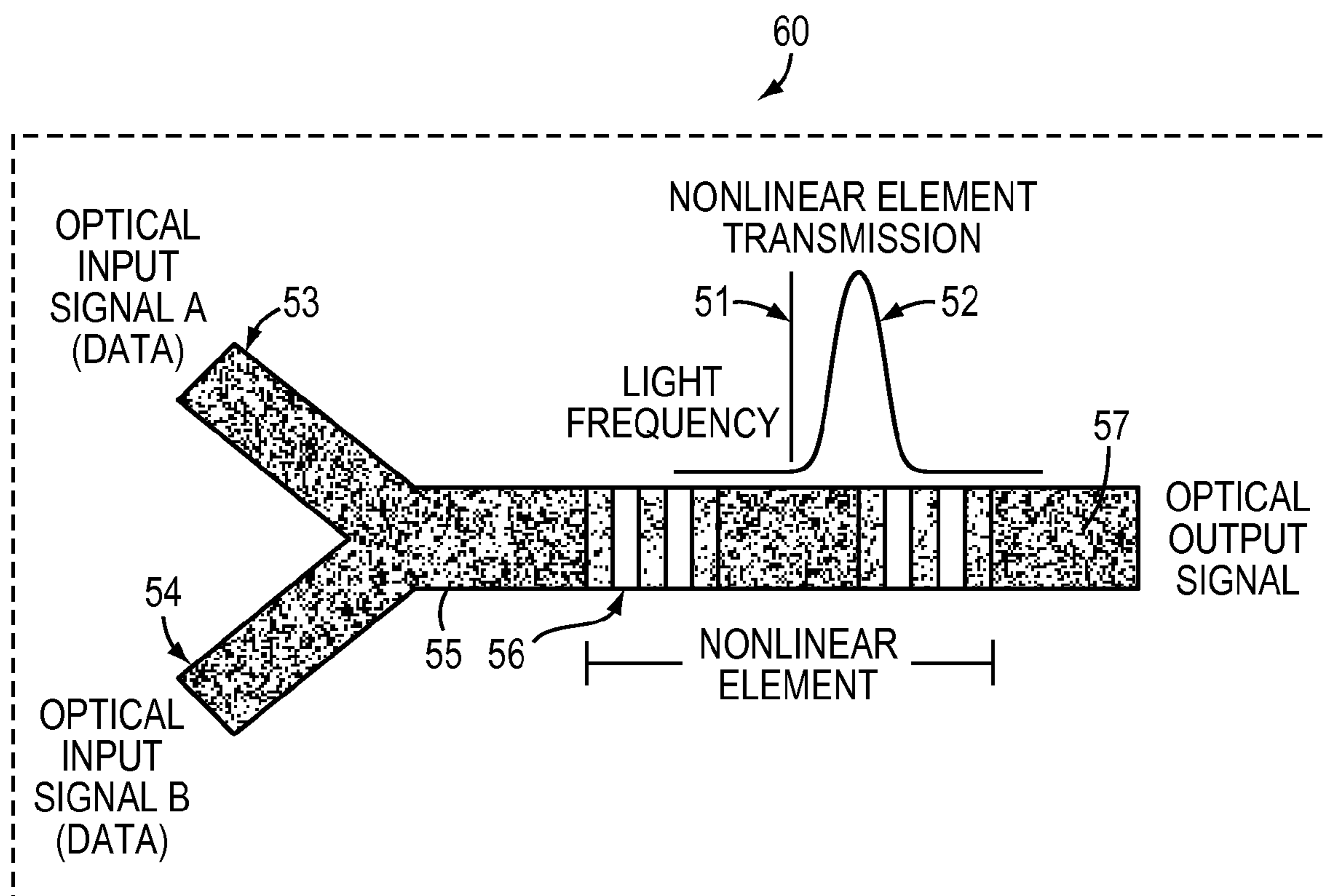
ALL-OPTICAL XOR GATE
