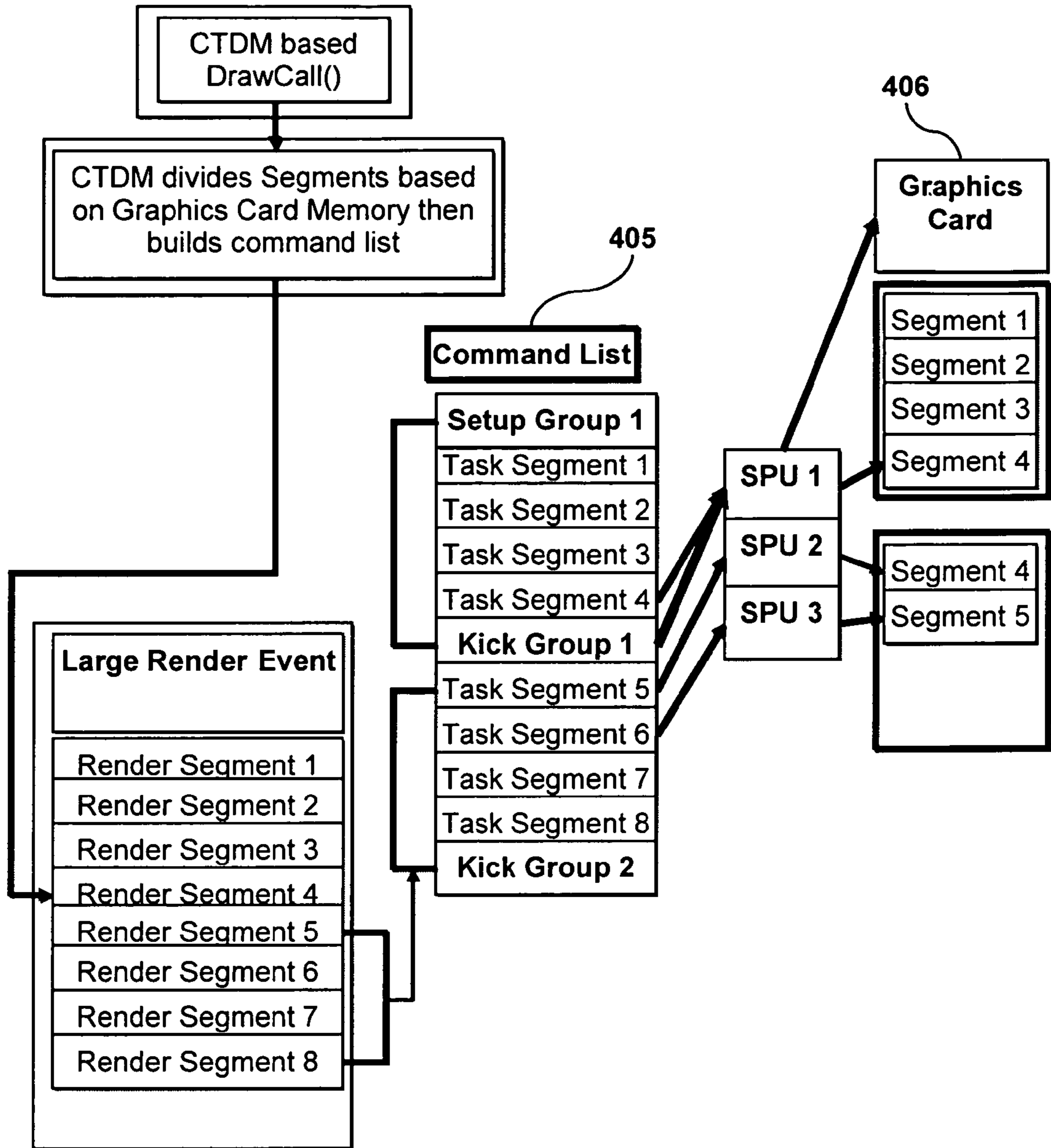
FIG. 4B
