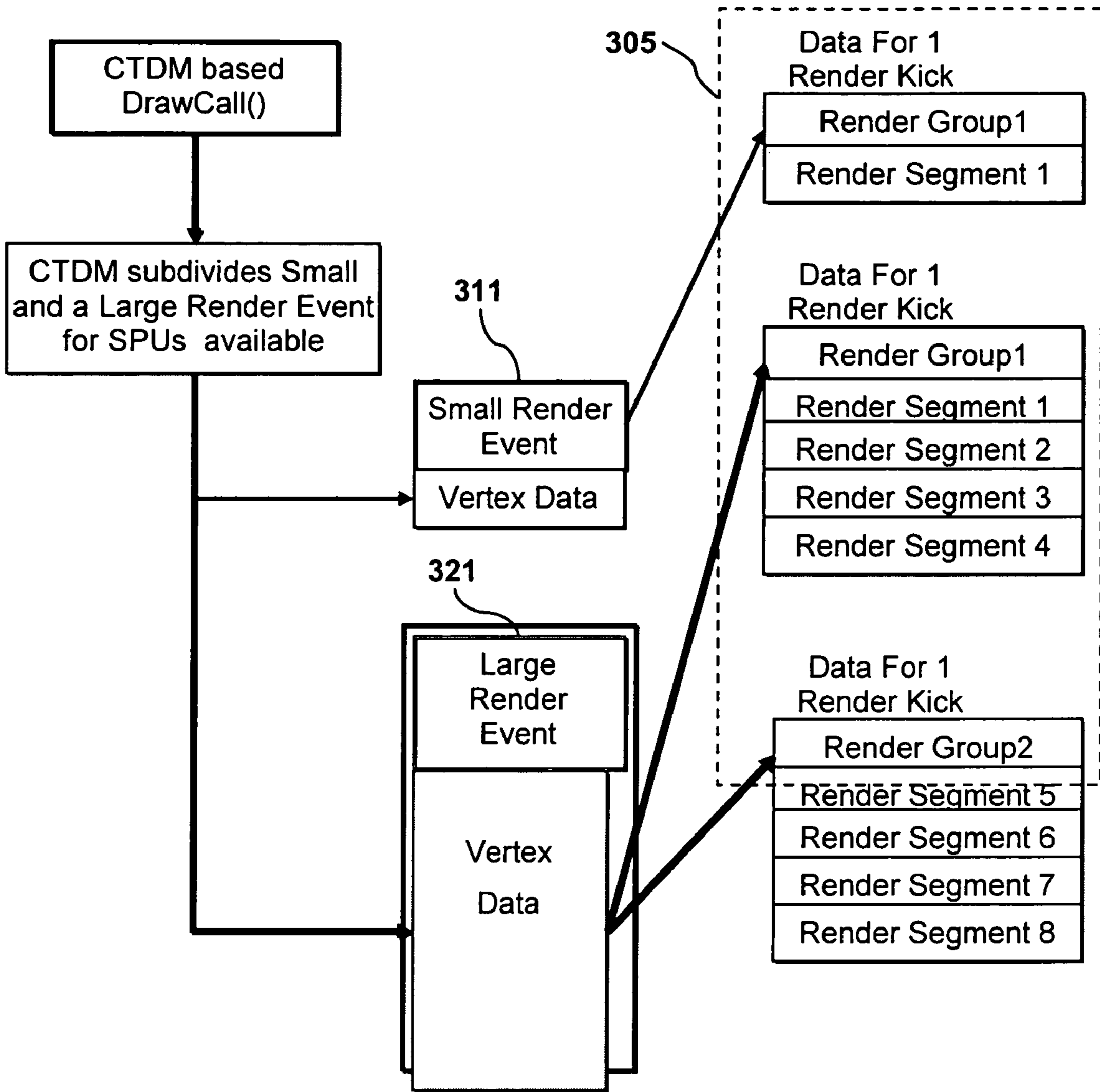
FIG. 3B
