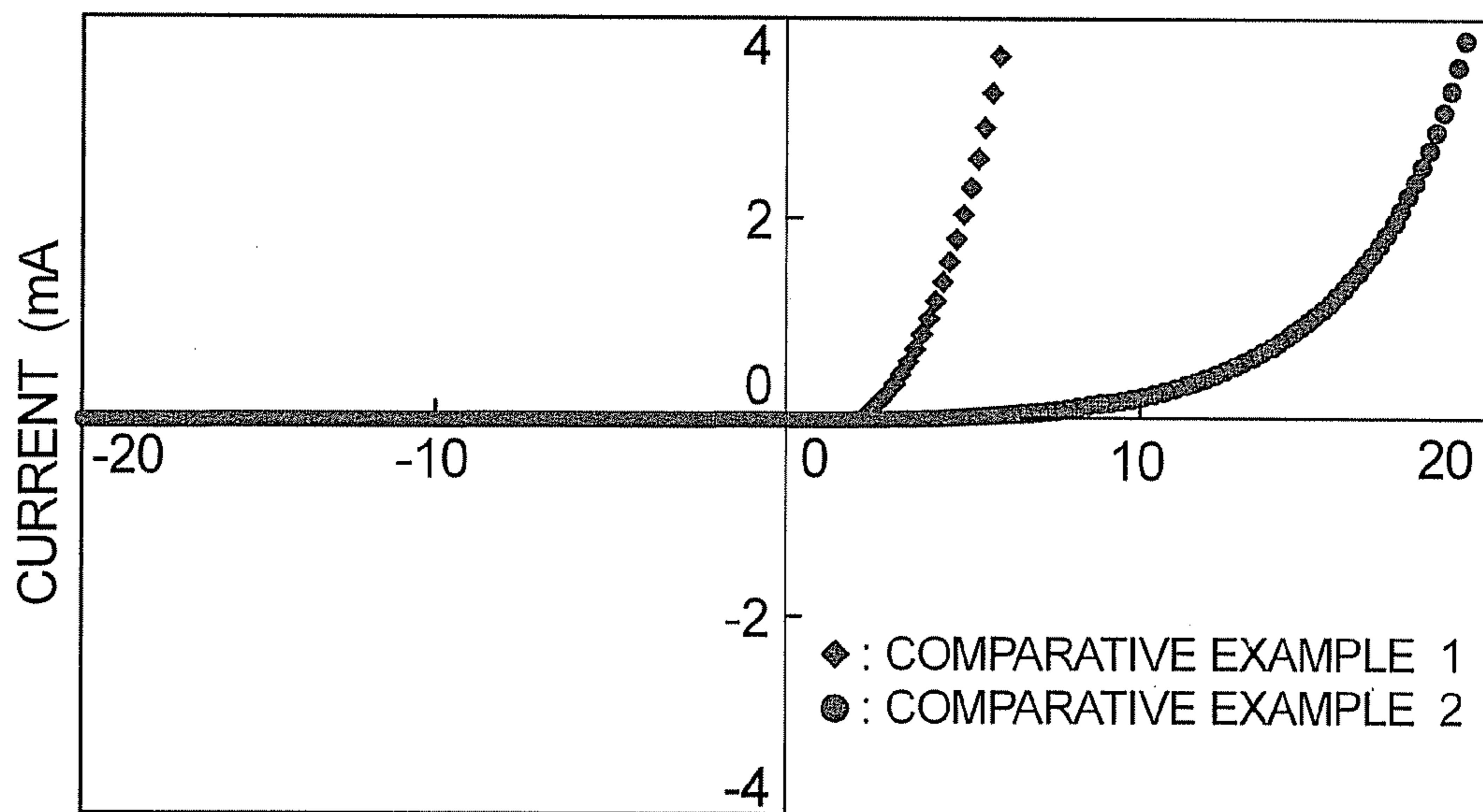
VOLTAGE (V) FIG. 14A
