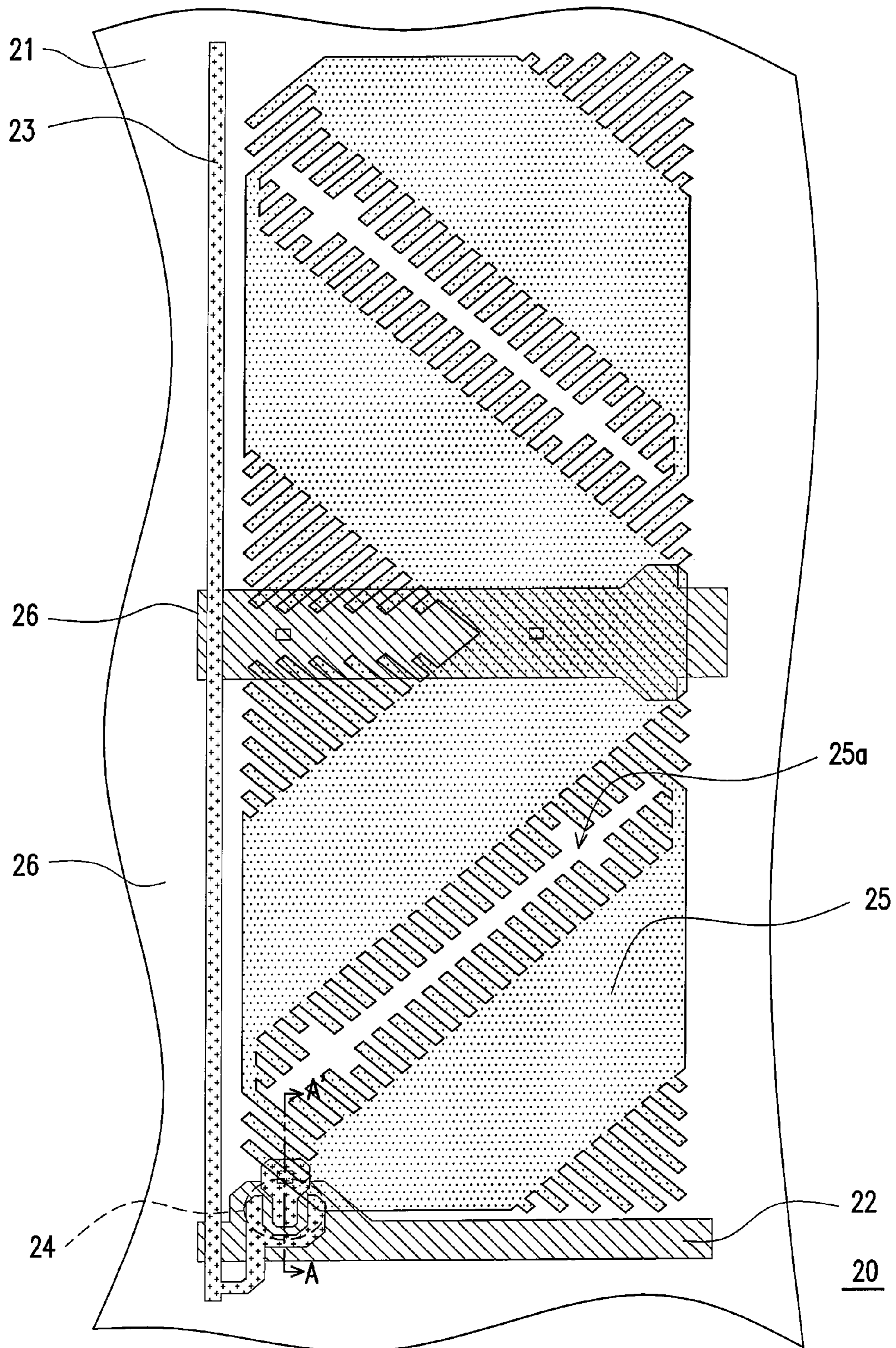
FIG. 1B(PRIOR ART)
