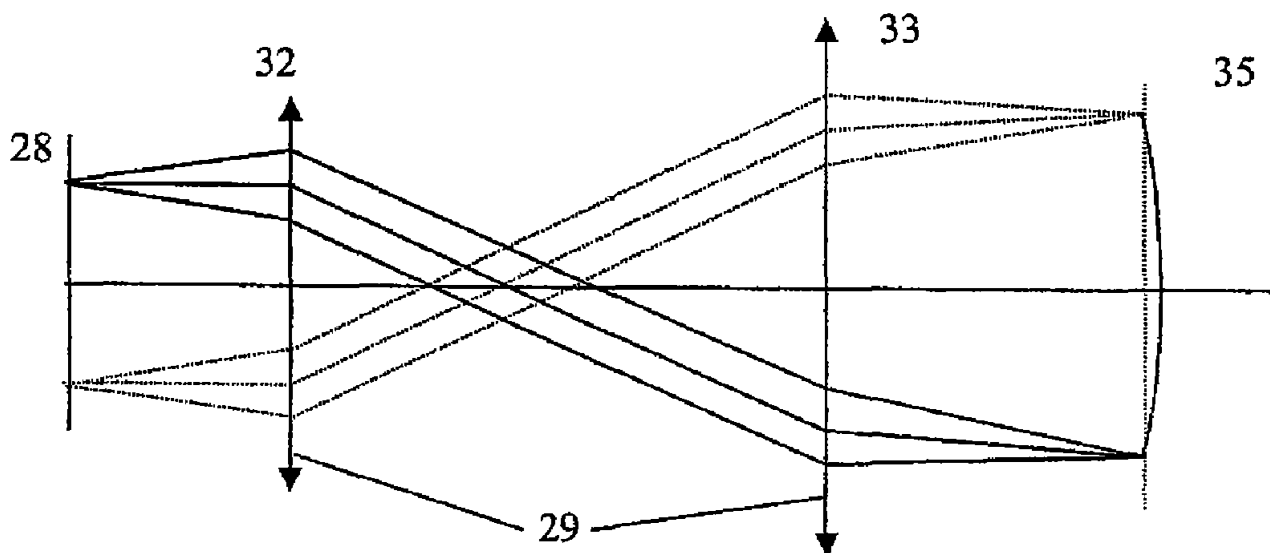
Fig. 10 -- Prior Art --
