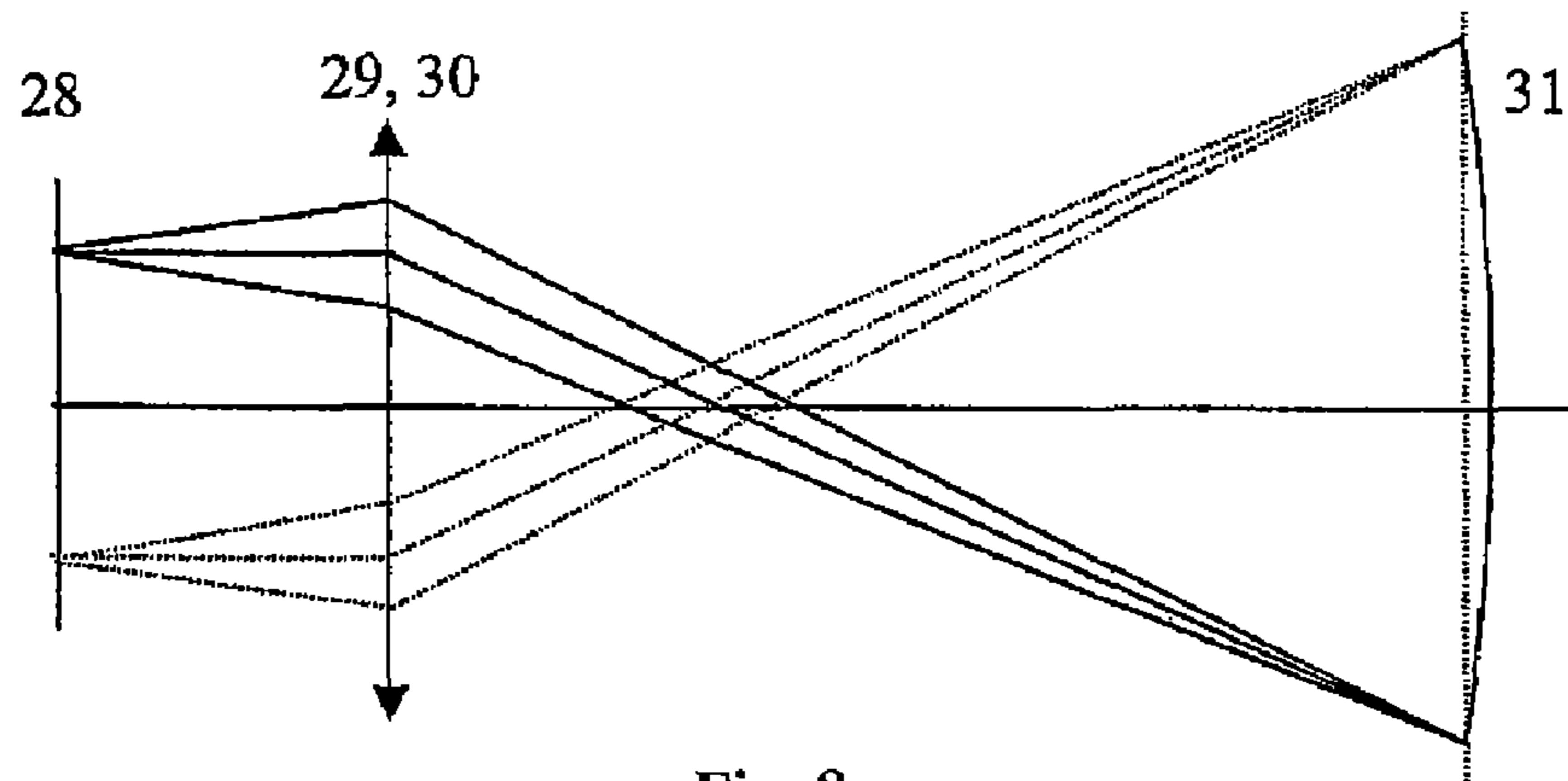
Fig. 8 -- Prior Art --
