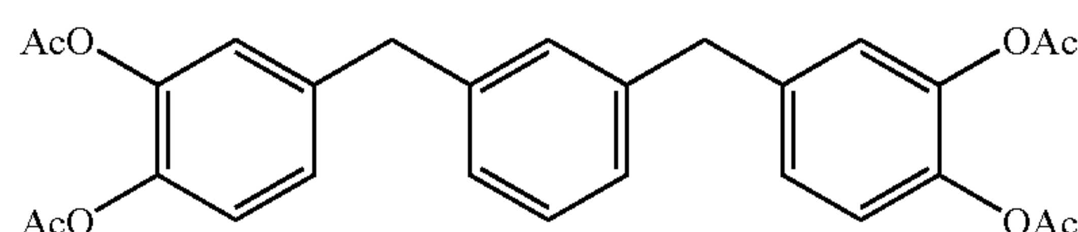
1,3-bis(3,4-diacetoxybenzyl)-benzene
