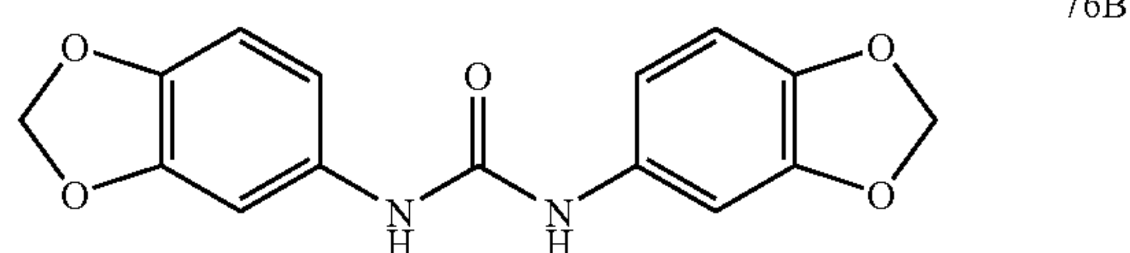
1,3-bis-(3,4-methylenedioxyphenyl)-urea
