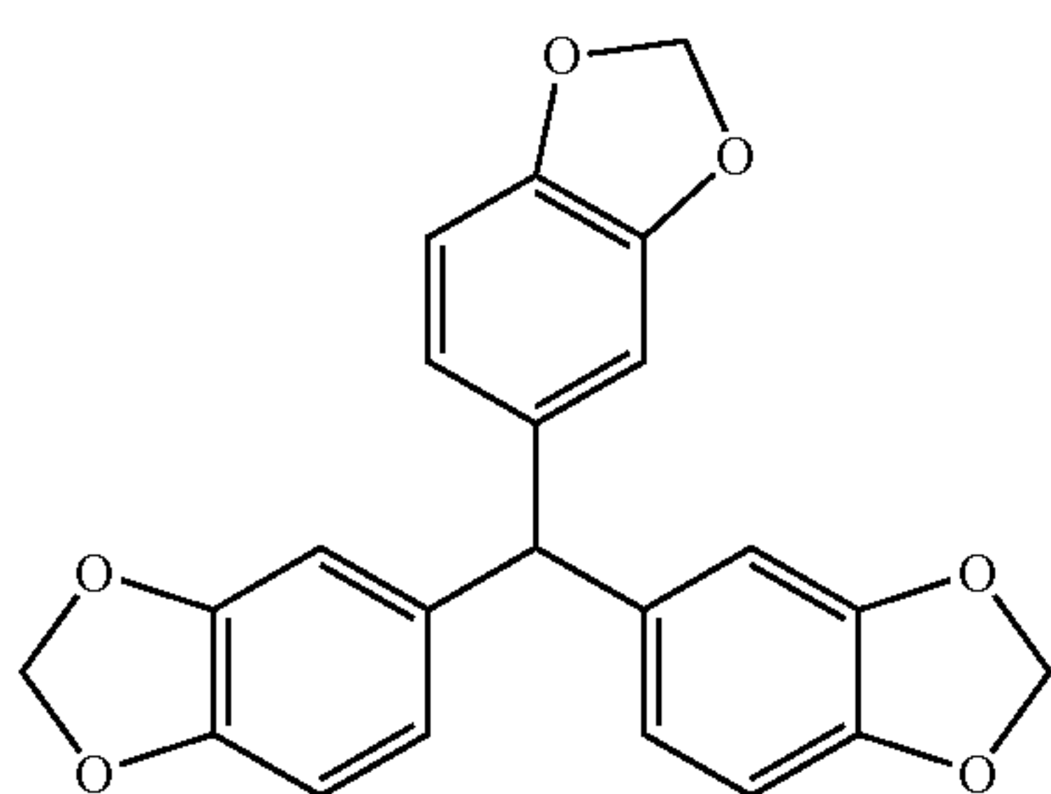
Tris-(3,4-methylenedioxyphenyl)methane
