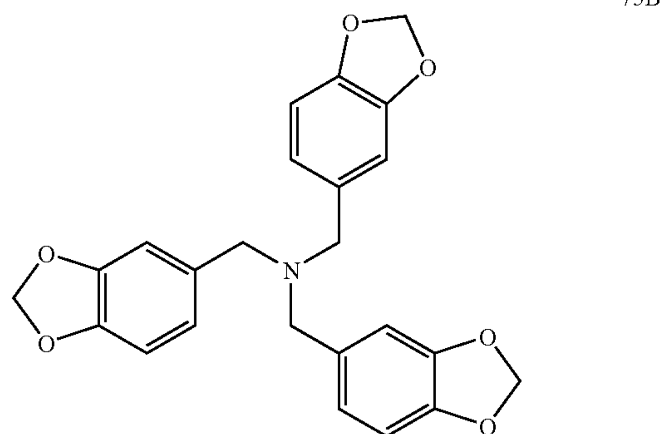
tris-(3,4-methylenedioxybenzyl)-amine
