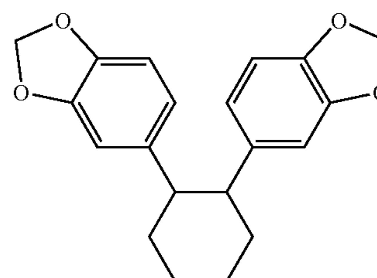
1,2-bis(3,4-methylenedioxyphenyl)-cyclohexane
