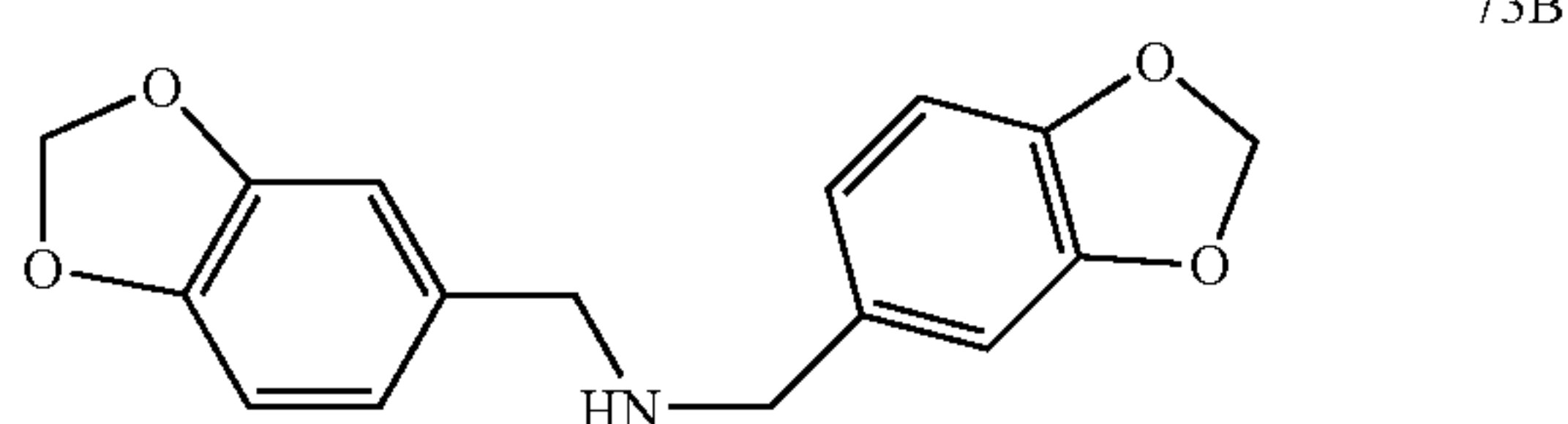
bis-(3,4-methylenedioxybenzyl)-amine
