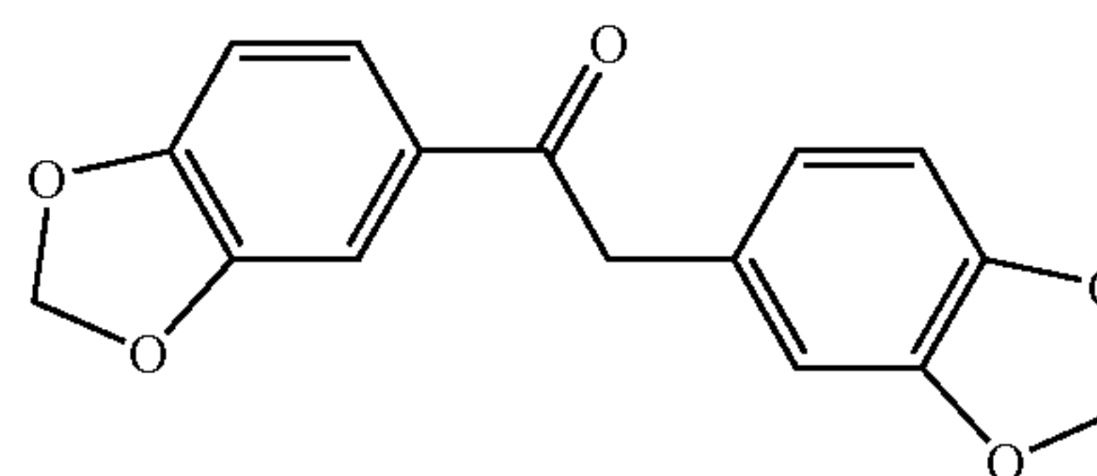
bis(3,4-methylenedioxy)desoxybenzoin
