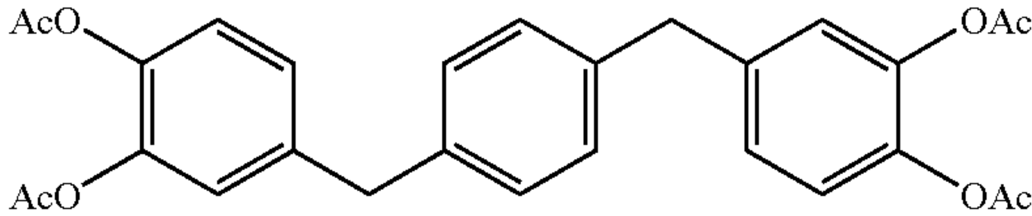
1,4-bis(3,4-diacetoxybenzyl)-benzene
