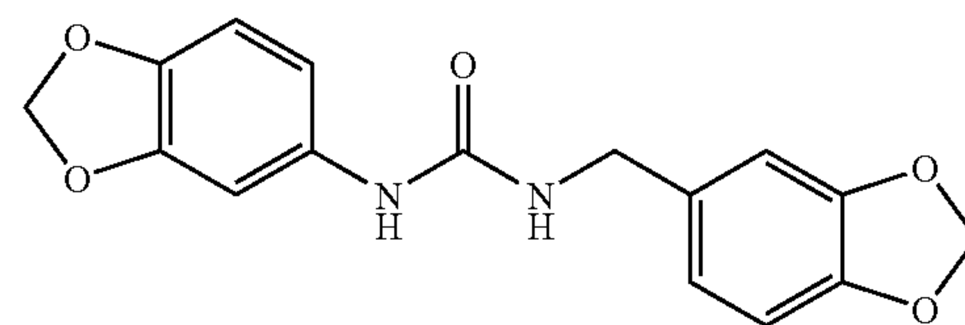
1-(3,4-methylenedioxyphenyl)-3-(3,4-methylenedioxybenzyl) urea
