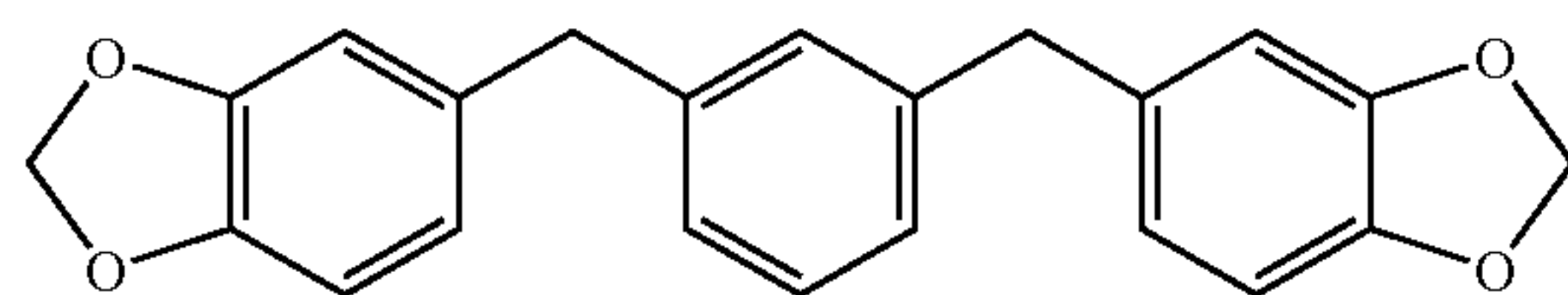
1,3-bis(3,4-methylenedioxybenzyl)-benzene
