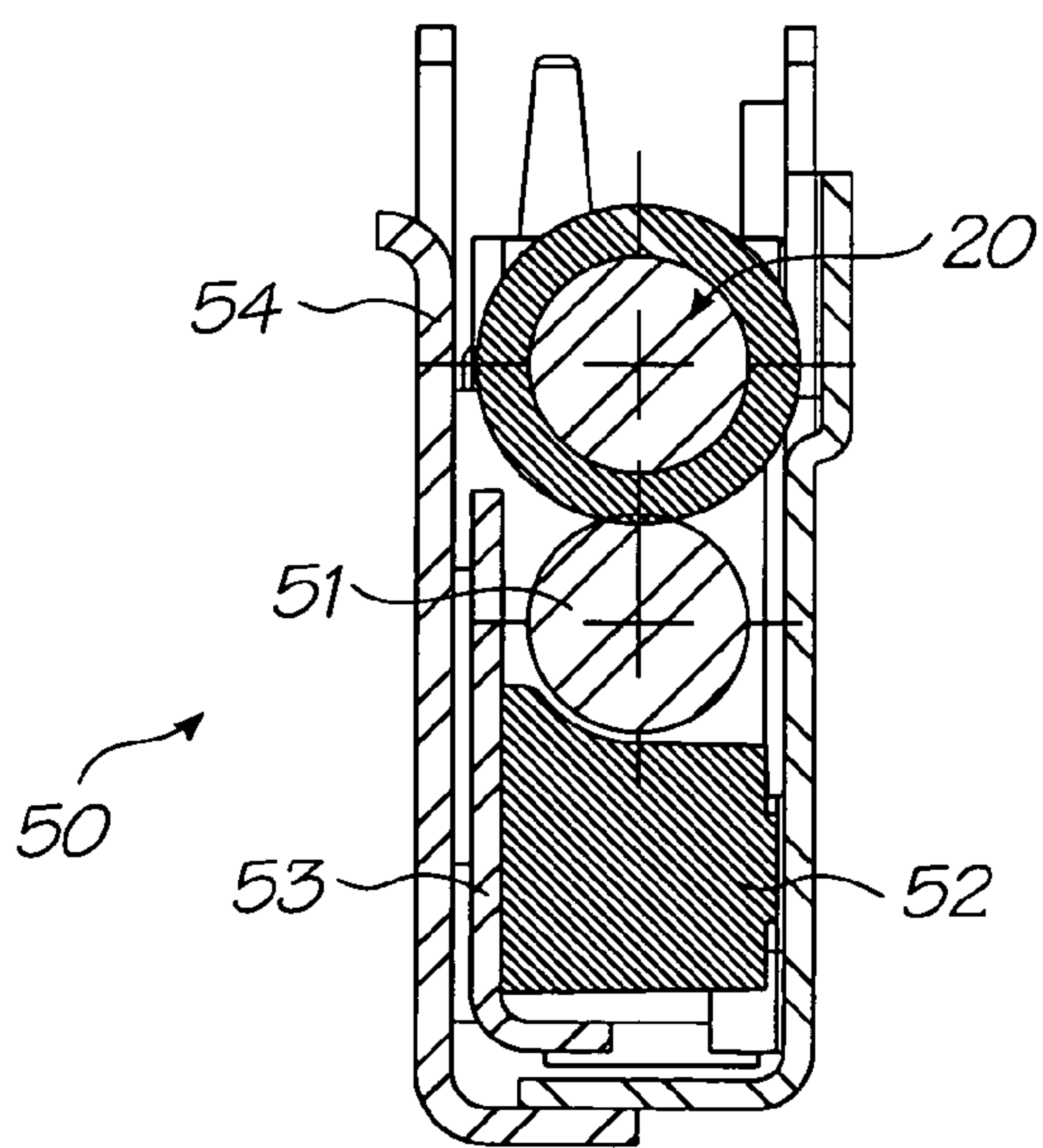
Section A-A
