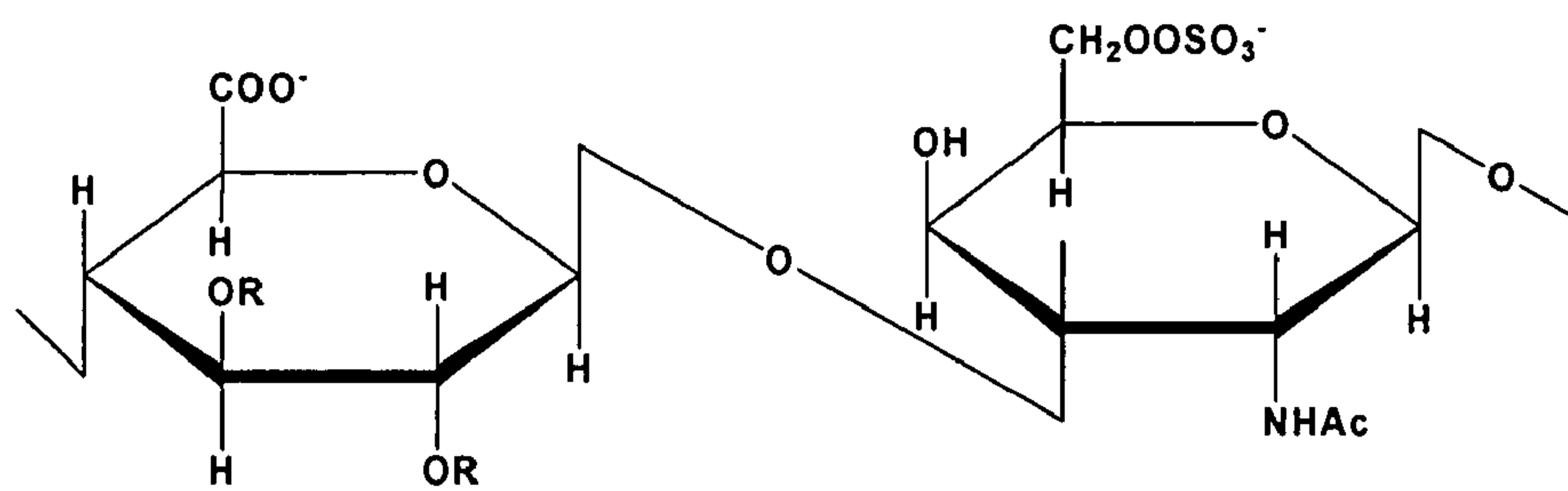
Chondroitin 6-Sulfate
