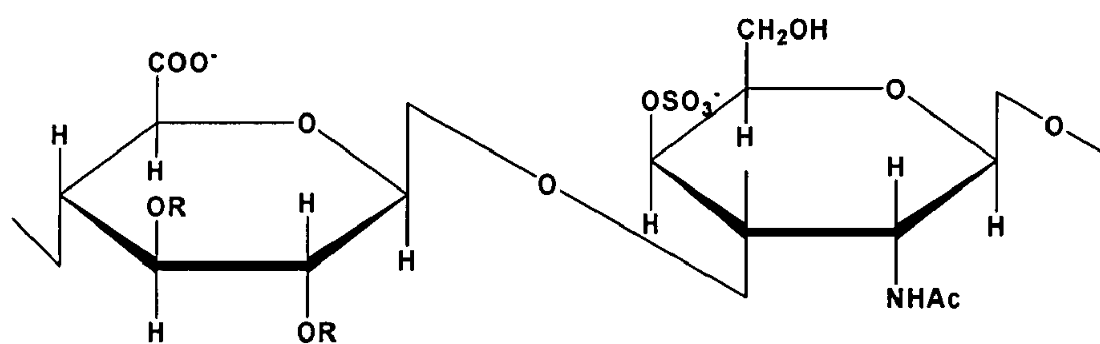
Chondroitin 4-Sulfate
