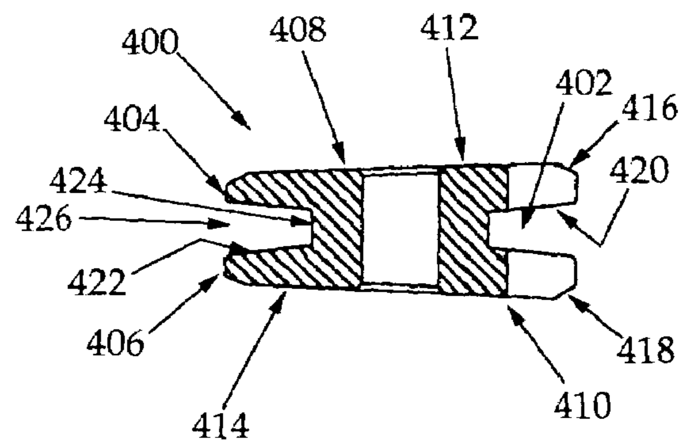
Section A-A
