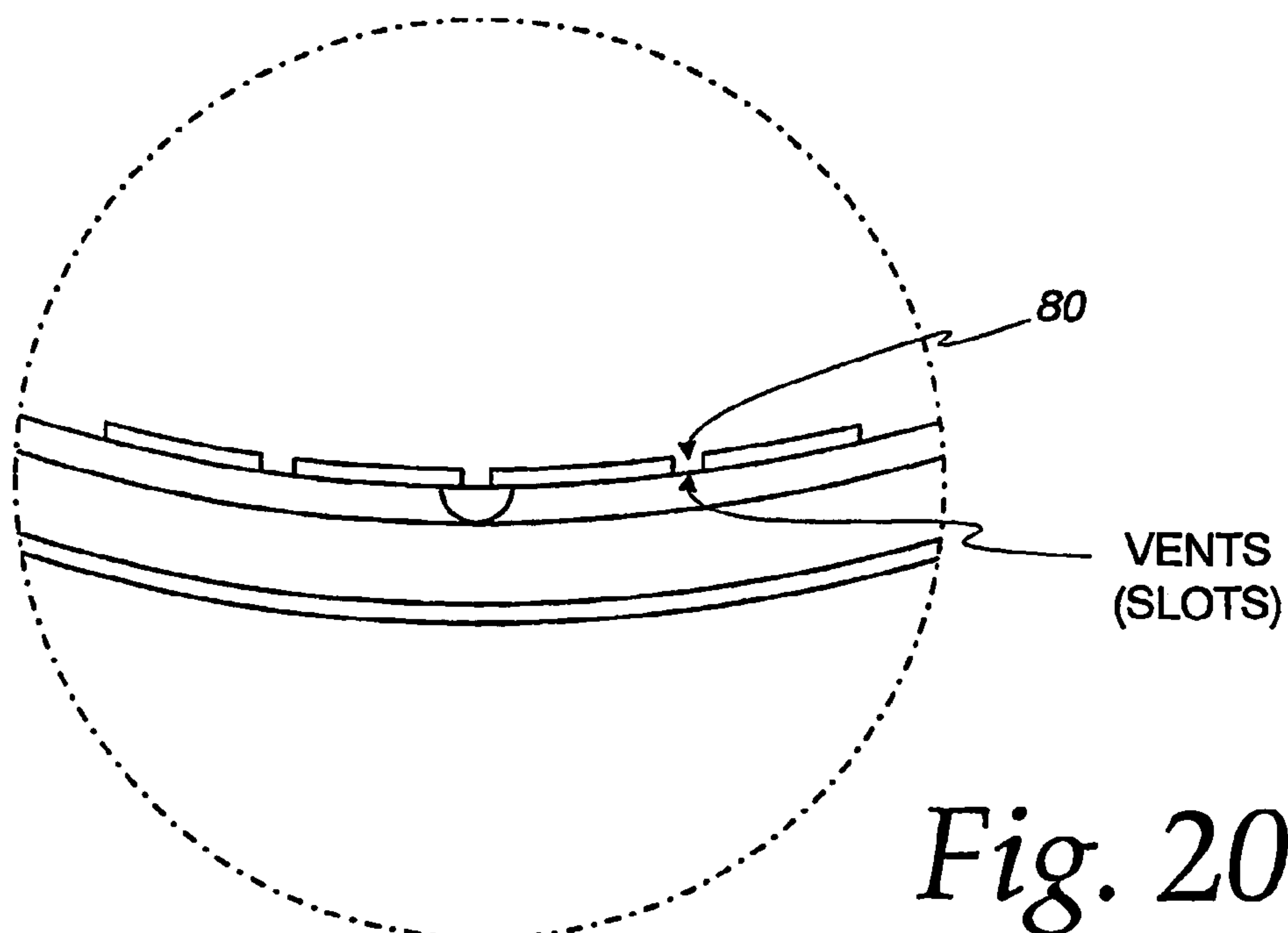
DETAIL Fig. 20
