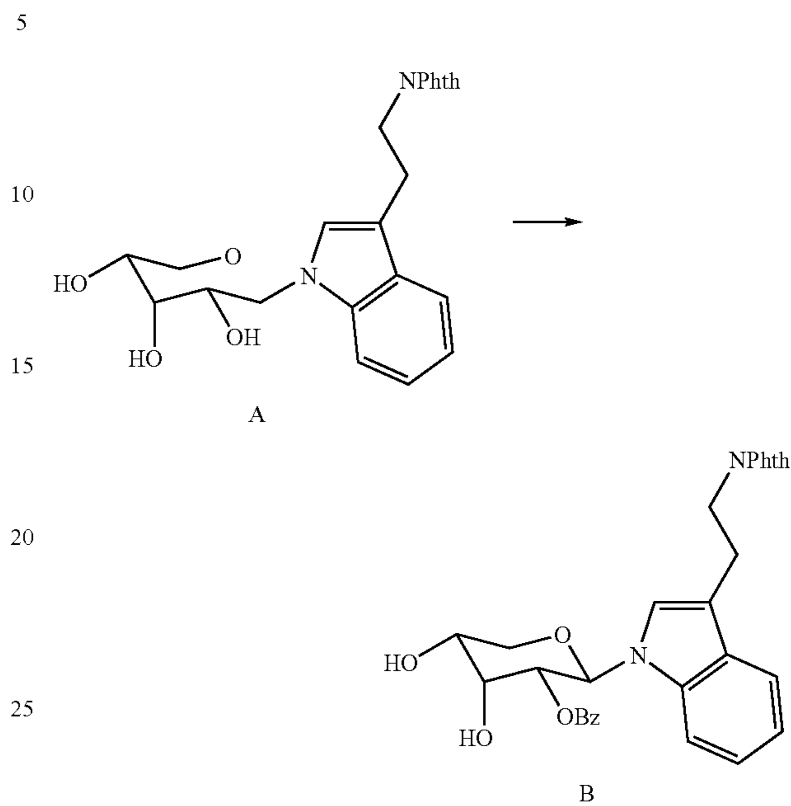
1-(2'-O-Benzoyl-β-D-ribo-pyranosyl)-3-(N-phthaloyl-2-aminoethyl)indole
