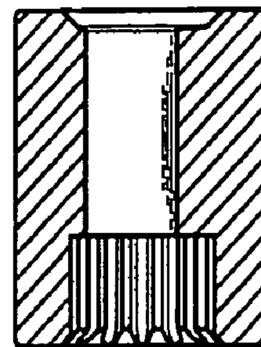
Fig. 7B (Section 7B - 7B)
