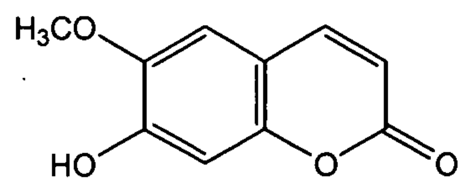
scopoletin (8)
