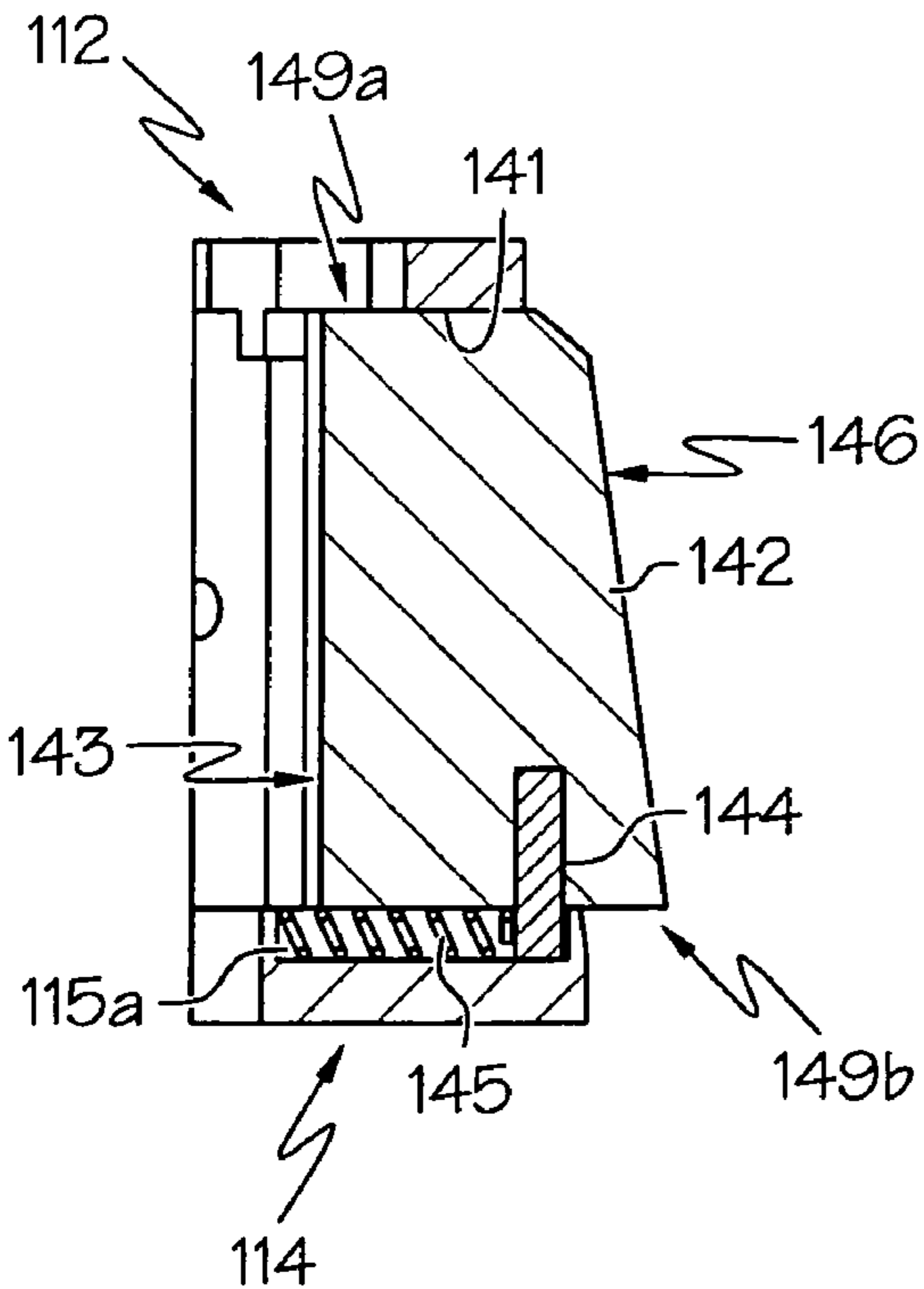
FIG. 3C
