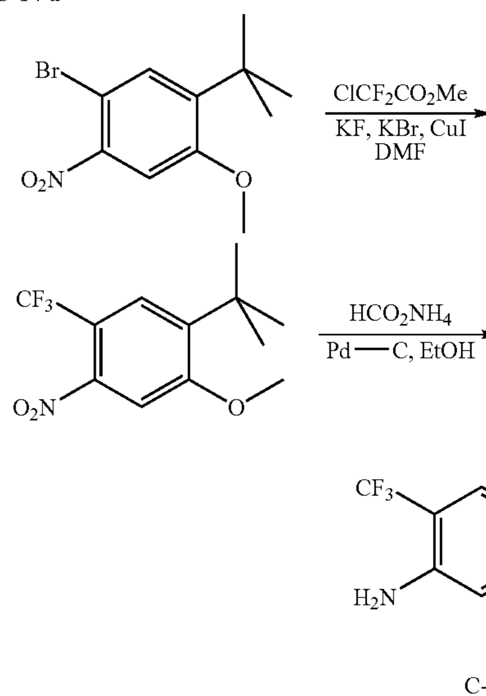
1-tert-Butyl-2-methoxy-5-bromo-4-nitrobenzene
