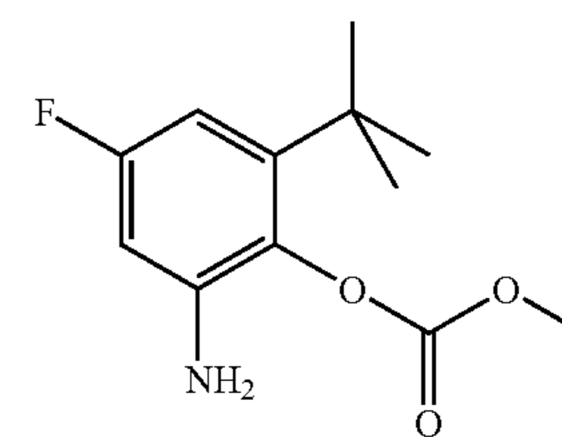
C-6
